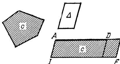
Рис. 2.2с, Приложение с избытком, или гиперболическое приложение.
