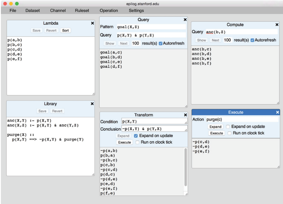
Рис. Б.29. Введено purge(c) и нажата кнопка Expand
