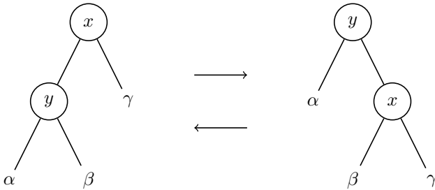
Рис. 3.1. Вращение деревьев поиска
