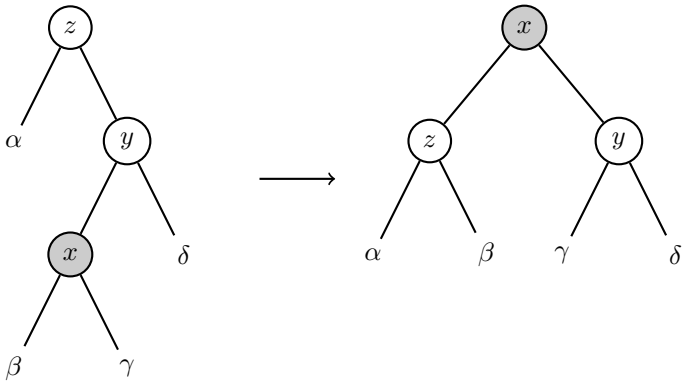
Рис. 3.4. Шаг типа zigzag
