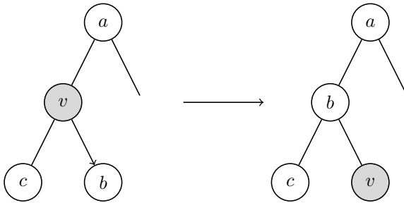
Рис. 4.2. Операция SIFT-Down
