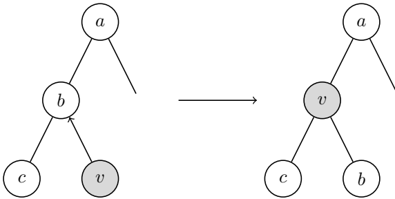
Рис. 4.1. Операция SIFT-UP
