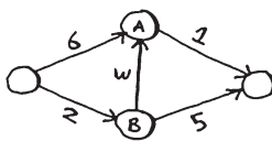
ВЗВЕШЕННЫЙ ГРАФ
