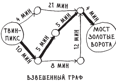
ВЗВЕШЕННЫЙ ГРАФ
