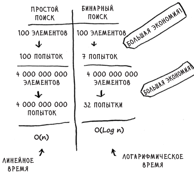
Время выполнения алгоритмов поиска
