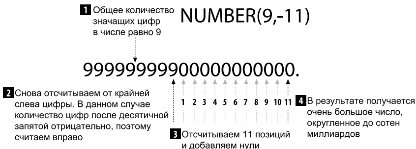
Рис. 9.3. Количество цифр после десятичной запятой задано отрицательным значением
