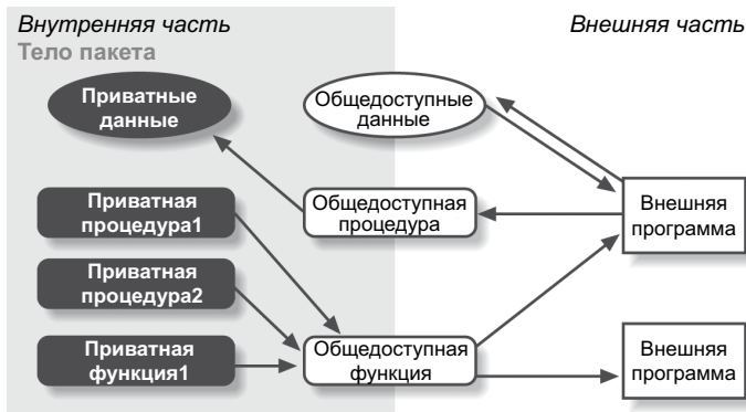
Рис. 18.1. Диаграмма Буча с общедоступными и частными элементами пакета
