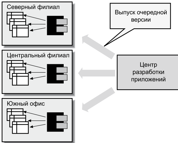
Рис. 24.4. Дублирование кода при использовании модели разрешений создателя
