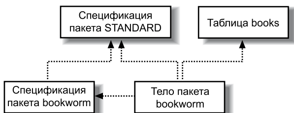
Рис. 20.1. Граф зависимостей пакета bookworm
