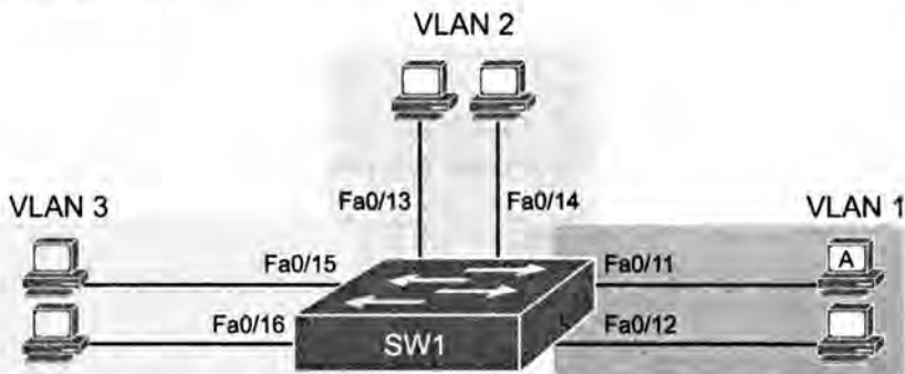
Рис. 1.1. Небольшая локальная сеть Ethernet с сетями VLAN
