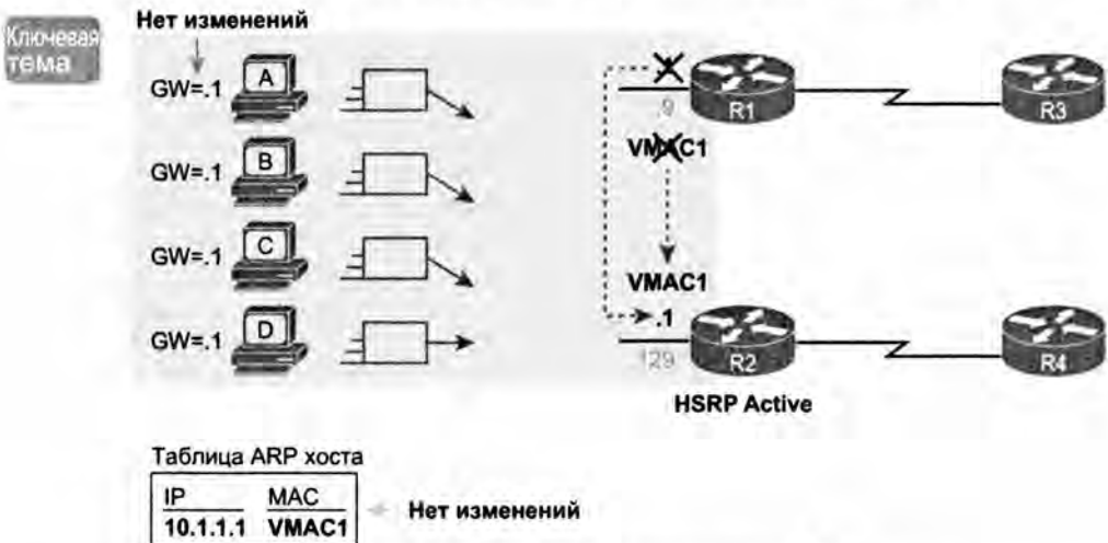
Рис. 6.6. Как только откажет маршрутизатор R1, посланные пакеты пройдут через маршрутизатор R2 (новый активный)
