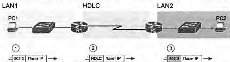
Рис. 12.2. Использование протокола HDLC маршрутизаторами для инкапсуляции пакетов
