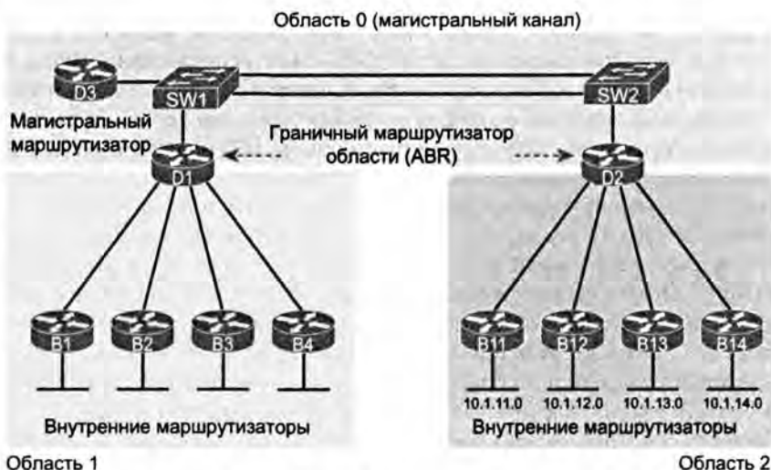
Рис. 8.7. Проект с тремя областями OSPF и маршрутизаторами D1 и D2 в качестве ABR
