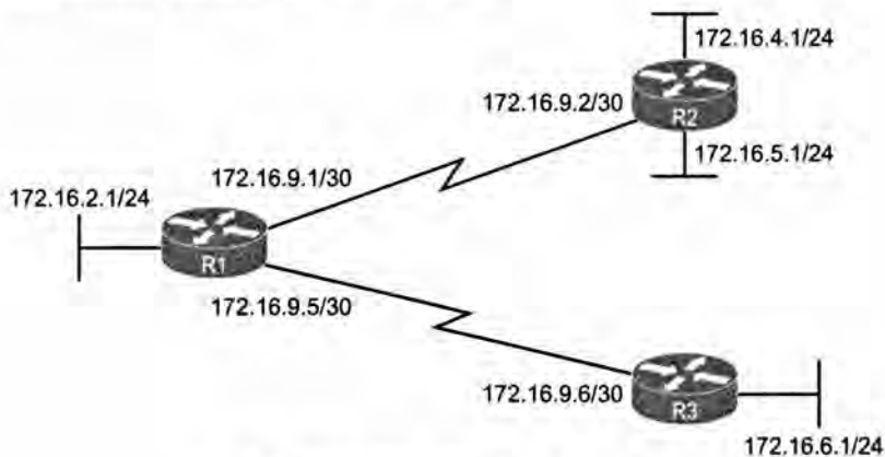
Рис. 11.1. Сеть с шестью подсетями
