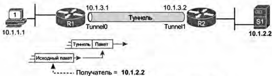
Рис. 7.6. Замена последовательного канала туннелем IP
