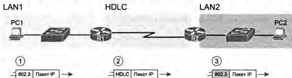
Рис. 12.10. Общая концепция деинкапсуляции и реинкапсуляции пакетов IP маршрутизаторами
