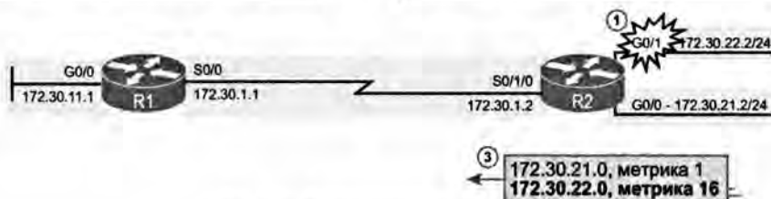
Рис. 9.7. Вытеснение маршрута
