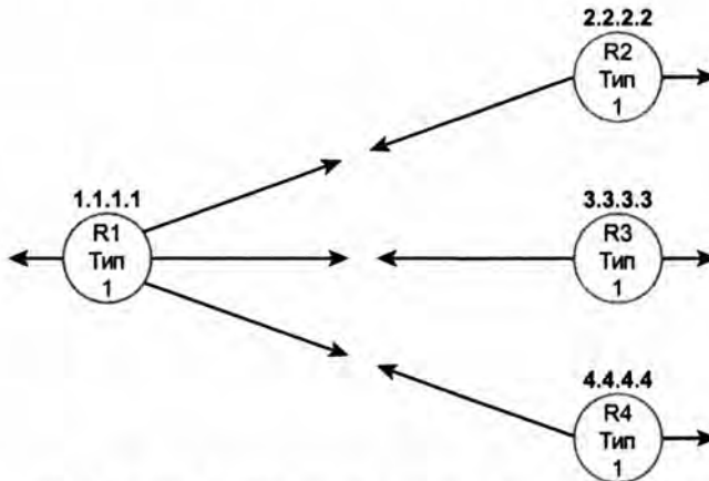
Рис. 8.10. Анонсы LSA типа 1 в проекте одиночной области
