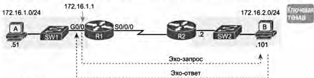
Рис. 4.11. Расширенная команда ping проверяет маршрут к 172.16.1.51
