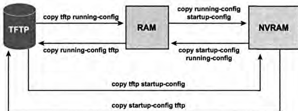
Рис. 20.5. Области и случаи копирования
