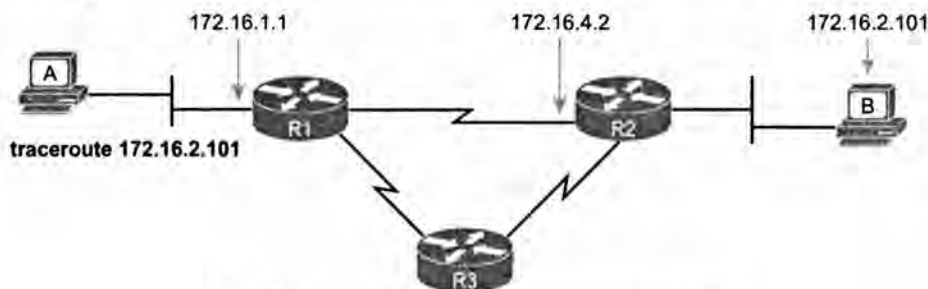
Рис. 4.16. IP-адреса, идентифицированные успехом команды traceroute 172.16.2.101 на хосте A
