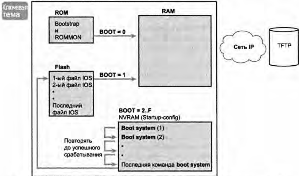
Рис. 20.4. Варианты загрузки операционной системы в современных маршрутизаторах Cisco
