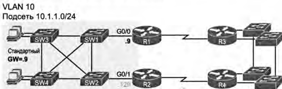
Рис. 6.3. Устранение всех единых точек отказа в проекте сети
