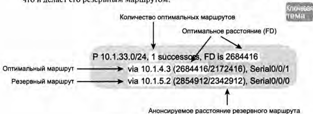
Рис. 10.7. Идентификация резервного маршрута
