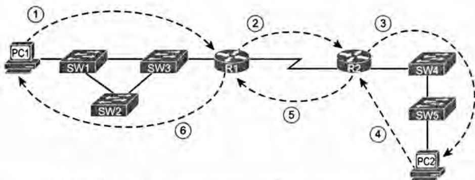
Рис. 3.1. Основные этапы перенаправления IP в рассматриваемом примере
