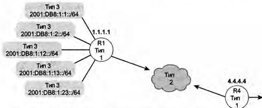
Рис. 17.6. Типы 1, 2 и 3 анонсов LSA, которые должны существовать в области 4
