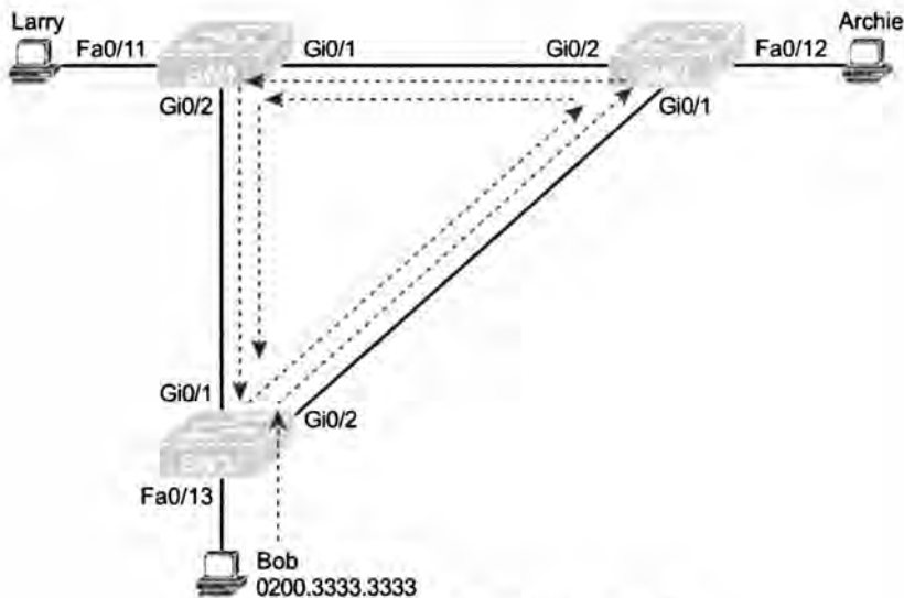
Рис. 1.3. Широковещательный шторм
