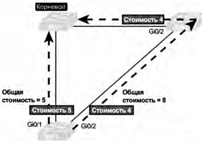
Рис. 1.7. Как человек мог бы вычислить стоимость STP от коммутатора SW3 до корневого коммутатора (SW1)
