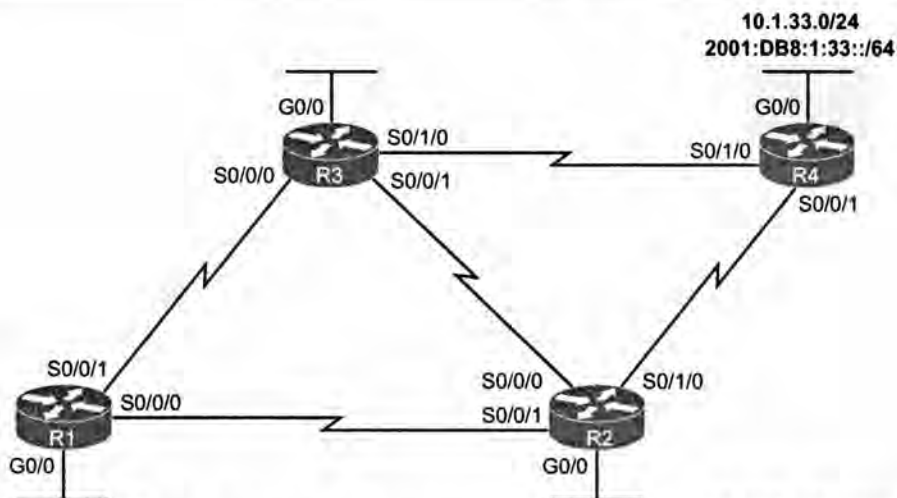
Рис. 18.3. Тот же маршрут через маршрутизатор R4 к подсетям IPv4 33 и IPv6 33
