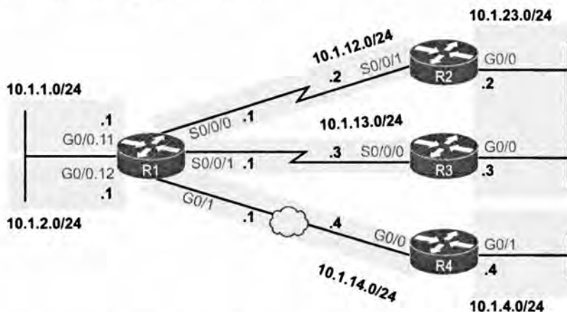
Рис. 8.16. Подсети примера конфигурации OSPF со многими областями
