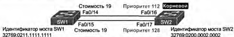
Рис. 2.9. Топология для двух последних схем разрешения конфликтов корневой порты
