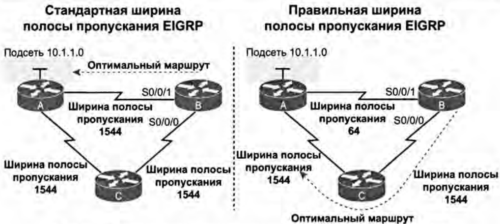
Рис. 9.11. Влияние ширины полосы пропускания на вычисление метрики EIGRP
