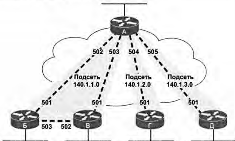
Рис. 14.6. Гибридная сеть: неполносвязная и полносвязная топологии
