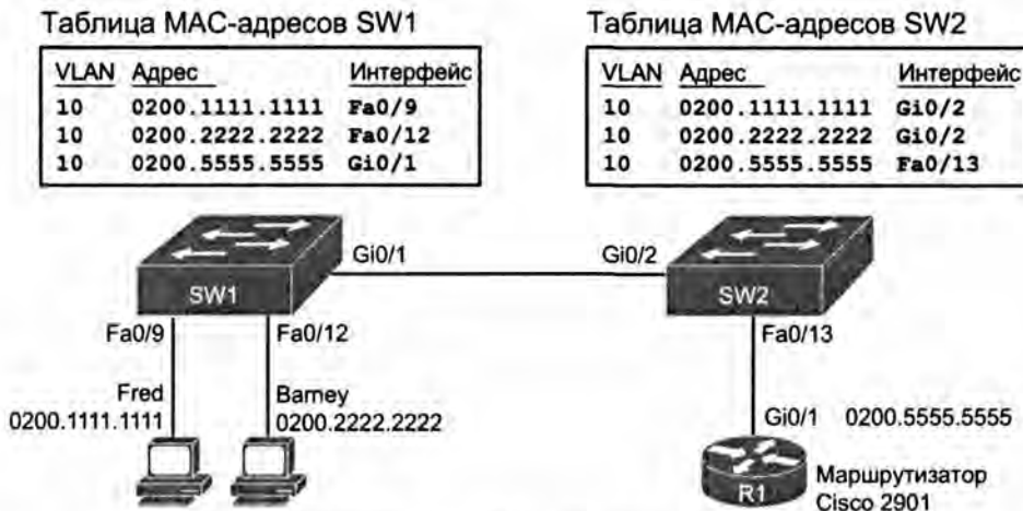
Рис. 1.2. Пример сети LAN с таблицами MAC-адресов
