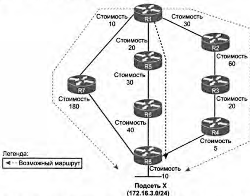
Рис. 8.15. Дерево SPF для выбора маршрута от маршрутизатора R1 к сети 172.16.3.0/24
