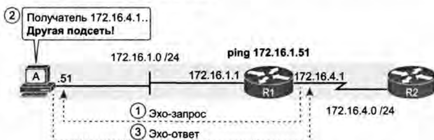
Рис. 4.13. Расширенная команда ping действительно проверяет параметр стандартного маршрутизатора хоста A
