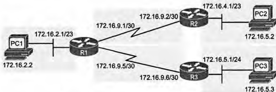
Рис. 5.14. План IP-адресации VLSM в сети 172.16.0.0
