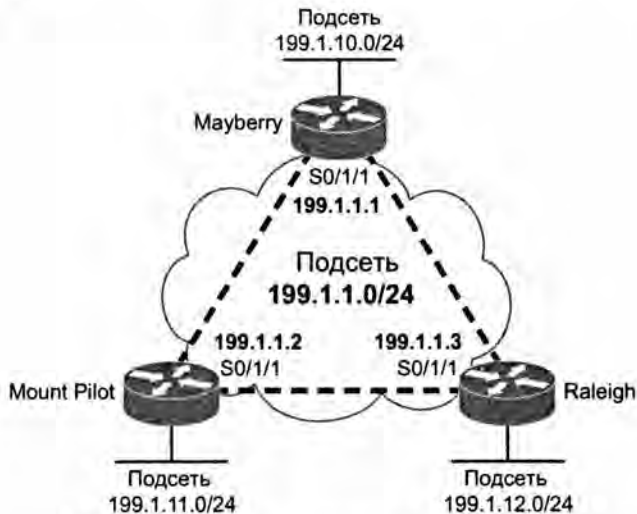
Рис. 14.1. Полносвязная топология с IP-адресами
