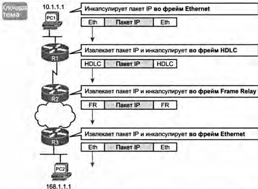
Рис. 4.4. Инкапсуляция и деинкапсуляция пакета при маршрутизации
