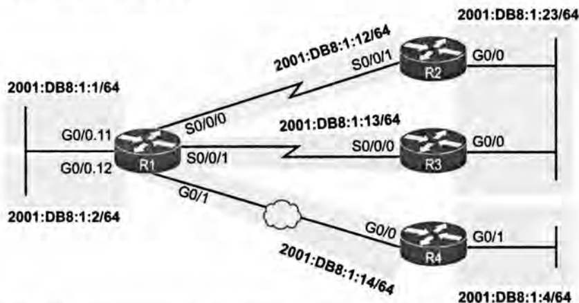
Рис. 17.1. Объединенная сеть для примера многообластной конфигурации OSPFv3
