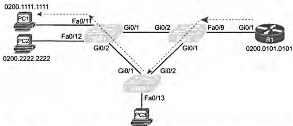
Рис. 3.8. Путь передачи ответа ARP (широковещание) с маршрутизатора R1 на компьютер PC1
