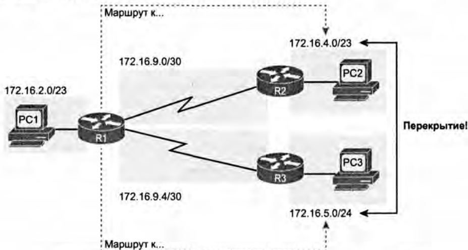
Рис. 5.15. Пример наложения при разных идентификаторах подсети
