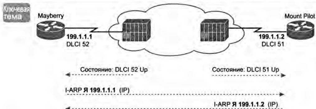
Рис. 14.4. Принцип работы протокола Inverse ARP
