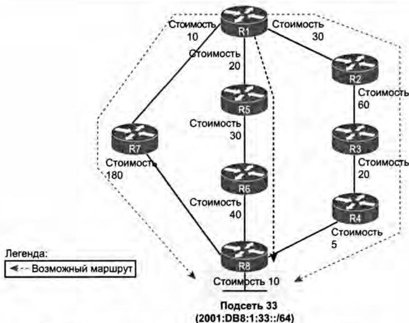
Рис. 17.3. Дерево SPF для поиска маршрута от маршрутизатора R1 к подсети 2001:DB8:1:33::/64
