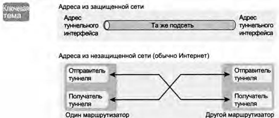
Рис. 7.12. Конфигурация туннеля GRE: отношения между параметрами
