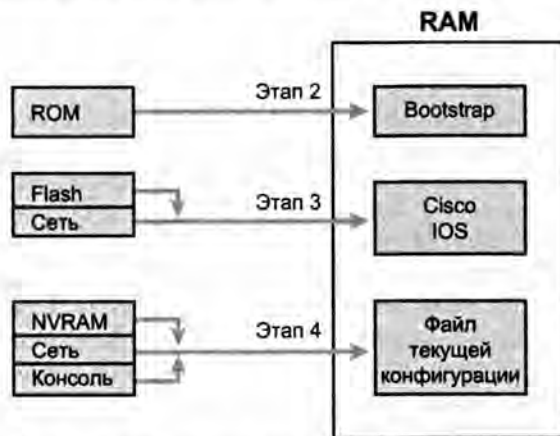
Рис. 20.3. Загрузка программы bootstrap , операционной системы IOS и начальной конфигурации
