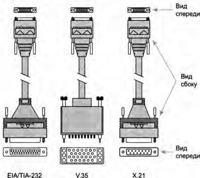
Рис. 12.5. Последовательные кабели, соединяющие модули CSU с маршрутизатором
