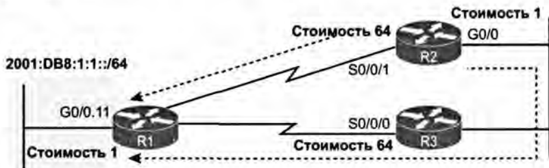
Рис. 17.8. Конкурирующий маршрут через маршрутизатор R2 к подсети 1
