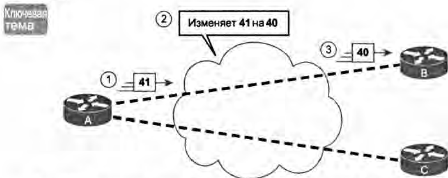
Рис. 13.8. Перенаправление Frame Relay от маршрутизатора А к маршрутизатору В
