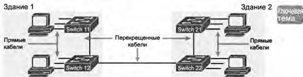
Рис. 3.4. Пример использования перекрестных кабелей и кабелей с прямыми соединениями
