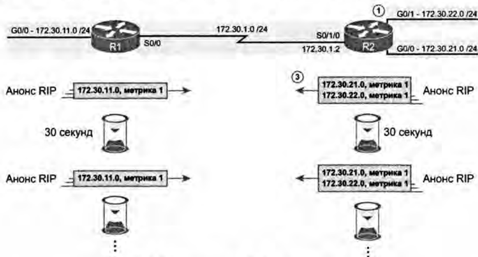
Рис. 9.5. Работа протокола RIP в нормальных условиях: полное обновление маршрутов с разделенным диапазоном
