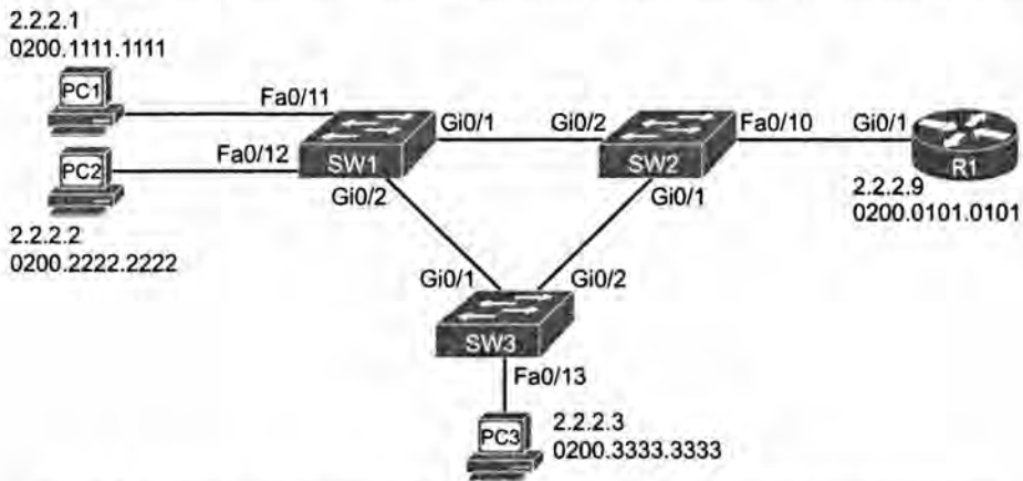
Рис. 3.5. Исходная схема сети первого примера поиска и устранения неисправностей
