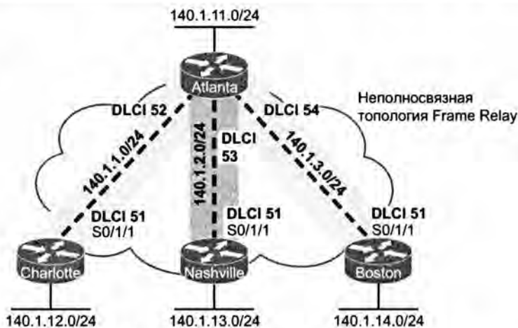
Рис. 13.12. IP-адреса в неполносвязной топологии
