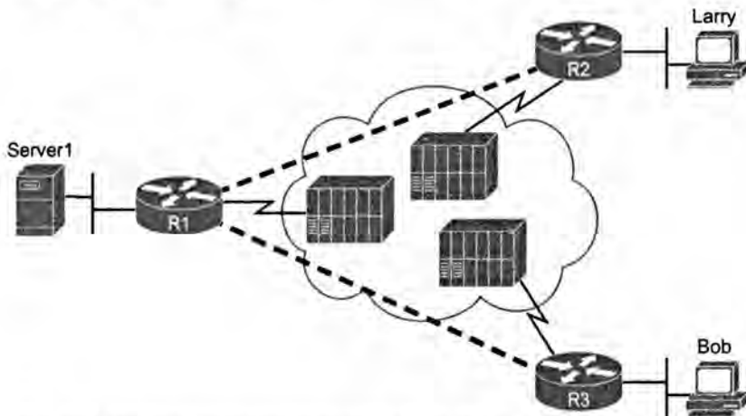
Рис. 13.4. Типичная неполносвязная сеть Frame Relay, соединяющая три хоста
