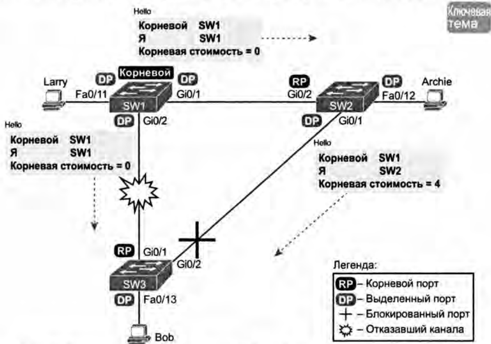
Рис. 1.9. Начальное состояние топологии STP перед отказом канала связи SW1–SW3
