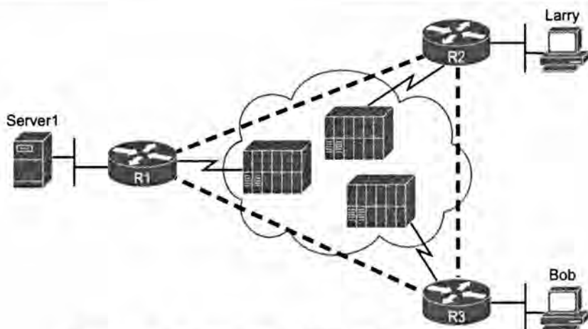
Рис. 13.3. Типичная сеть Frame Relay, соединяющая три хоста
