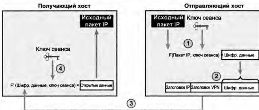
Рис. 7.3. Основные этапы процесса шифрования IPsec
