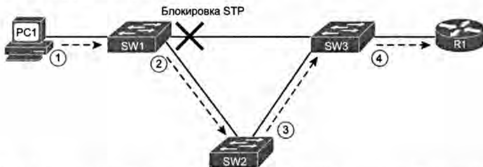
Рис. 3.2. Основные этапы в примере пересылки данных в процессе коммутации локальной сети
