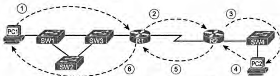
Рис. 4.1. Основные этапы маршрутизации IP
