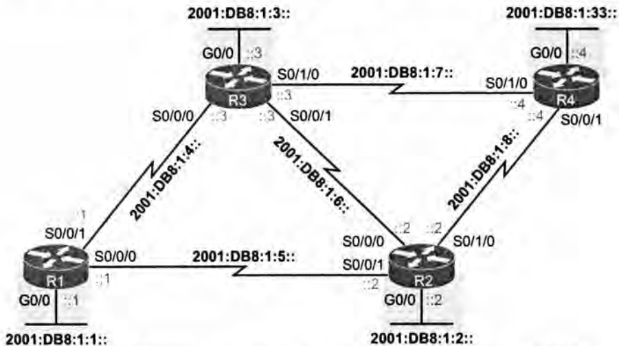
Рис. 18.2. Объединенная сеть примера многообластной конфигурации EIGRPv6
