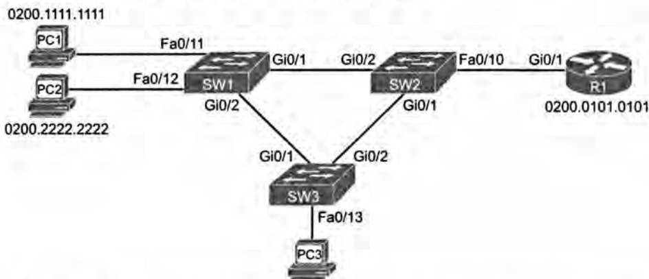
Рис. 3.3. Коммутируемая сеть, используемая в ходе анализа уровня данных в этой главе
