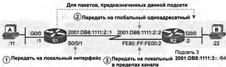
Рис. 16.9. Три возможности статических маршрутов в конфигурации IPv6
