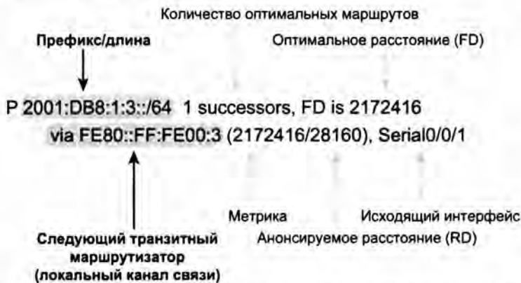
Рис. 18.5. Сравнение подробностей IPv6 с общими элементами топологических данных EIGRP
