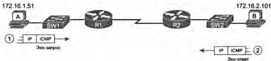
Рис. 4.6. Концепция, лежащая в основе команды ping 172.16.2.101 на хосте А
