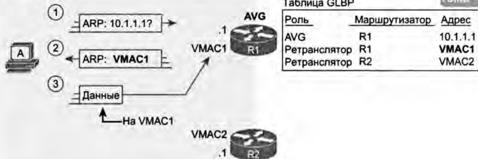
Рис. 6.8. Протокол GLBP настраивает хост А, возвращая сообщение ARP Reply с адресом VMAC1 маршрутизатора R1
