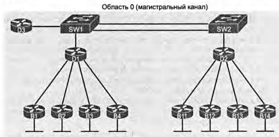
Рис. 8.6. Одиночная область OSPF
