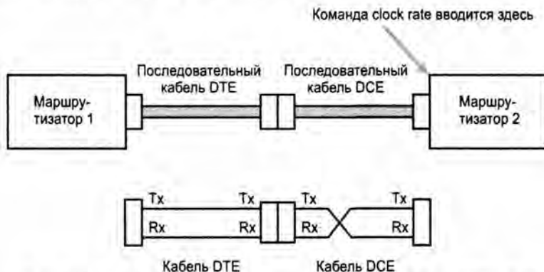
Рис. 12.8. Последовательное соединение использует кабели DTE и DCE
