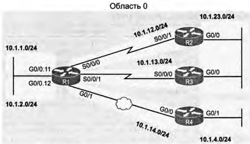
Рис. 8.9. Корпоративная сеть с семью подсетями IPv4
