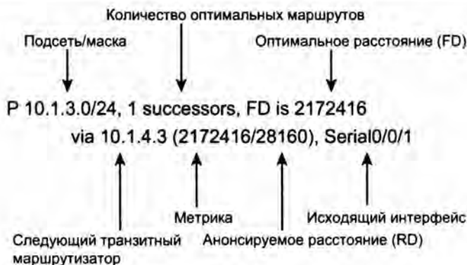
Рис. 10.4. Поля в выводе команды show ip eigrp topology
