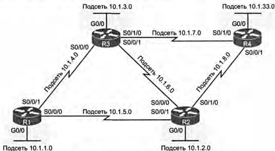
Рис. 10.3. Расширенная объединенная сеть
