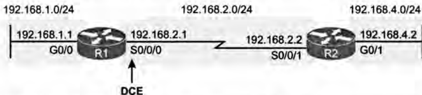
Рис. 12.11. Типичный последовательный канал между двумя маршрутизаторами
