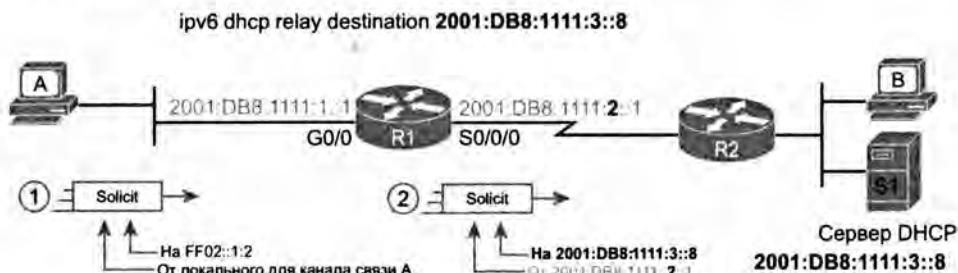
Рис. 16.6. Агент пересылки DHCPv6 и IPv6-адреса DHCP
