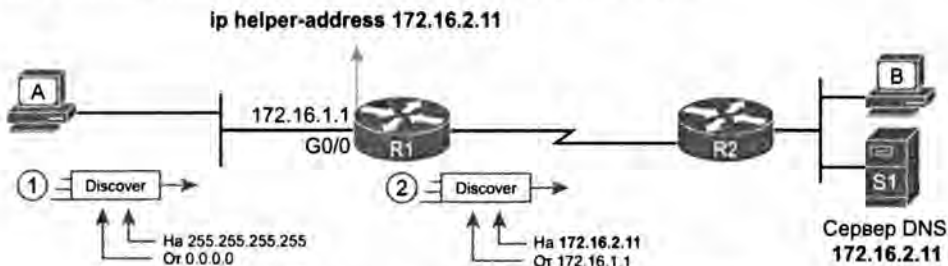
Рис. 5.9. Действие команды ip helper-address
