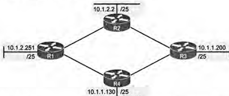
Рис. 5.12. IP-адреса интерфейсов LAN с единой маской (/25) в сети 10.0.0.0
