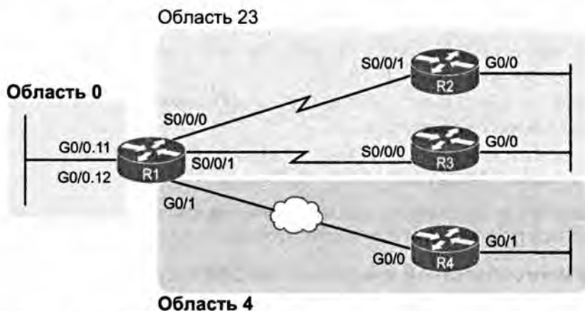
Рис. 8.17. Проект областей примера конфигурации OSPF со многими областями
