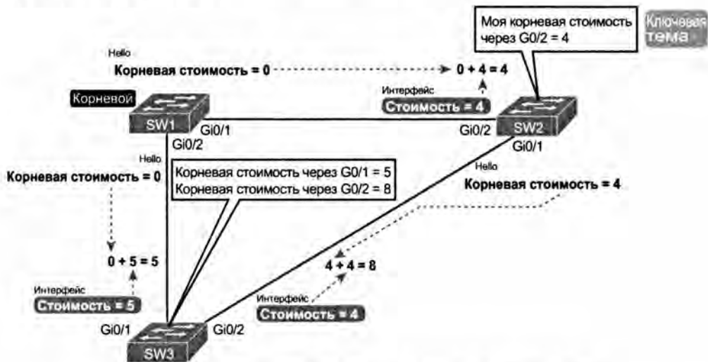
Рис. 1.8. Так протокол STP фактически вычисляет стоимость от коммутатора SW3 до корневого коммутатора (SW1)
