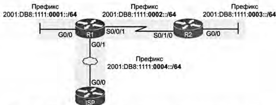
Рис. 16.2. Проект подсети с глобальным префиксом маршрутизации 2001:0DB8:1111
