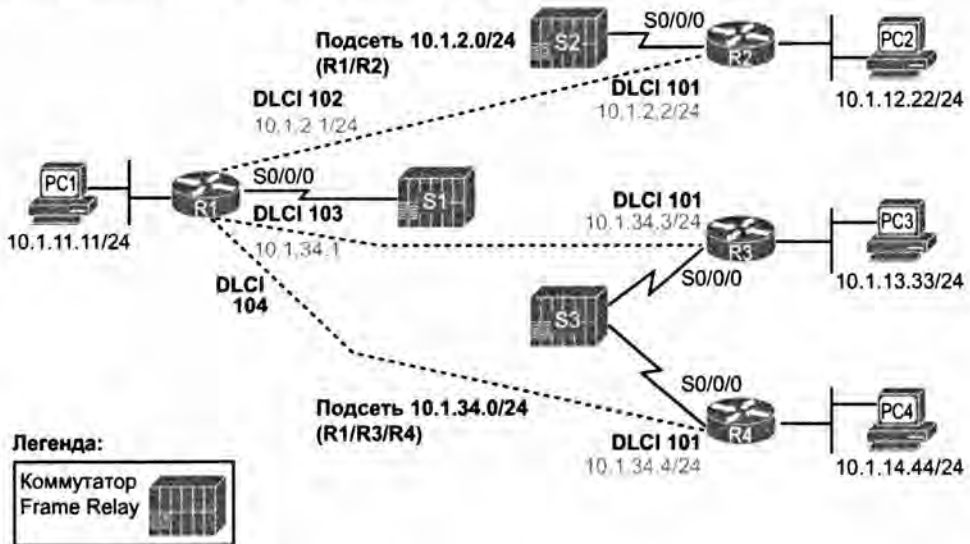
Рис. 14.7. Пример сети протокола Frame Relay для иллюстрации процесса поиска ошибок
