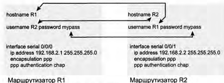
Рис. 12.15. Конфигурация CHAP
