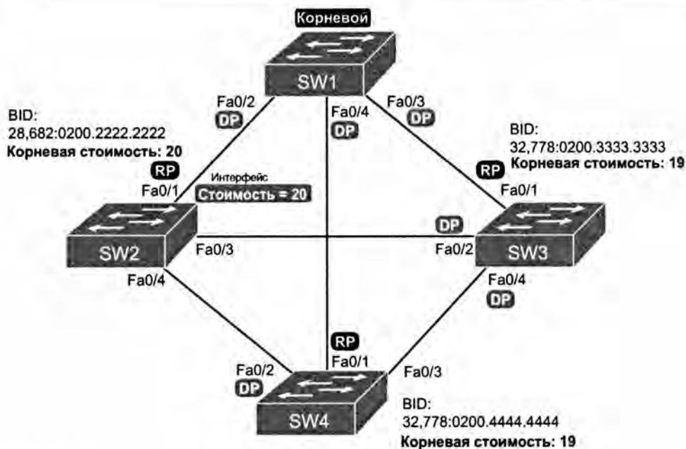
Рис. 2.10. Выборы выделенного порта
