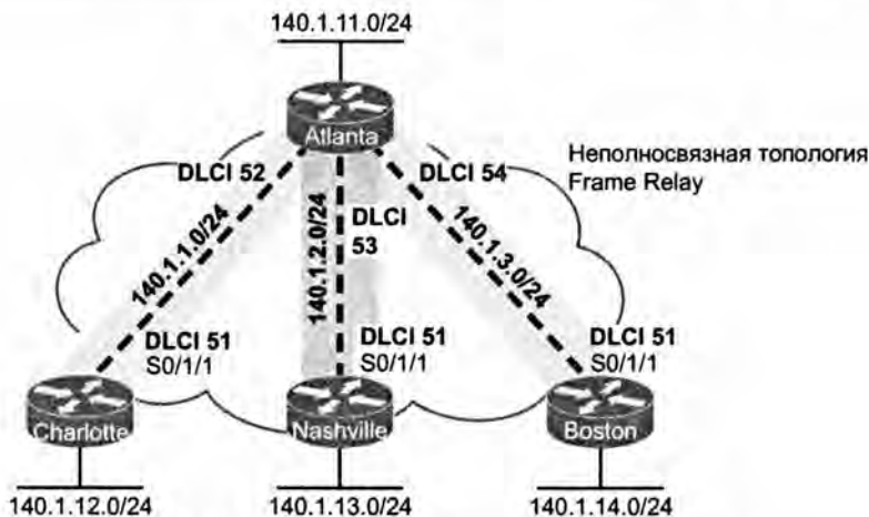
Рис. 14.5. Неполносвязная топология с IP-адресами и глобальными идентификаторами DLCI
