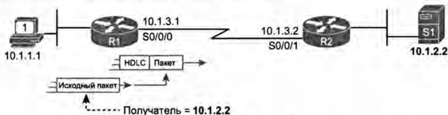
Рис. 7.5. Маршрутизация пакета IP по последовательному каналу
