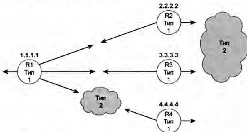
Рис. 8.11. Анонсы LSA типа 1 и 2 в области 0 проекта одиночной области
