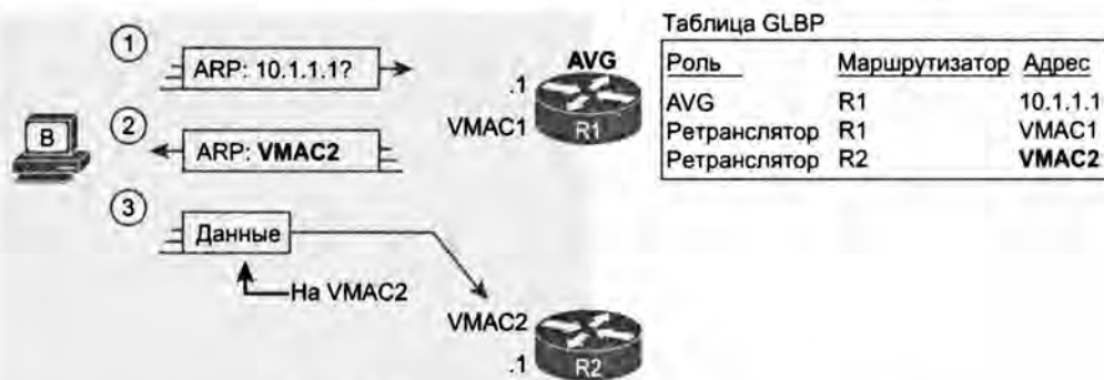
Рис. 6.9. Протокол GLBP настраивает хост В, возвращая сообщение ARP Reply с адресом VMAC2 маршрутизатора R2
