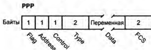
Рис. 12.12. Формат фрейма PPP
