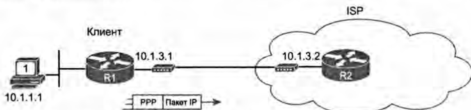
Рис. 15.12. Передача фреймов PPP между маршрутизаторами по соединению dial-up с провайдером ISP
