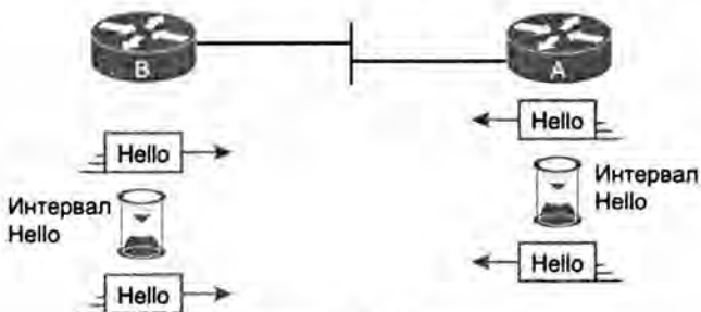
Рис. 9.8. Пакеты Hello протокола EIGRP
