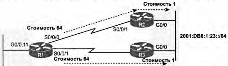
Рис. 17.7. Два маршрута с равными метриками от маршрутизатора R1 к подсети 2001:DB8:1:23::/64
