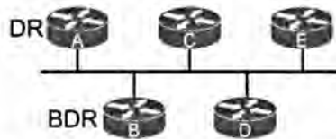
Рис. 8.4. Маршрутизаторы A и B выбраны маршрутизаторами DR и BDR соответственно
