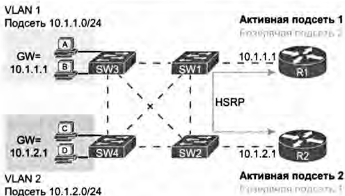
Рис. 6.7. Балансировка нагрузки протоколом HSRP при использовании разных активных маршрутизаторов в подсетях
