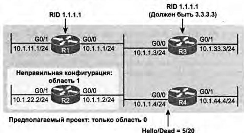
Рис. 11.6. Проблемы, препятствующие соседским отношениям OSPF в сети LAN
