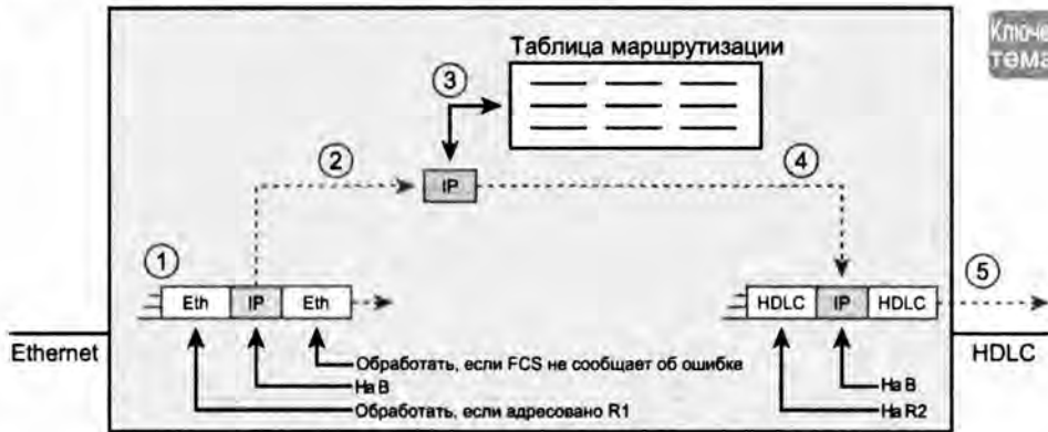
Рис. 4.3. Логика перенаправления маршрутизатора
