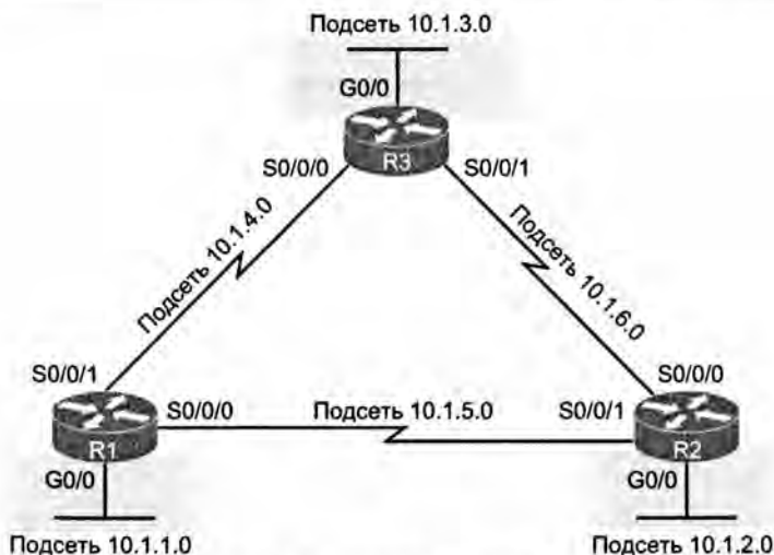
Рис. 10.1. Схема сети для примеров настройки протокола EIGRP
