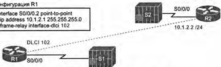
Рис. 14.8. Сведения о конфигурации, относящиеся к неудачной команде ping 10.1.2.2 маршрутизатора R1
