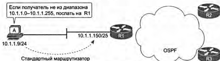
Рис. 5.3. Разные результаты вычисления подсети на хосте и в сети
