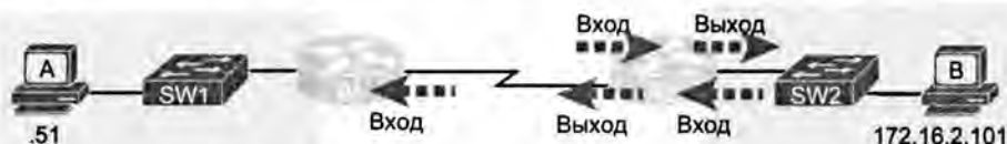
Рис. 4.9. Области, где списки ACL могут отфильтровать сообщения команды ping
