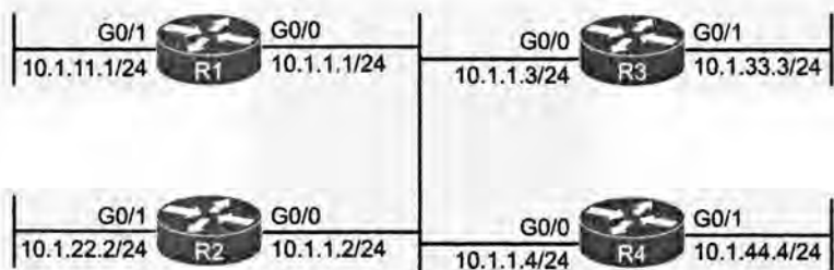
Рис. 11.3. Схема сети для иллюстрации команд процесса поиска и устранения неисправностей в протоколах EIGRP и OSPF
