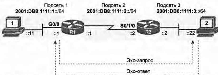
Рис. 16.12. Адреса отправителя и получателя расширенной команды ping в примере 16.5
