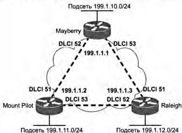
Рис. 14.2. Полносвязная топология с показанными глобальными идентификаторами DLCI
