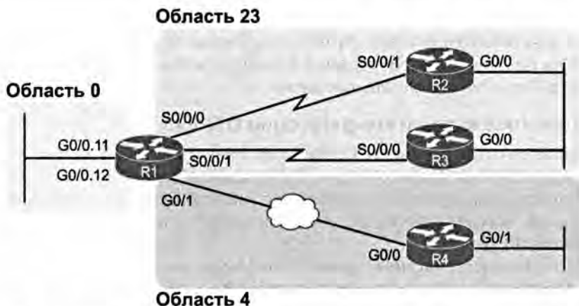
Рис. 17.2. Проект областей примера многообластной конфигурации OSPFv3
