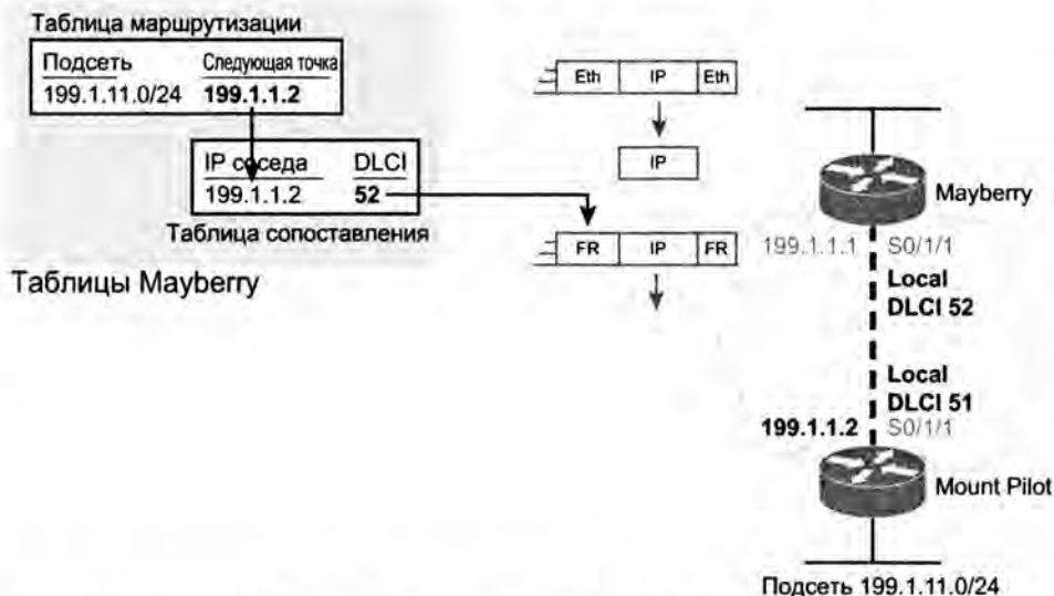
Рис. 14.3. Логика выбора правильного идентификатора DLCI на маршрутизаторе Mayberry
