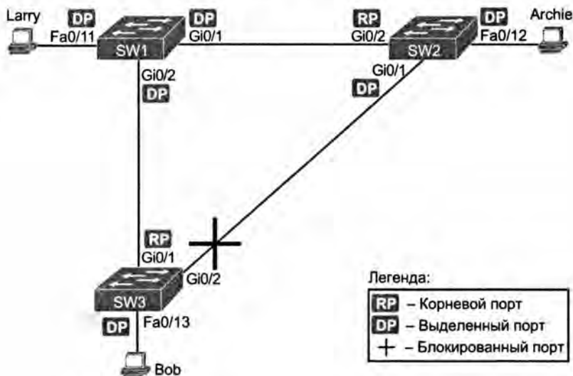
Рис. 2.4. Сеть LAN для примеров настройки и проверки STP
