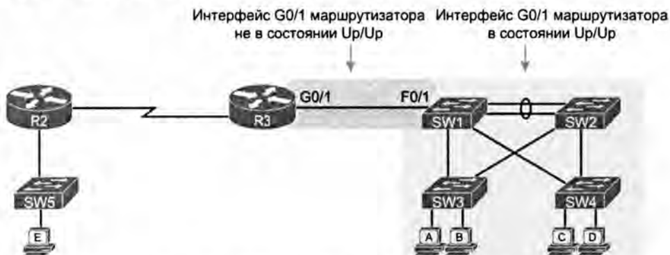
Рис. 5.10. Где искать проблемы на основании состояния интерфейса LAN маршрутизатора
