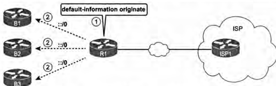
Рис. 17.4. Использование протокола OSPFv3 для анонсирования стандартного маршрута
