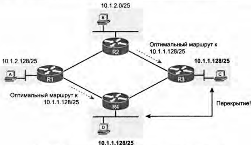
Рис. 5.13. Идентификаторы подсети, вычисленные по рис. 5.12
