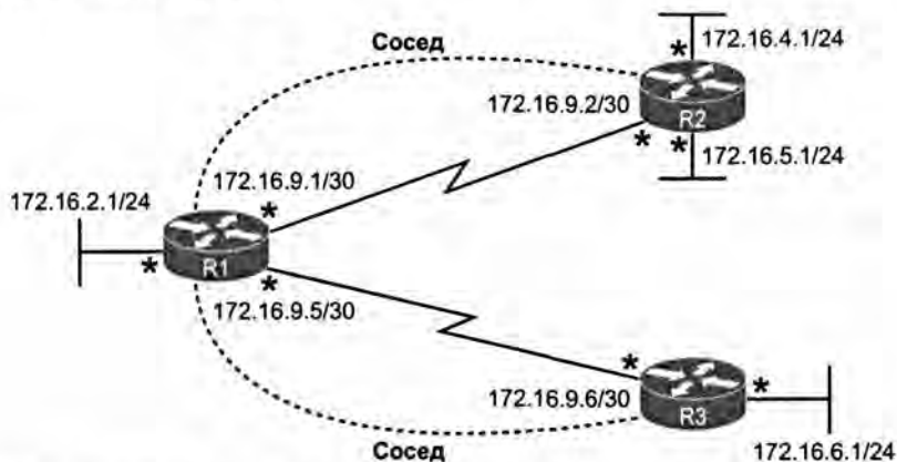
Рис. 11.2. Интерфейсы, на которых разрешен протокол маршрутизации, и соседские отношения
