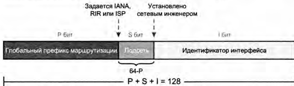
Рис. 16.1. Структура глобального одноадресного IPv6-адреса в подсети
