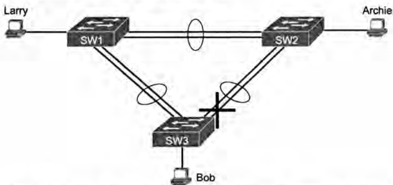
Рис. 1.10. Каналы EtherChannel с двумя сегментами между коммутаторами
