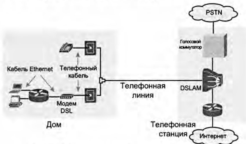
Рис. 15.9. Кабели и устройства домашнего канала связи DSL
