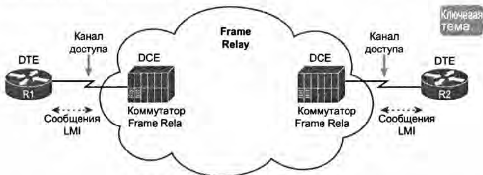
Рис. 13.1. Компоненты сети Frame Relay
