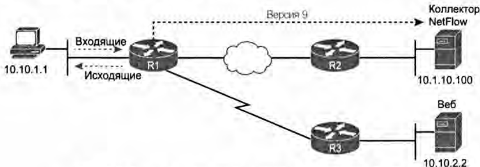
Рис. 19.7. Сеть, используемая для примера конфигурации NetFlow
