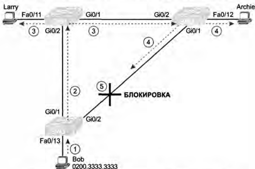
Рис. 1.4. Протокол STP блокирует порт, чтобы разорвать круг
