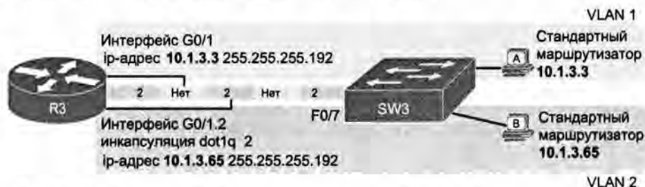
Рис. 5.8. Конфигурация IP-адреса маршрутизатора с ROAS и собственная сеть VLAN 1
