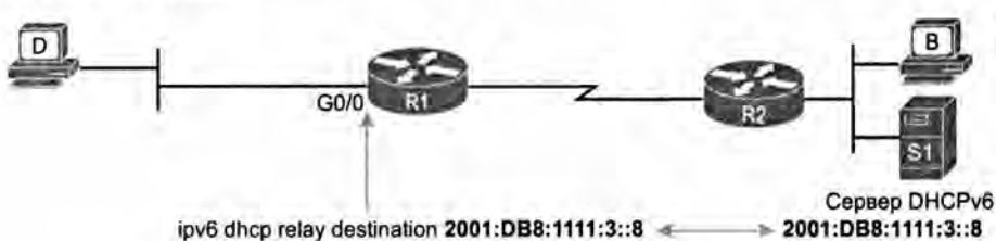
Рис. 16.16. Ретранслятор DHCP IPv6
