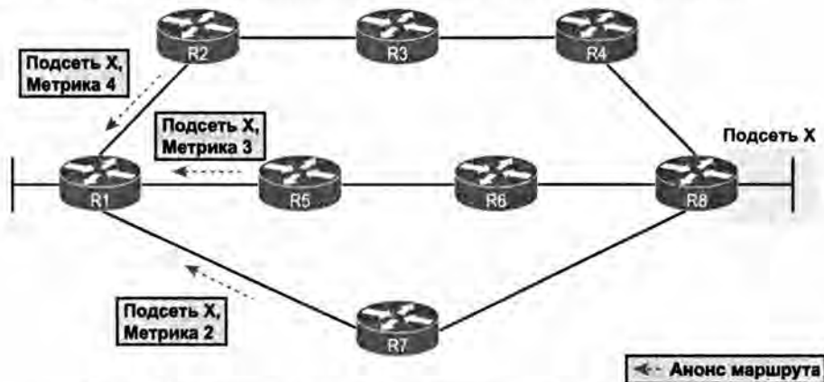
Рис. 9.3. Информация, изученная по дистанционно-векторному протоколу
