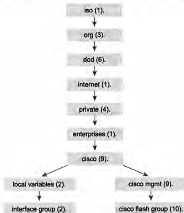
Рис. 19.4. База управляющей информации (MIB)
