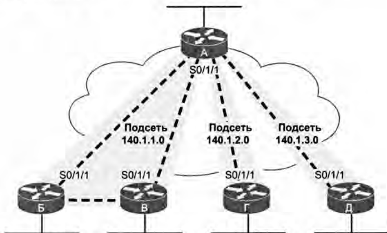
Рис. 13.13. Гибрид полносвязной и неполносвязной топологий
