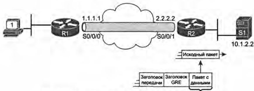
Рис. 7.11. Маршрутизаторы Интернета перенаправляют пакет IP GRE на основании открытых IP-адресов
