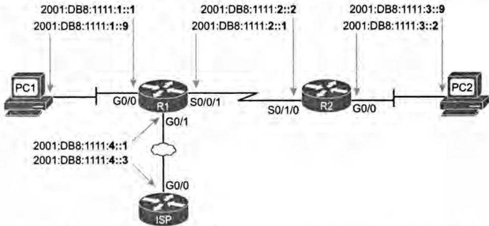
Рис. 16.3. Пример статических IPv6-адресов на основании проекта подсети на рис. 16.2
