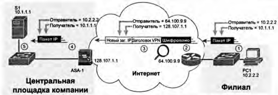
Рис. 7.1. Концепция туннеля VPN между площадками в Интранете
