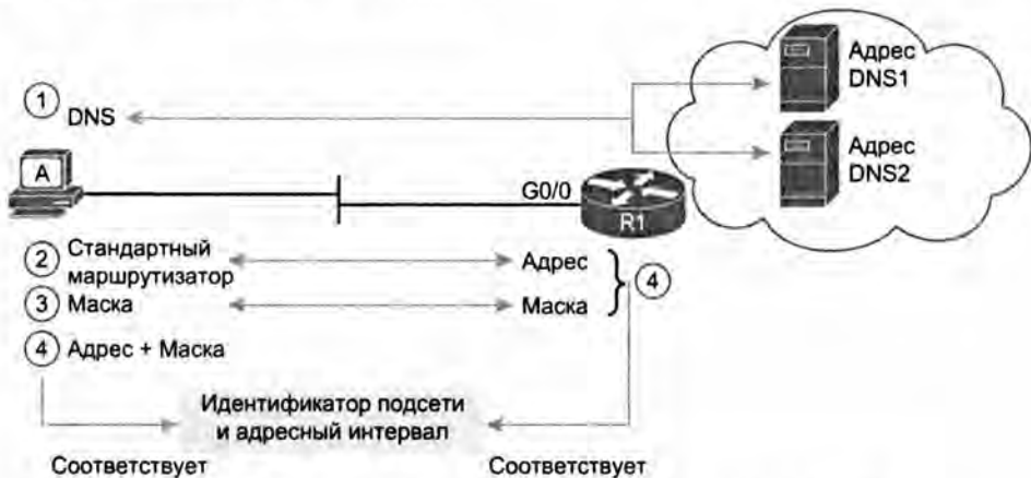
Рис. 5.2. Сравнение параметров IPv4 хоста с используемыми в сети
