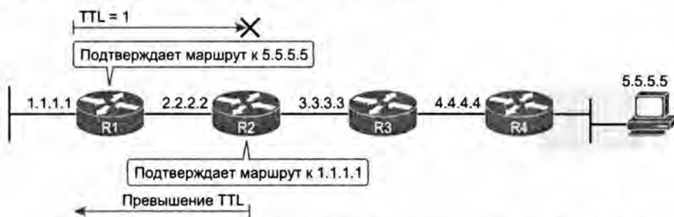
Рис. 4.19. Сообщения, позволяющие команде traceroute вывести адрес 2.2.2.2
