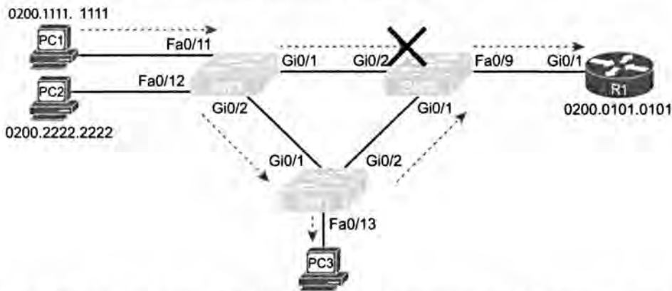
Рис. 3.7. Путь передачи запроса ARP (широковещание) с компьютера PC1 на маршрутизатор R1
