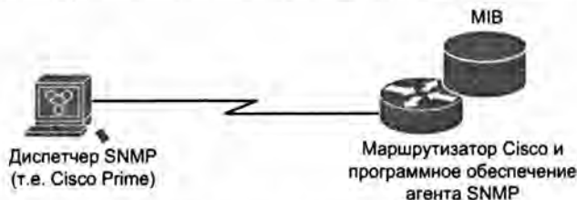
Рис. 19.1. Элементы простого протокола управления сетью
