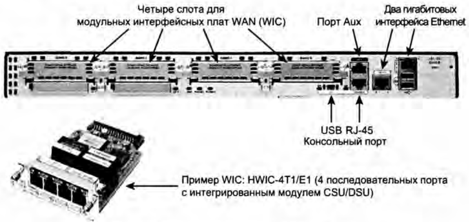
Рис. 12.6. Маршрутизатор с набором плат WIC, обладающих интегрированными модулями CSU/DSU и портами RJ-48
