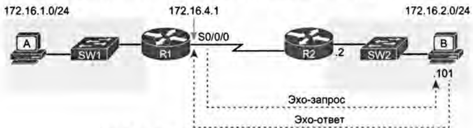
Рис. 4.7. Стандартно команда ping 172.6.2.101 использует IP-адрес исходящего интерфейса
