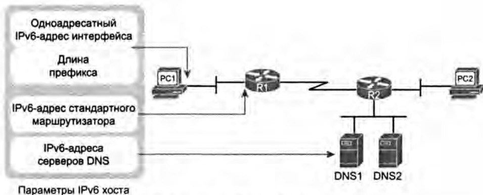
Рис. 16.10. Параметры IPv6, необходимые на хостах
