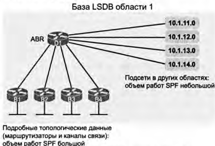
Рис. 8.8. Концепция баз LSDB меньшей области 1
