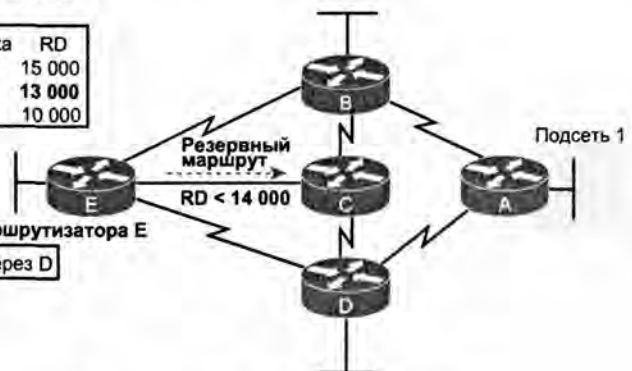
Рис. 9.14. Маршрут через маршрутизатор C является резервным
