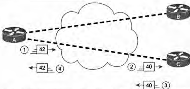
Рис. 13.10. Перенаправление Frame Relay между маршрутизаторами А и С
