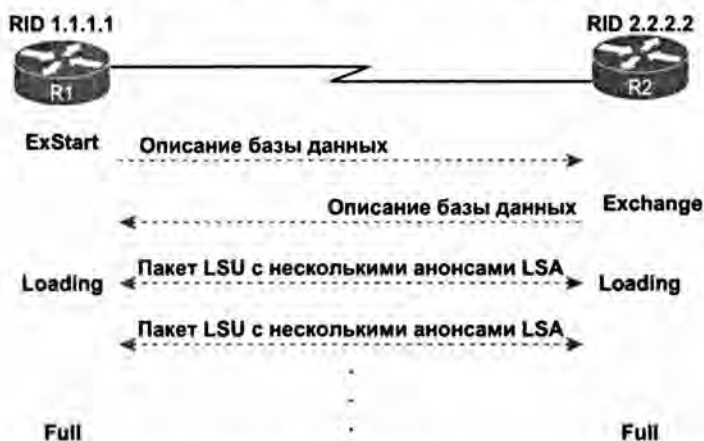
Рис. 8.3. Пример обмена базами данных, завершающийся состоянием полной синхронизации
