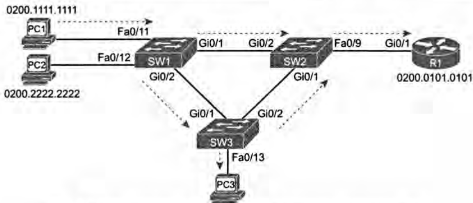
Рис. 3.6. Сеть для второго примера поиска и устранения неисправностей
