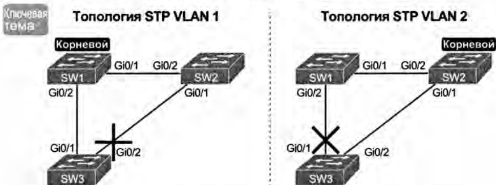
Рис. 2.2. Балансировка нагрузки при помощи протокола PVST+
