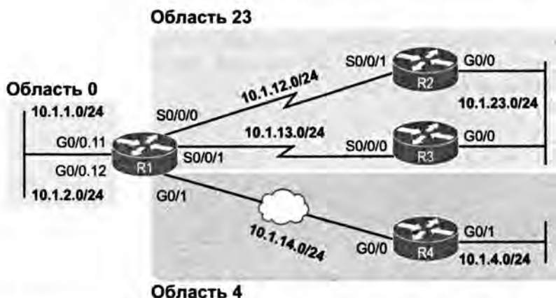
Рис. 8.12. Проект с многими областями той же объединенной сети, что и на рис. 8.9
