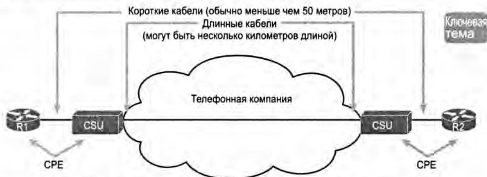
Рис. 12.4. Двухточечная выделенная линия: компоненты и терминология
