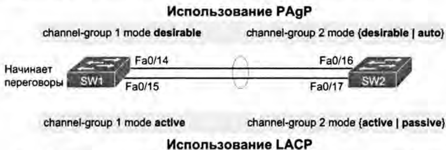
Рис. 2.7. Правильные комбинации параметров в конфигурации канала EtherChannel
