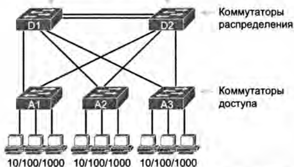
Рис. 2.1. Типичный выбор конфигурации: корневым стоит сделать коммутатор распределения
