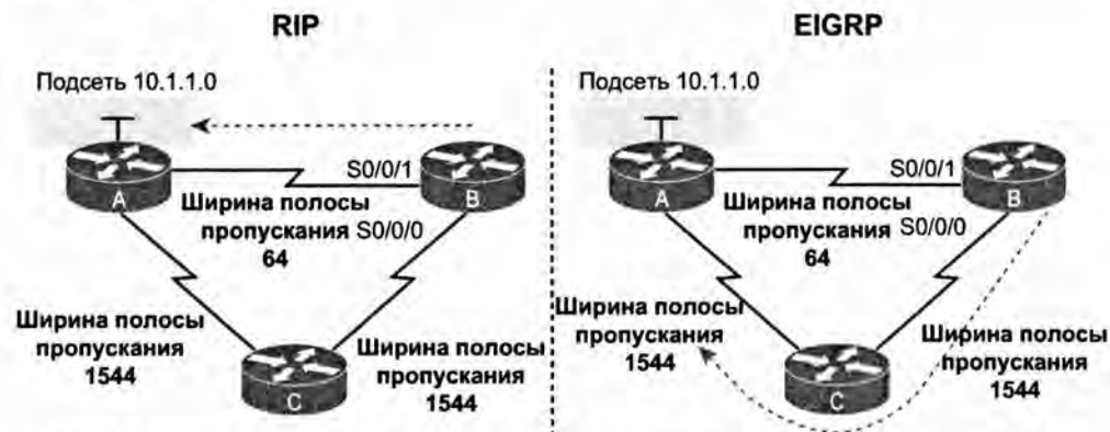
Рис. 9.2. Протокол EIGRP выбирает более длинный, но лучший маршрут к подсети 10.1.1.0
