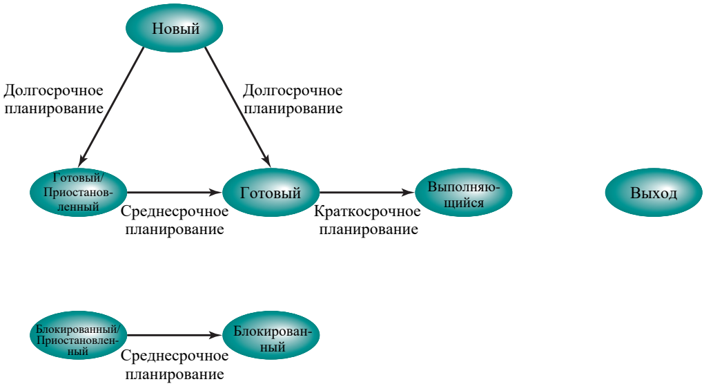
Рис. 9.1. Место планирования в диаграмме переходов состояний процесса
