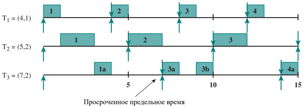
Рис. 10.8. Пример работы RMS
