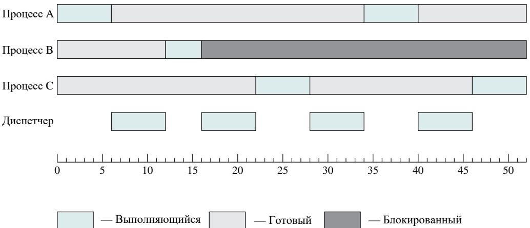
Рис. 3.7. Состояния процессов из рис. 3.4
