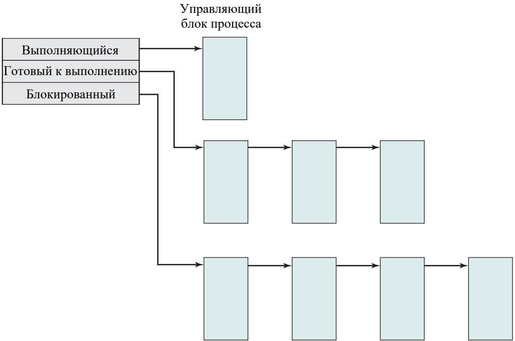
Рис. 3.14. Структура списков процессов
