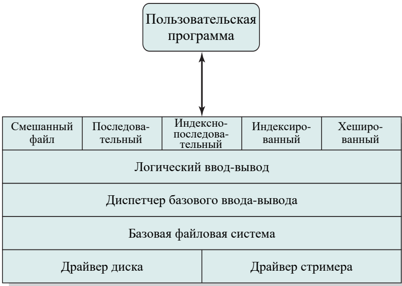
Рис. 12.1. Архитектура программного обеспечения файловой системы [95]
