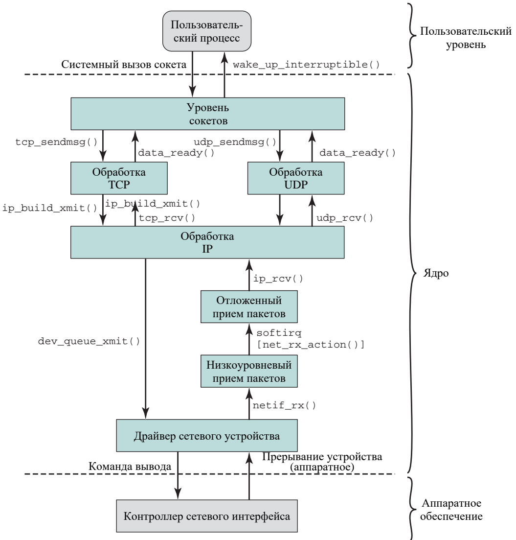
Рис. 17.7. Компоненты ядра Linux для обработки данных по протоколам TCP/IP
