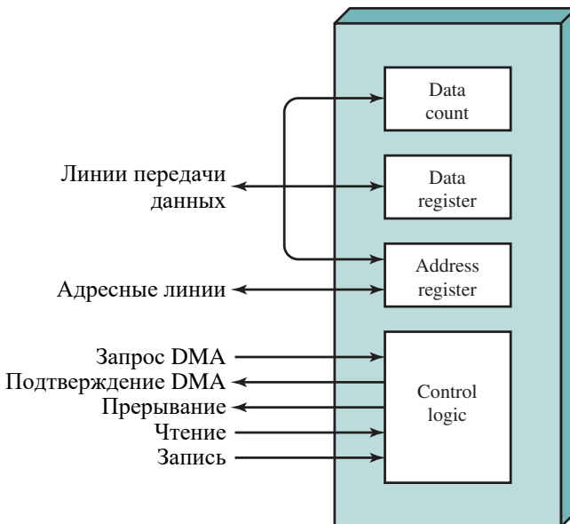
Рис. 11.2. Блок-схема прямого доступа к памяти
