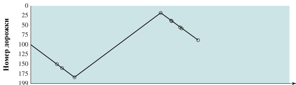
Рис. 11.7. Сравнение алгоритмов дискового планирования (см. табл. 11.2)
