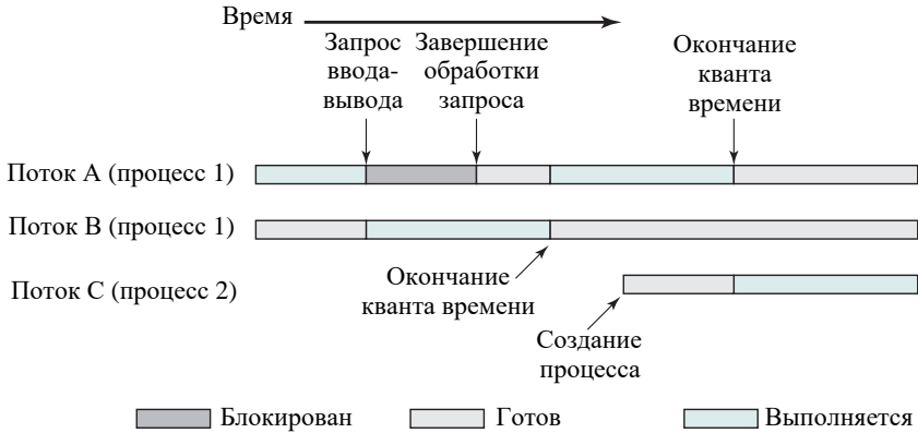
Рис. 4.4. Пример многопоточности в однопроцессорной системе
