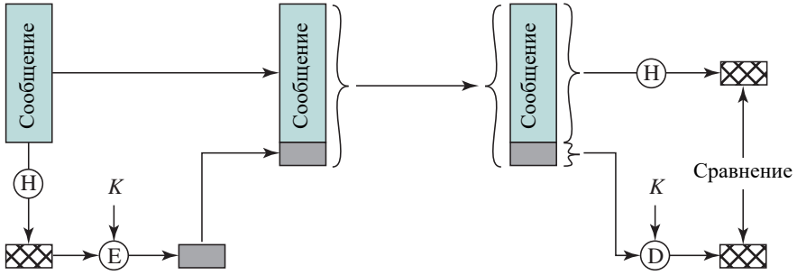
а) Использование симметричного шифрования
