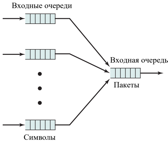
Рис. 21.10. Модель системы массового обслуживания для модуля сборки и разборки пакетов (PAD)
