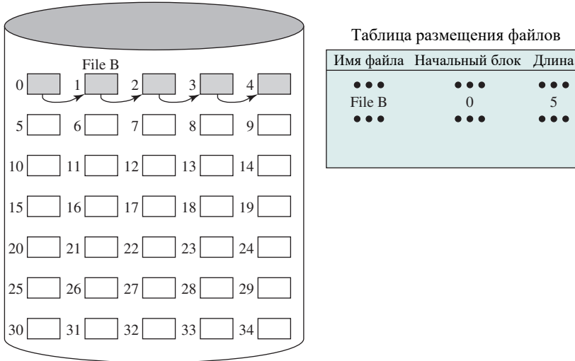
Рис. 12.12. Цепочечное размещение файлов (после уплотнения)
