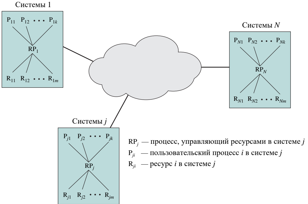
Рис. 19.7. Модель для решения задачи взаимного исключения при управлении распределенными процессами
