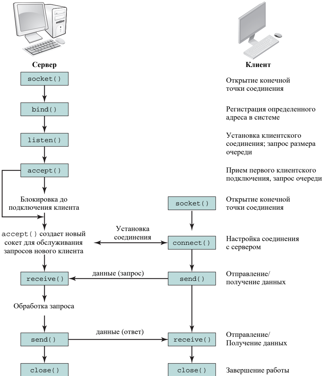
Рис. 17.6. Системные вызовы сокетов для ориентированного на соединения протокола
