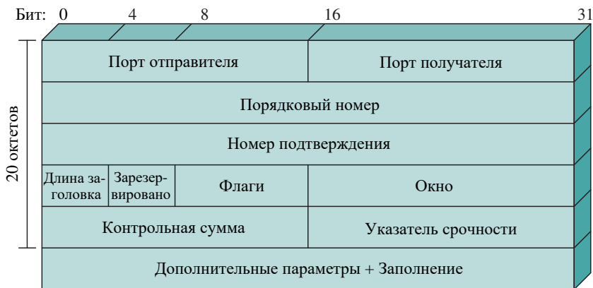
а) Заголовок пакета TCP
