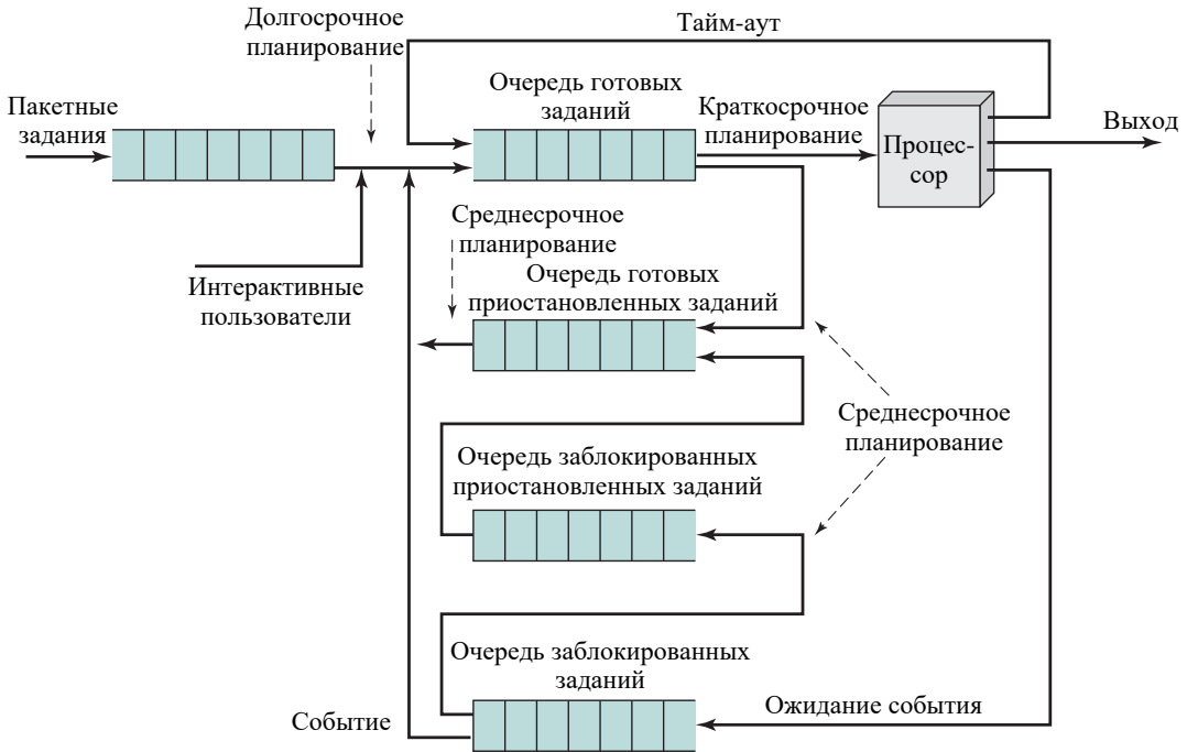
9.3 Диаграмма планирования с участием очередей
