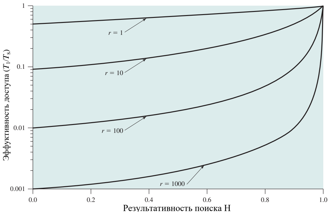
Рис. 1.23. Эффективность доступа в зависимости от результативности поиска
