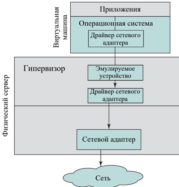
Рис. 14.8. Ввод-вывод в виртуальной среде
