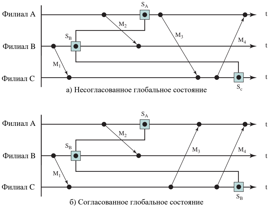
Рис. 19.4. Несогласованные и согласованные глобальные состояния
