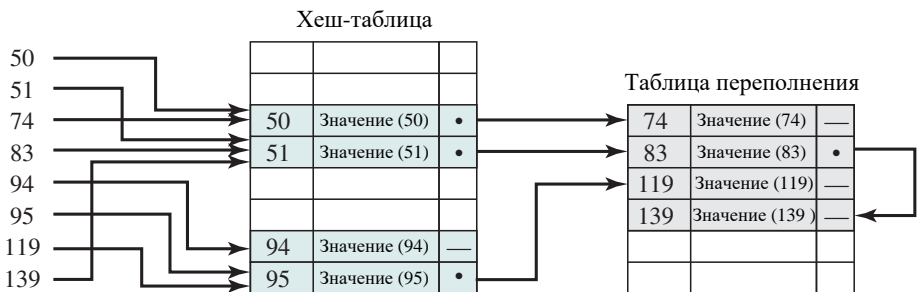
б) Переполнение с цепочками
