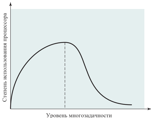
Рис. 8.19. Влияние уровня многозадачности на степень использования процессора
