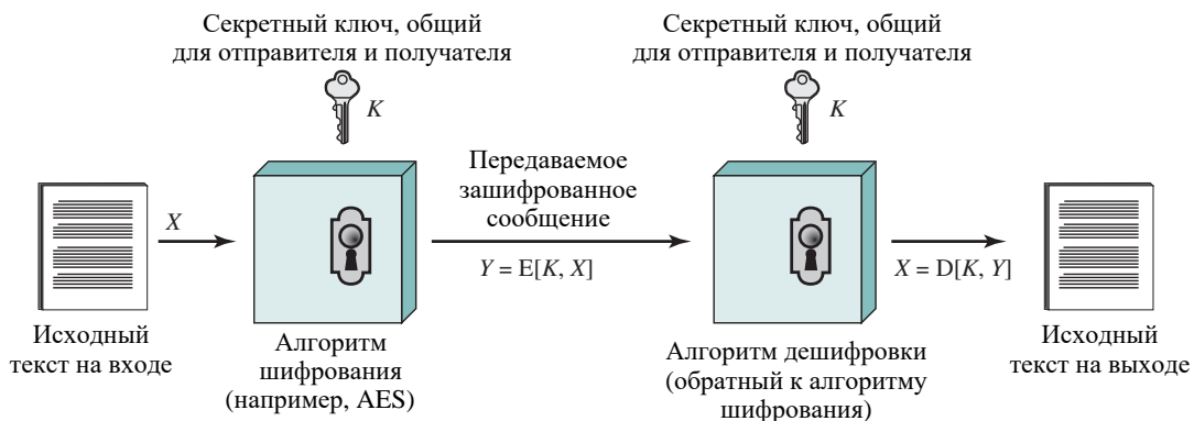
Рис. Л.1. Упрощенная модель симметричного шифрования
