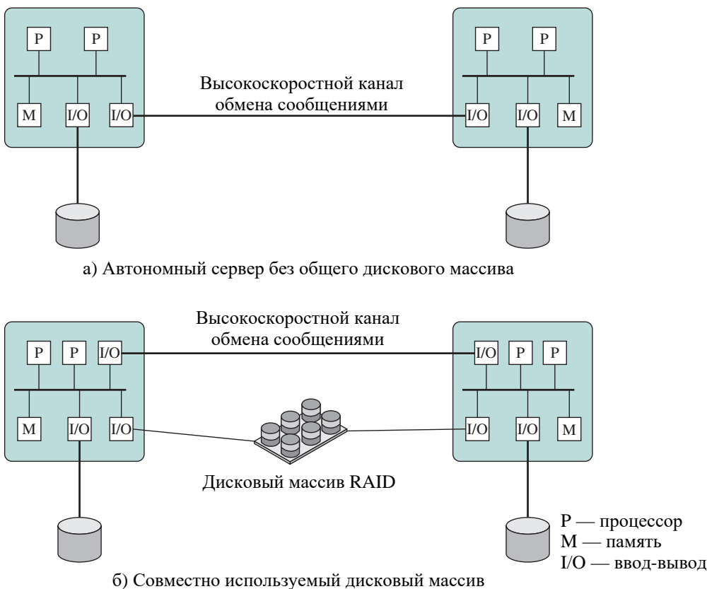
Рис. 18.13. Конфигурации кластеров
