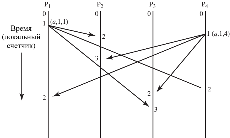
Рис. 19.9. Еще один пример операции по алгоритму присваивания отметки времени
