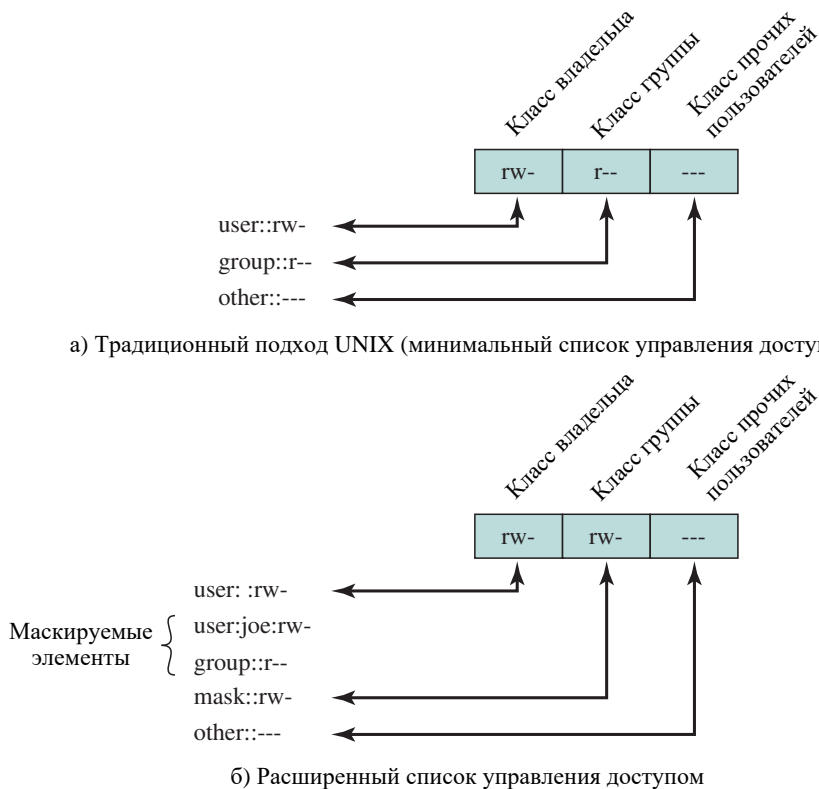
Рис. 15.8. Управление доступом к файлам в UNIX
