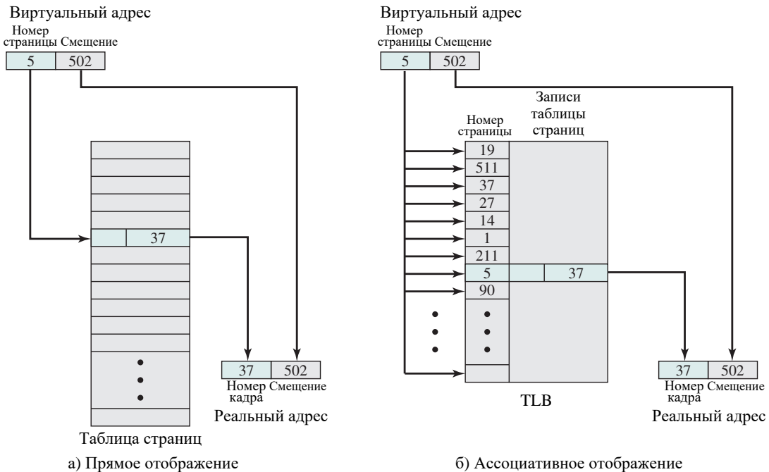
Рис. 8.8. Прямой и ассоциативный поиск записи таблицы страниц
