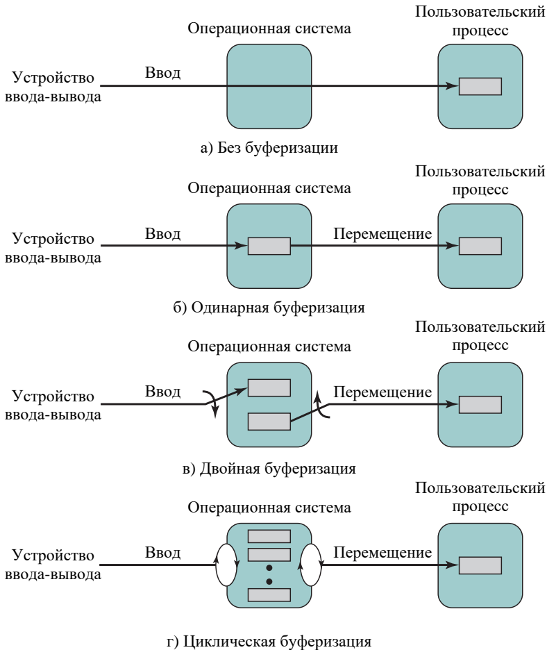
Рис. 11.5. Схемы буферизации ввода-вывода (ввод)
