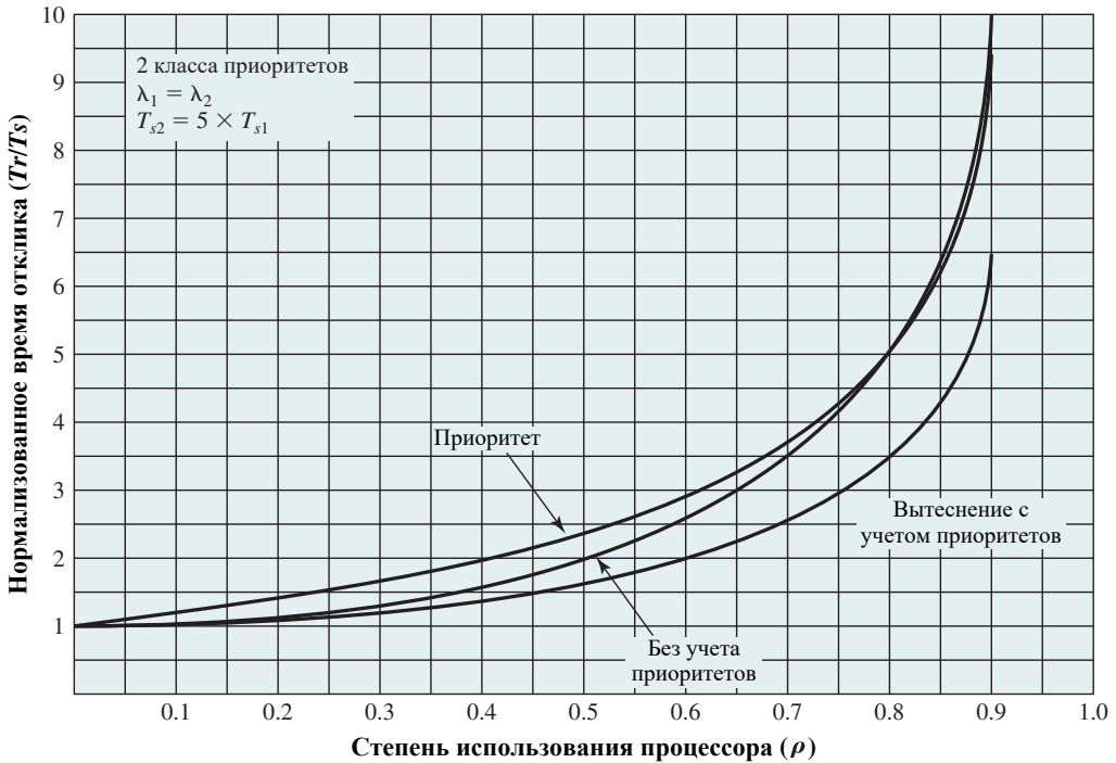
Рис. 9.11. Общее нормализованное время отклика
