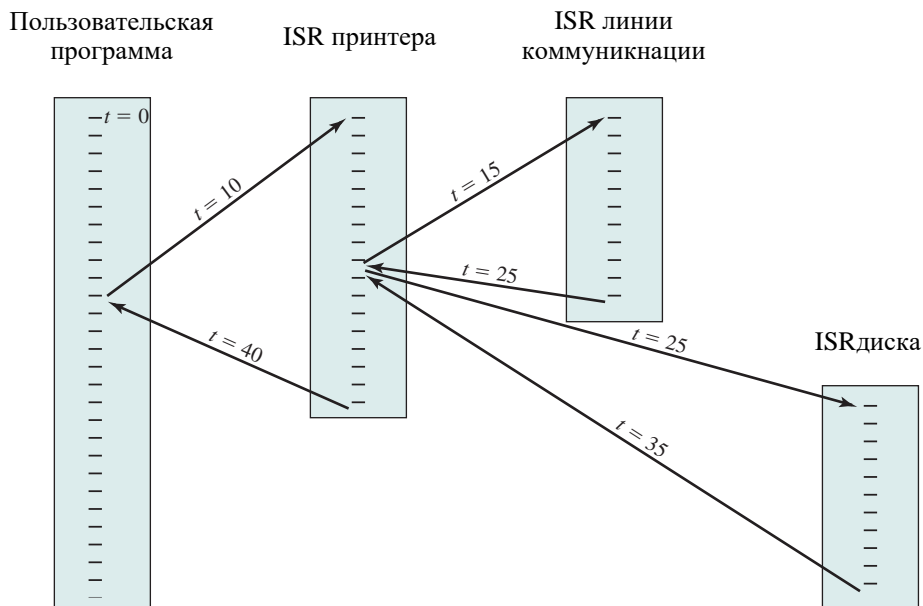
Рис. 1.13. Пример временной последовательности множественных прерываний
