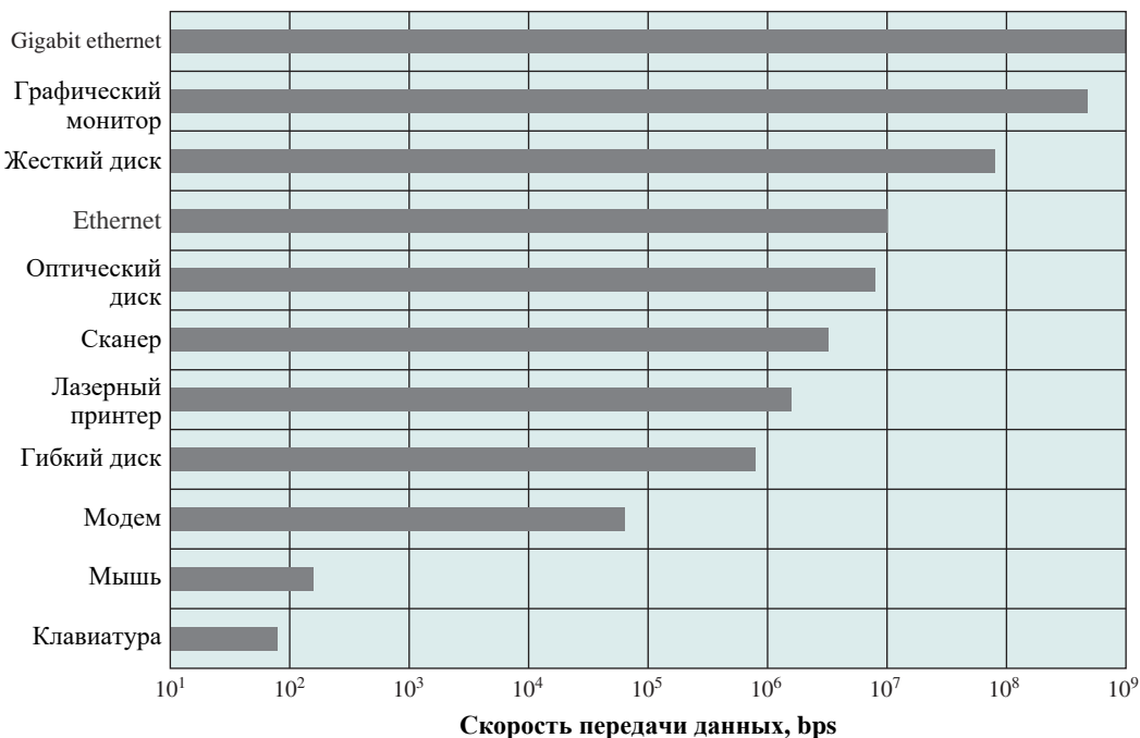
Рис. 11.1. Скорость передачи данных у типичных устройств ввода-вывода
