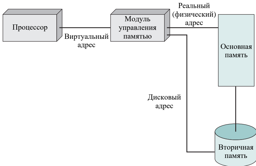
Рис. 2.10. Адресация виртуальной памяти
