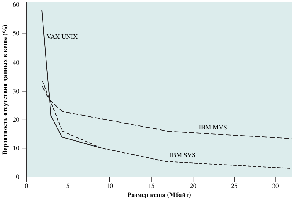
Рис. 11.10. Производительность дискового кеша при использовании LRU
