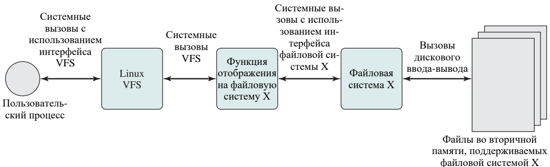
Рис. 12.18. Концепция VFS Linux
