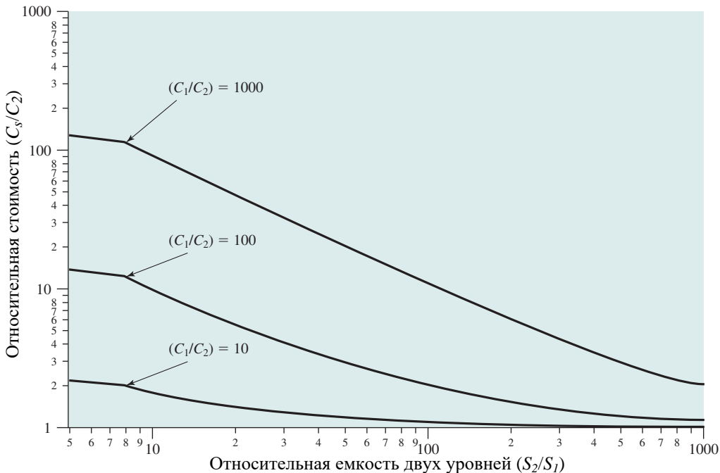
Рис. 1.22. Зависимость средней стоимости двухуровневой памяти от относительной емкости уровней
