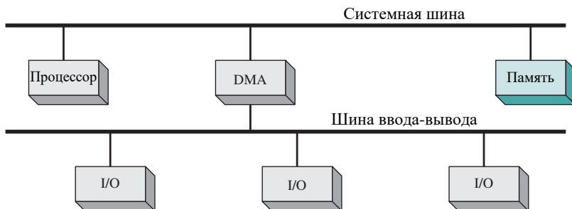
в) Шина ввода-вывода
