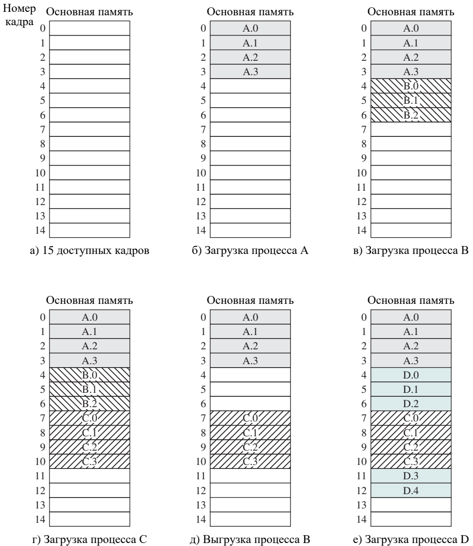
Рис. 7.9. Распределение страниц по свободным кадрам
