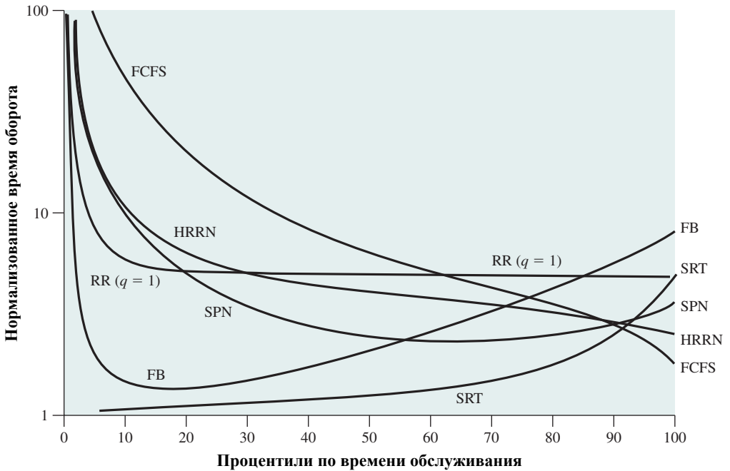
Рис. 9.14. Результаты имитационного моделирования для нормализованного времени оборота
