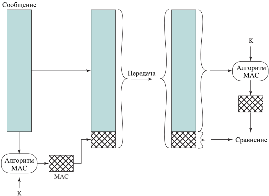
Рис. Л.3. Аутентификация сообщения с использованием MAC
