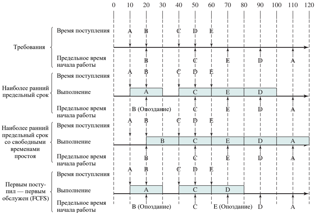
Рис. 10.6. Планирование неперiodических заданий реального времени с предельными сроками начала работы
