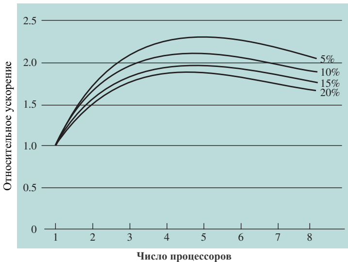
б) Ускорение с учетом накладных расходов
