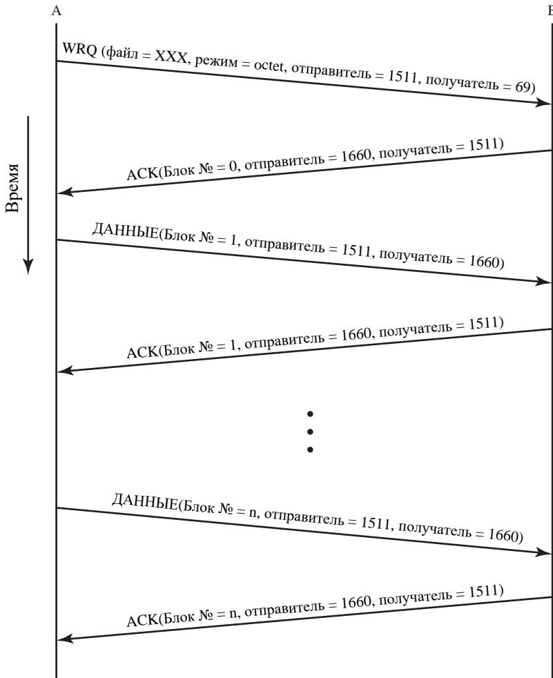
Рис. 17.11. Пример операции передачи файла по протоколу TFTP
