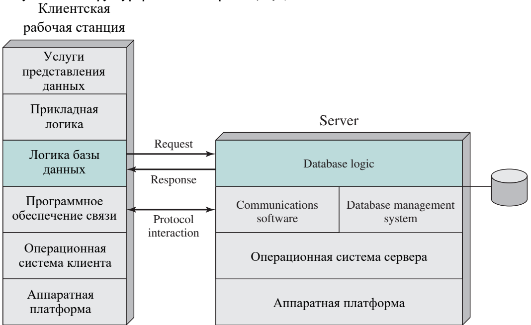
Рис. 18.3. Архитектура "клиент/сервер" для приложений баз данных
