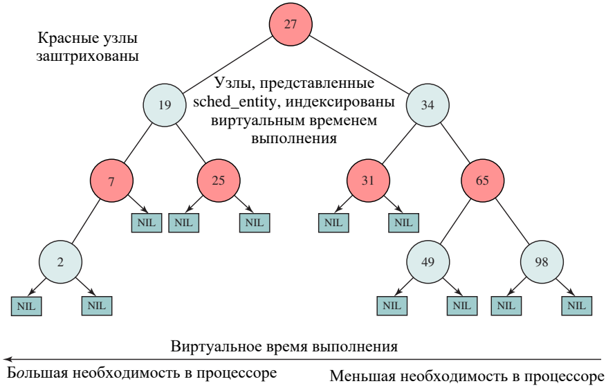
Рис. 10.11. Пример применения красно-черного дерева для CFS
