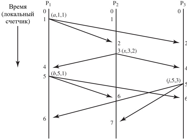
Рис. 19.8. Пример операции по алгоритму присваивания отметки времени
