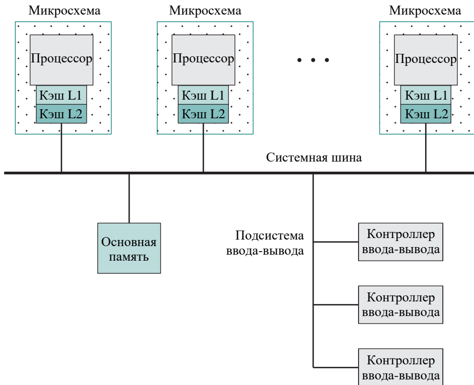
Рис. 1.19. Организация SMP
