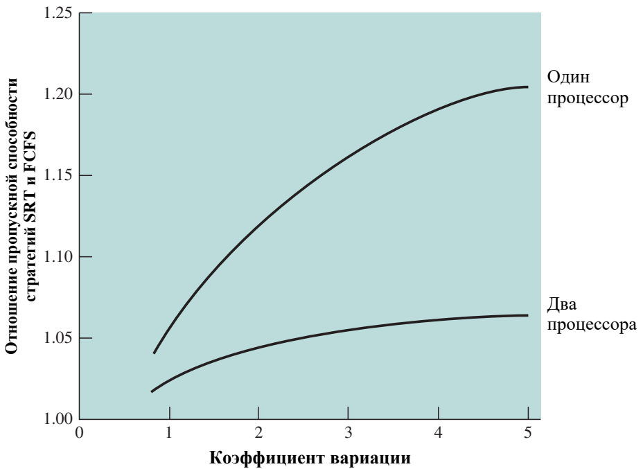
б) Сравнение стратегий SRT и FCFS
