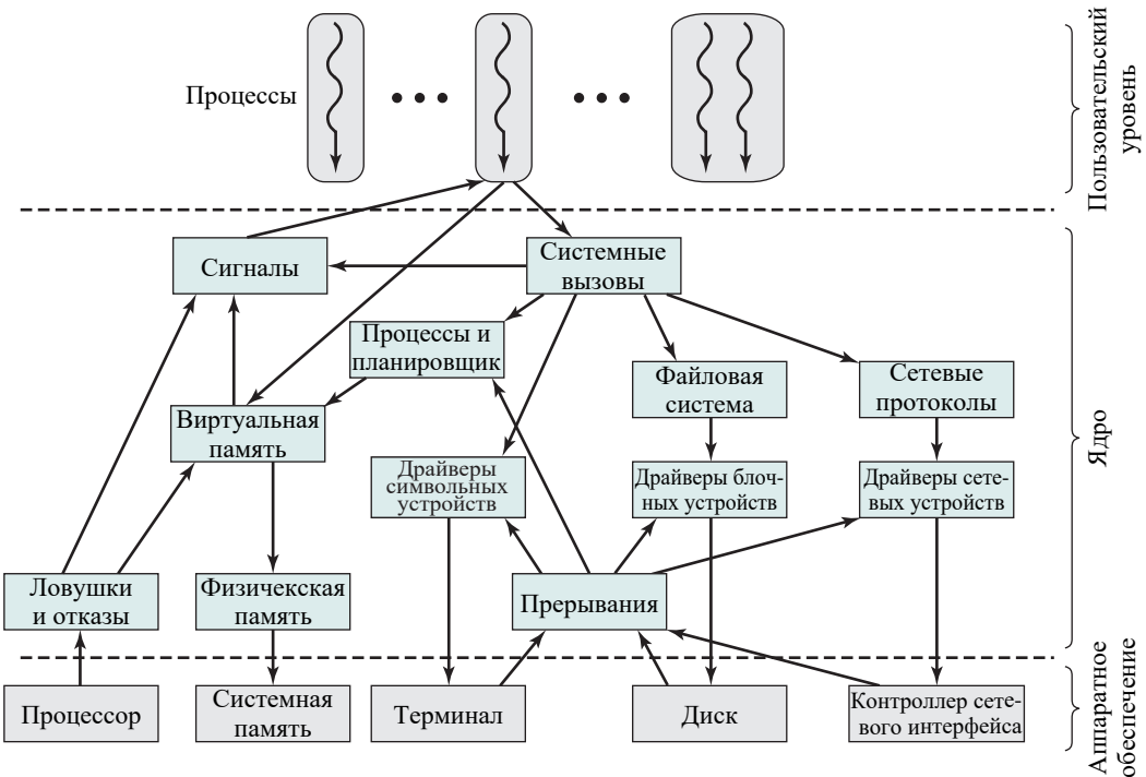
Рис. 2.19. Компоненты ядра Linux
