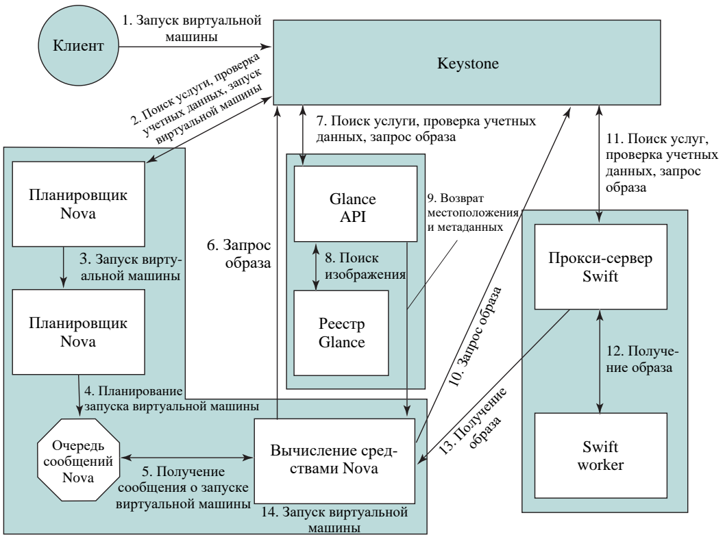
Рис. 16.11. Запуск виртуальной машины
