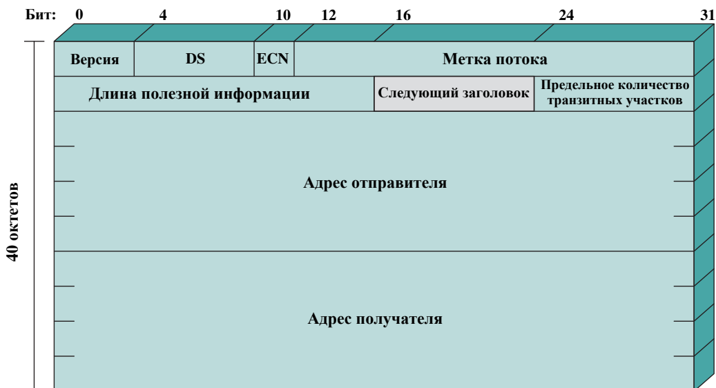
б) Заголовок пакета IPv6
