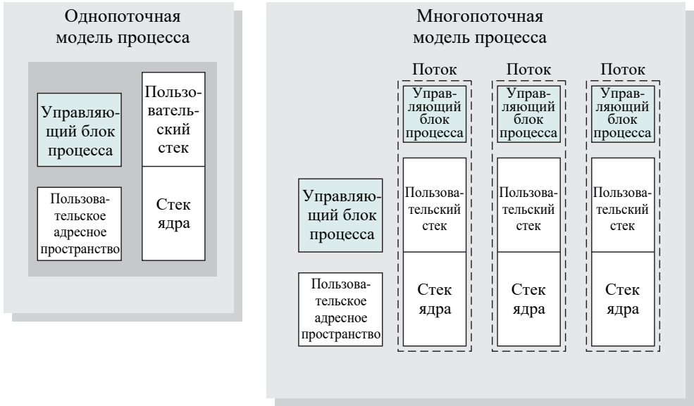
Рис. 4.2. Однопоточная и многопоточная модели процесса
