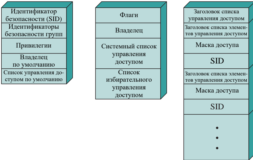
а) Токен доступа б) Дескриптор безопасности в) Список управления доступом
