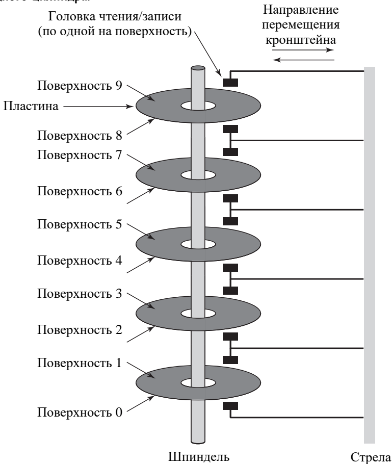
Рис. К.3. Компоненты магнитного диска
