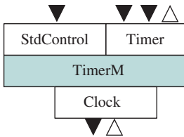
(a) Компонент TimerM
