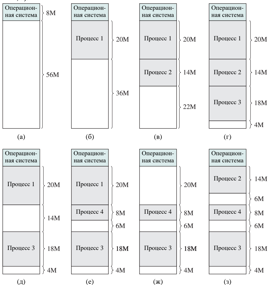
Рис. 7.4. Пример динамического распределения
