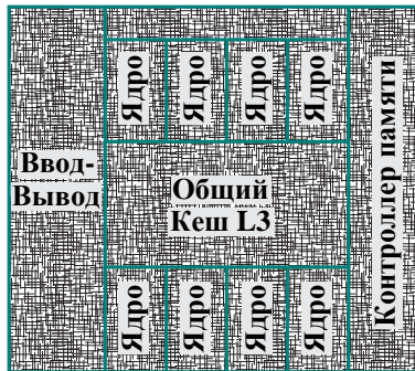
б) Физическое размещение на плате
