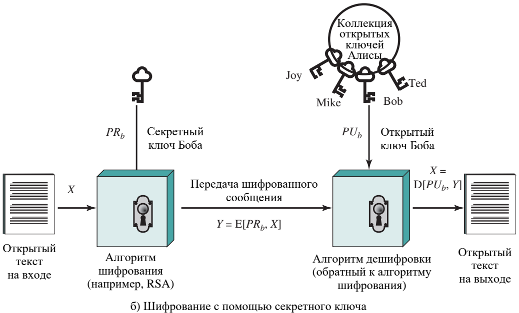
Рис. Л.2. Шифрование с открытым ключом
