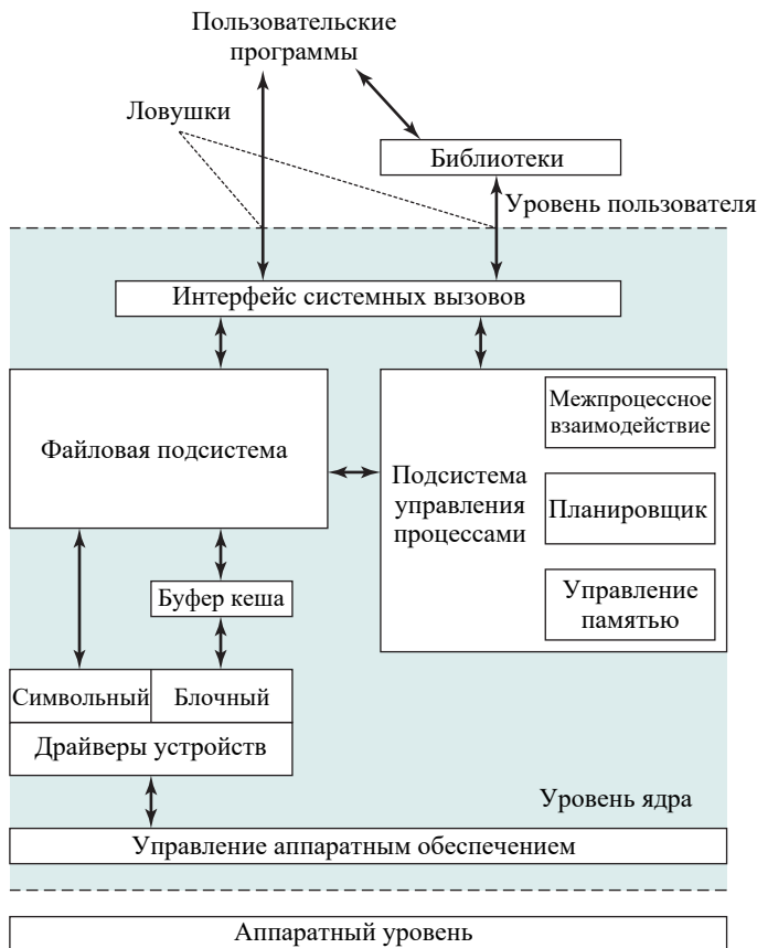
Рис. 2.15. Традиционная архитектура UNIX
