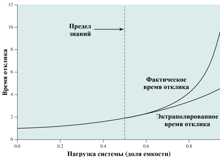
Рис. 21.1. Сравнение планируемого и фактического времени отклика
