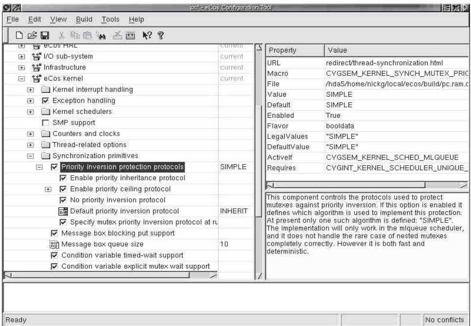
Рис. Р.2. Инструмент конфигурирования eCos: детали ядра
