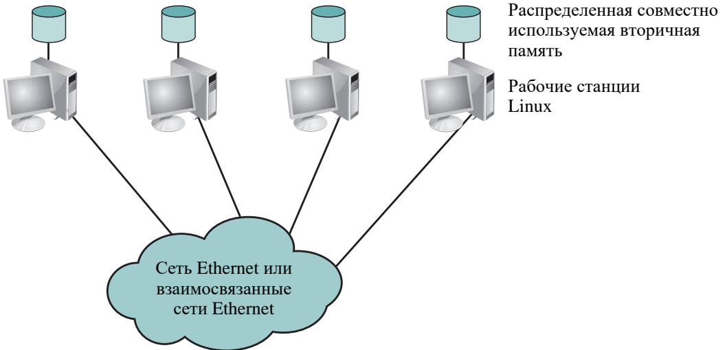
Рис. 18.16. Типичная конфигурация Beowulf
