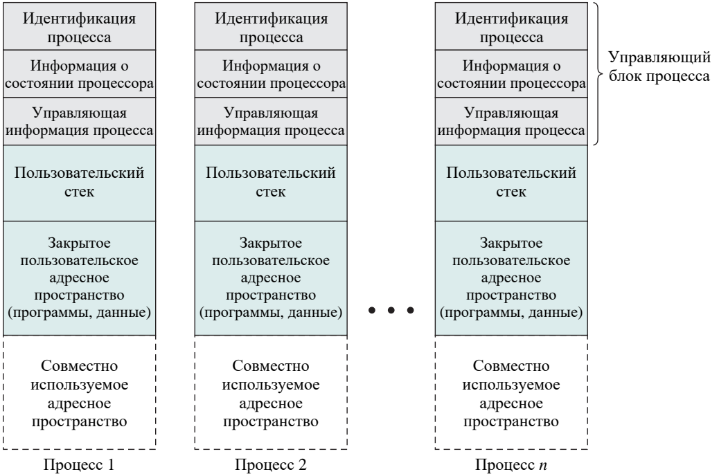
Рис. 3.13. Пользовательские процессы в виртуальной памяти
