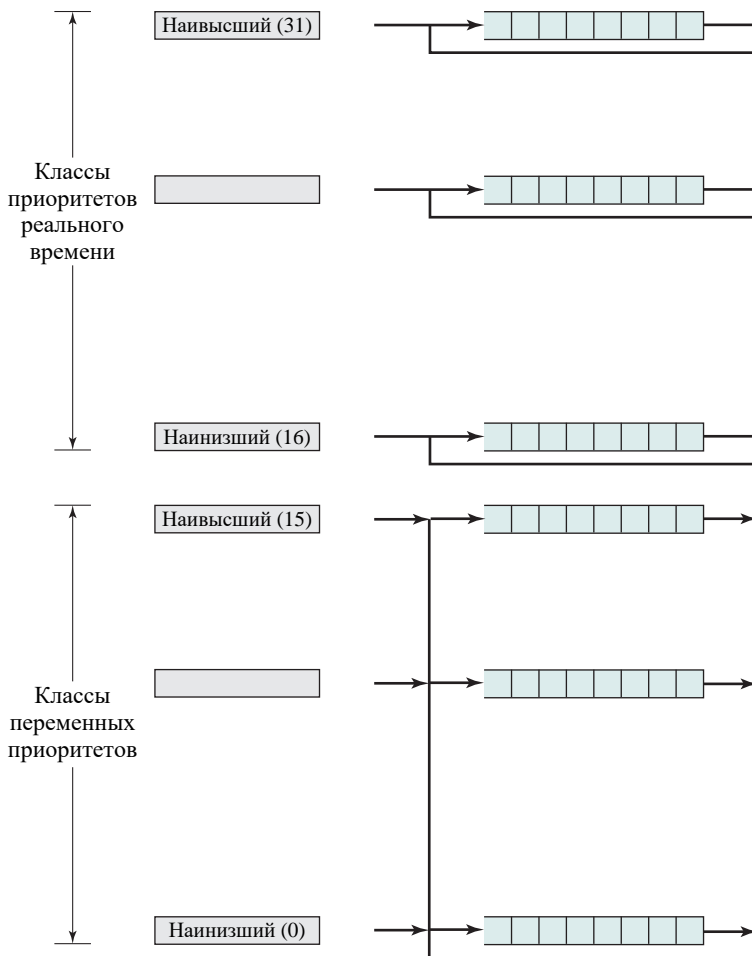
Рис. 10.14. Приоритеты потоков Windows
