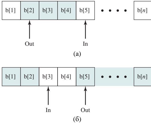
Рис. 5.15. Конечный циклический буфер для задачи “производитель/потребитель”
