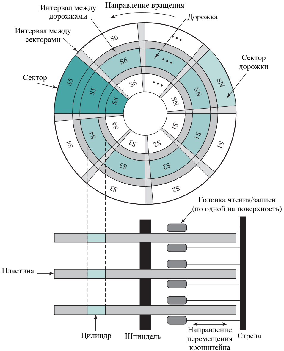
Рис. К.1. Схема размещения данных на диске
