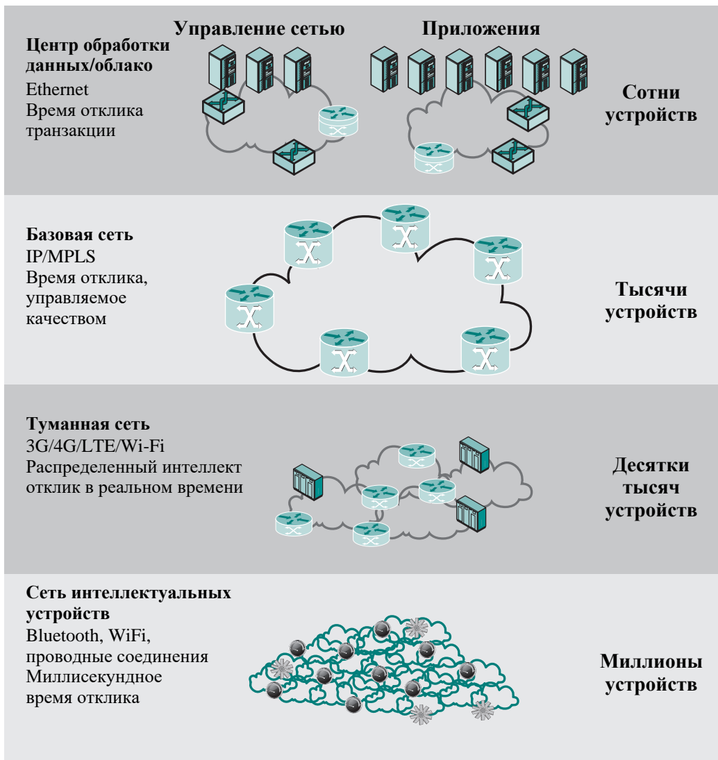
Рис. 16.12. Контекст Интернета вещей
