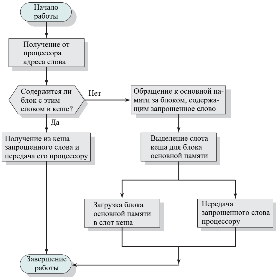
Рис. 1.18. Операция чтения из кеша
