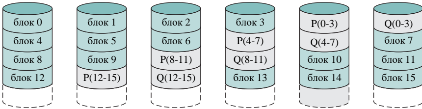
ж) RAID 6 (двойная распределенная четность с чередующимися блоками)
