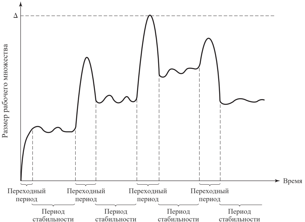
Рис. 8.18. Типичная диаграмма изменения размера рабочего множества [161]
