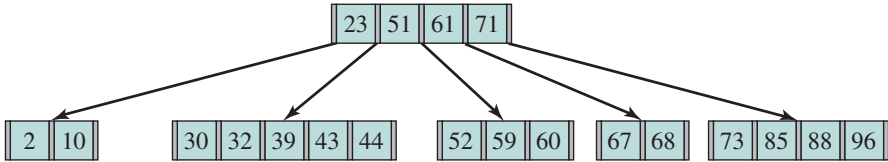
а) В-дерево с минимальной степенью d=3
