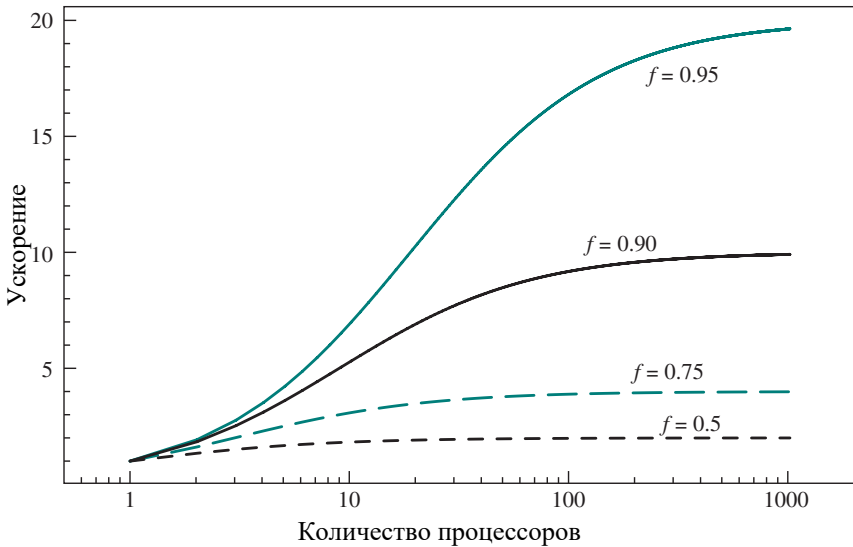
Рис. Д.1. Закон Амдала для многопроцессорных систем
