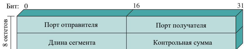
б) Заголовок пакета UDP
