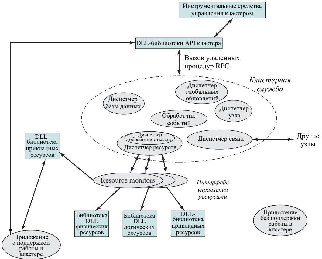
Рис. 18.15. Блок-схема кластерного сервера в Windows
