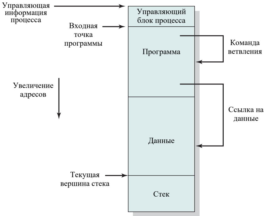
Рис. 7.1. Требования к адресации процесса
