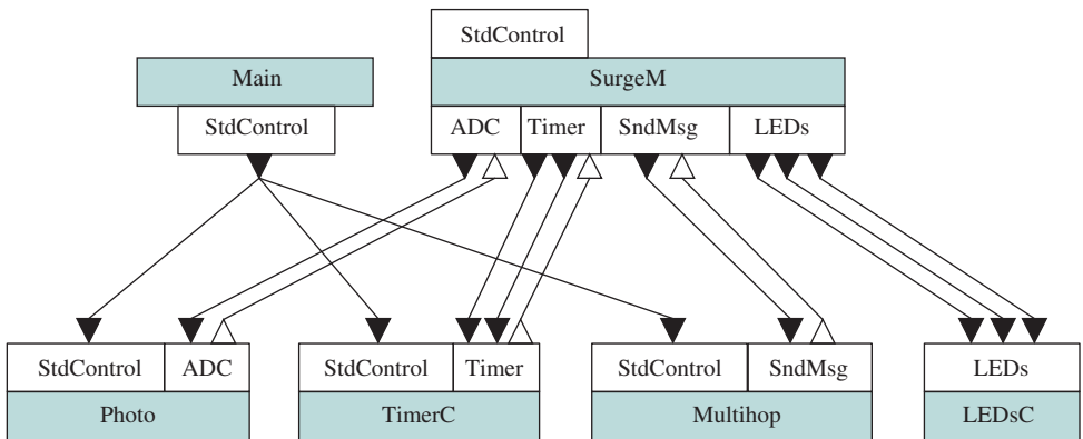
б) Конфигурация Surge высокого уровня
