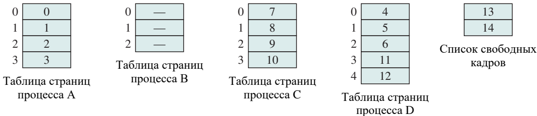
Рис. 7.10. Структуры данных, соответствующие примеру на рис. 7.9, е
