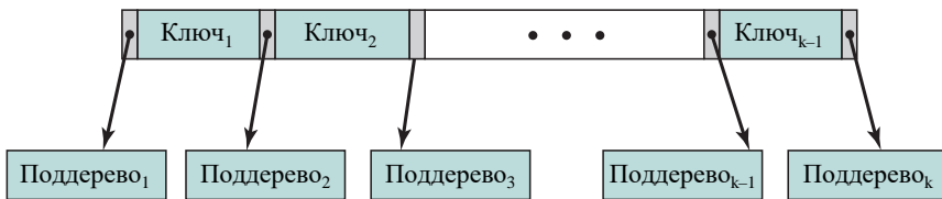
Рис. 12.4. Узел В-дерева с k дочерними узлами
