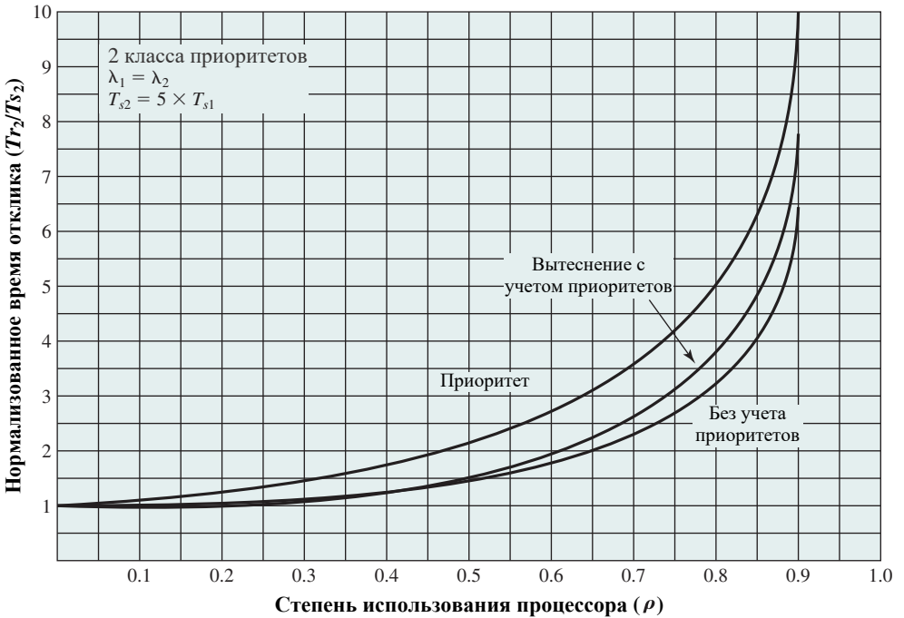
Рис. 9.13. Нормализованное время отклика для длинных процессов
