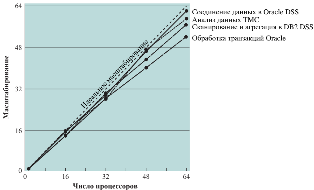
Рис. 4.8. Масштабирование загрузок баз данных в многопроцессорных системах
