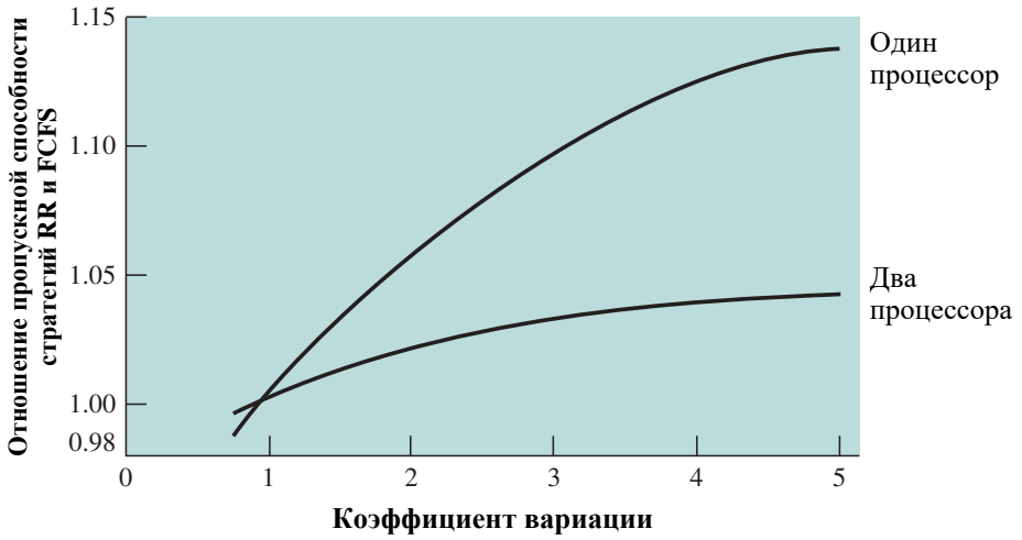
а) Сравнение стратегий RR и FCFS
