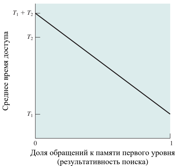
Рис. 1.15. Производительность простой двухуровневой системы
