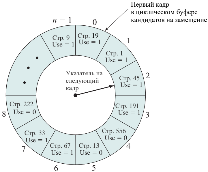
а) Состояние буфера непосредственно перед замещением страницы
