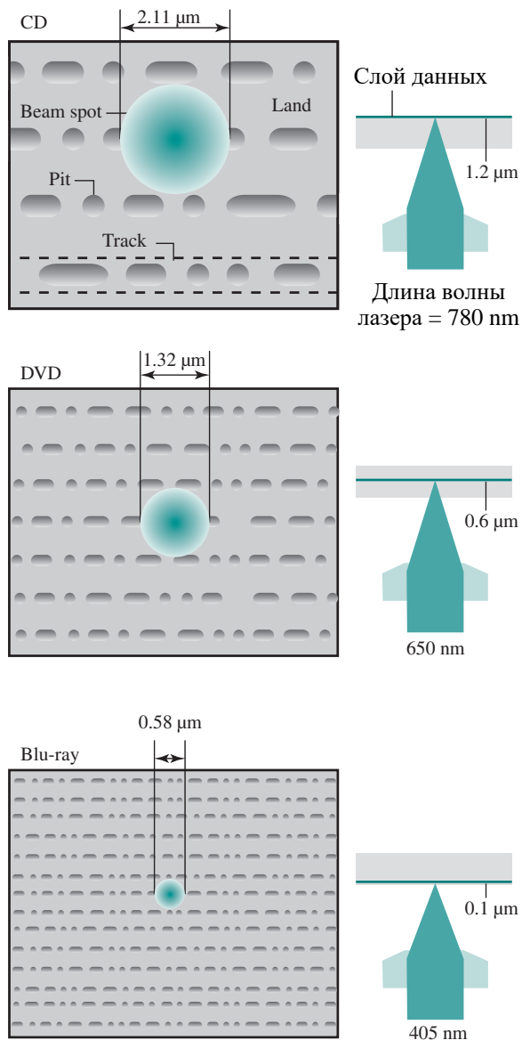
Рис. К.6. Характеристики оптических накопителей
