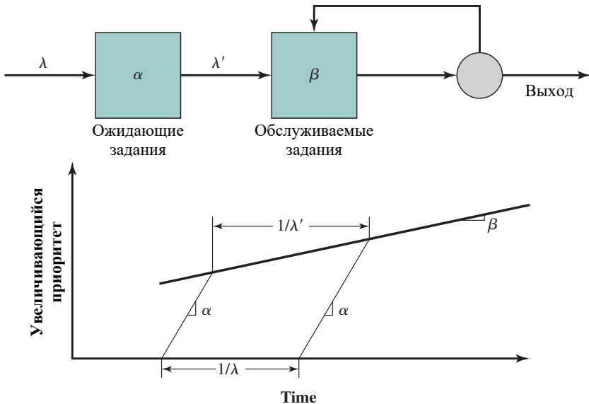
Рис. 9.19. Эгоистичное круговое планирование
