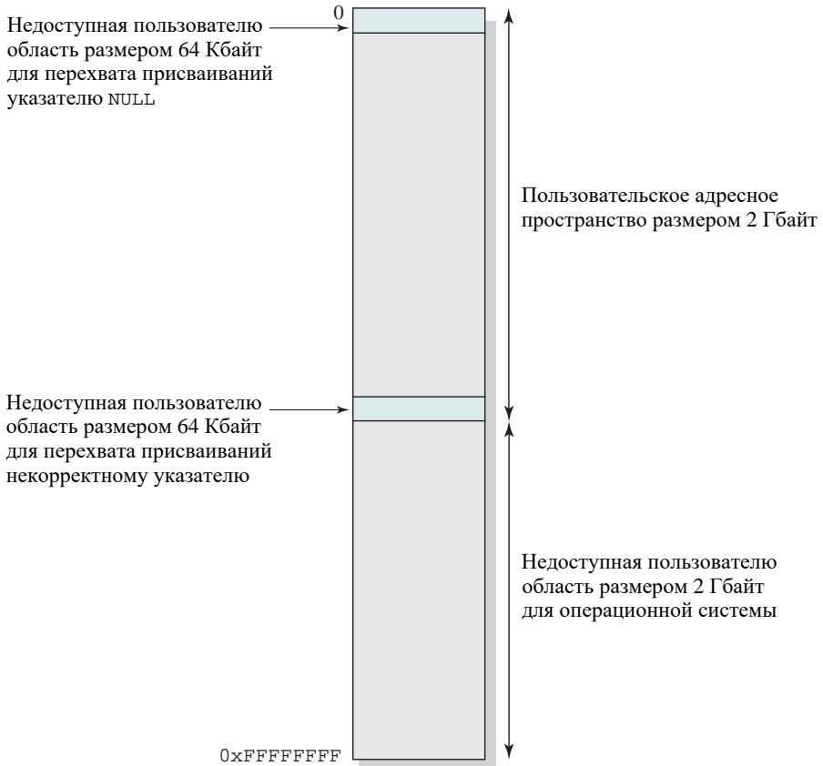
Рис. 8.25. 32-битное виртуальное адресное пространство Windows по умолчанию
