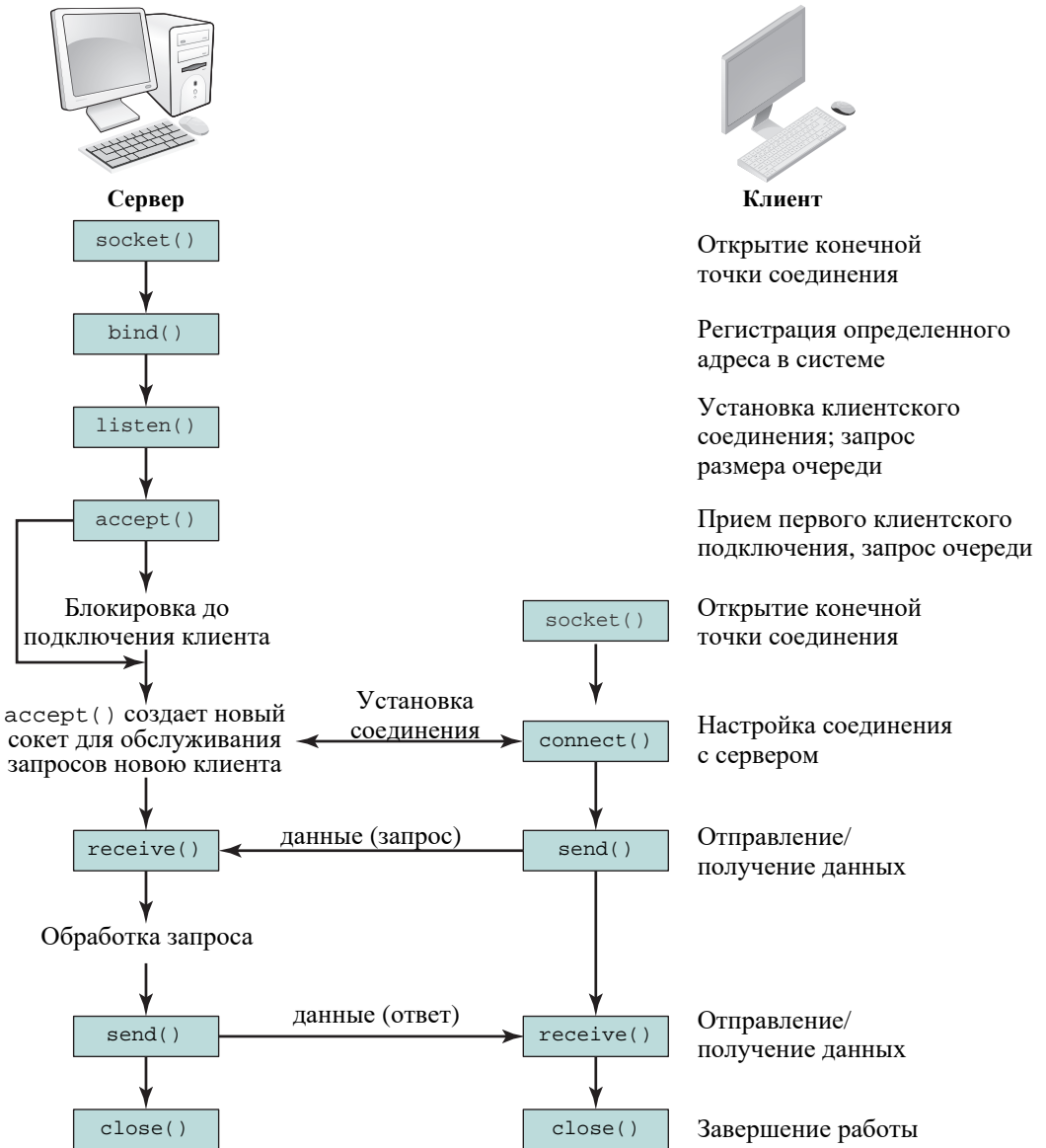
Рис. М.2. Системные вызовы сокетов для ориентированного на соединения протокола
