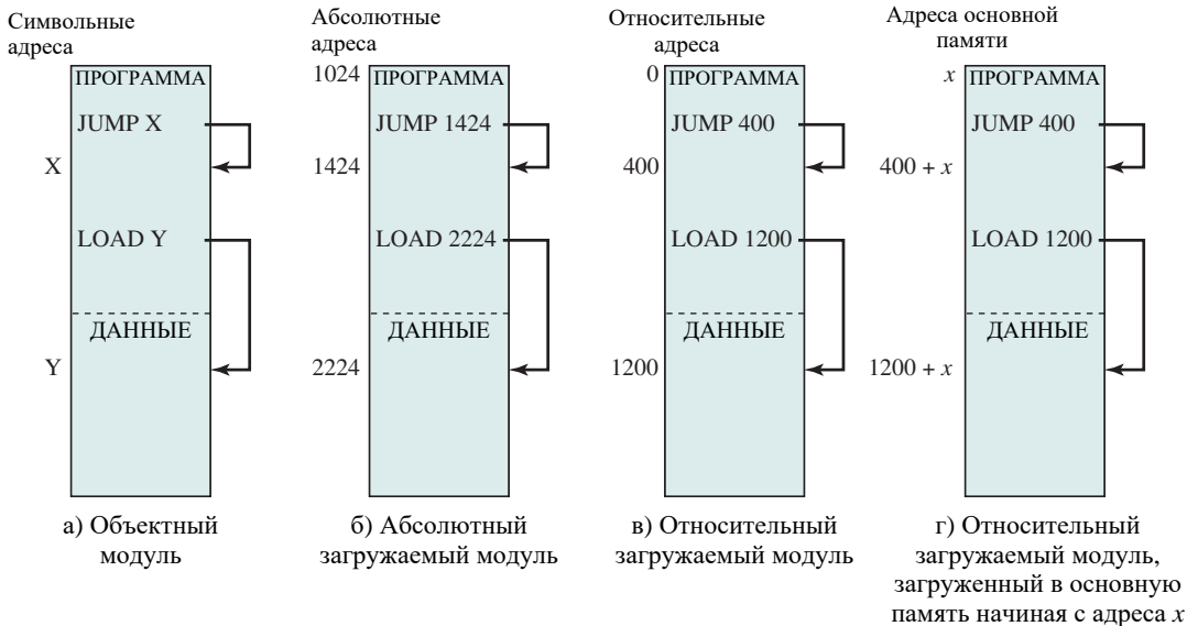
Рис. 7.15. Абсолютные и перемещаемые загружаемые модули
