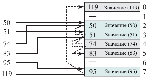
а) Линейное хеширование
