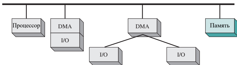
б) Одиночная шина, интегрированный DMA-I/O
