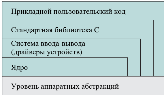
Рис. P.4. Многоуровневая структура eCos
