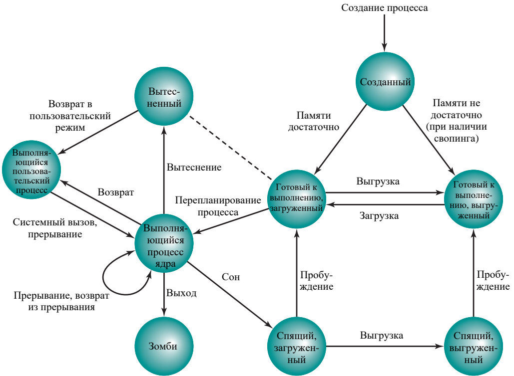
Рис. 3.17. Диаграмма переходов между состояниями процессов в системе UNIX
