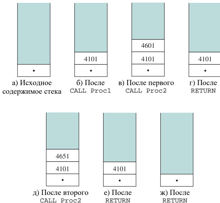
Рис. П.3. Использование стека при реализации вложенных процедур на рис. П.2
