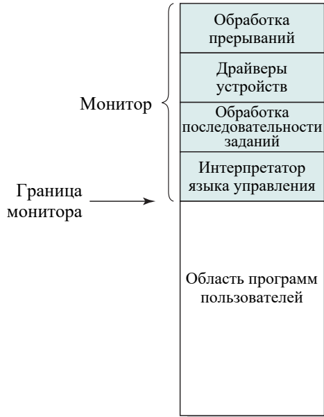
Рис. 2.3. Схема размещения резидентного монитора в памяти
