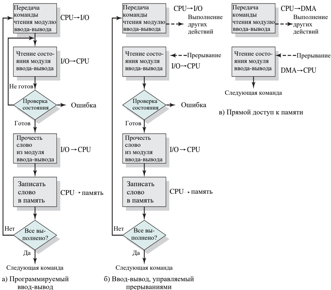
Рис. В. 1. Три метода передачи блока входных данных
