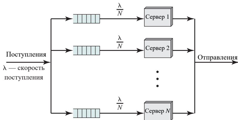
б) Несколько одноканальных систем массового обслуживания
