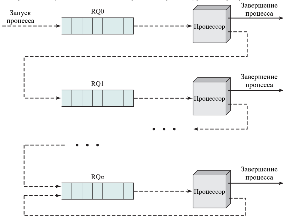
Рис. 9.10. Планирование со снижением приоритета
