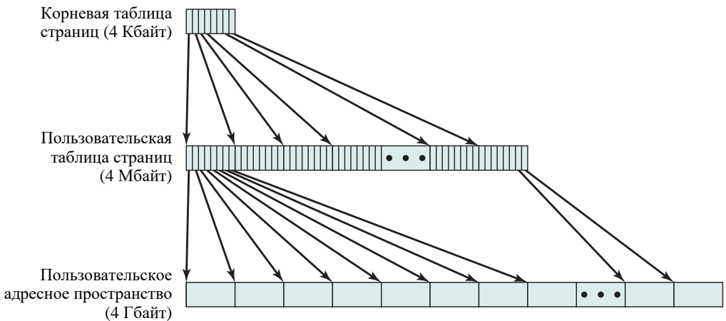
Рис. 8.3. Двухуровневая иерархическая таблица страниц
