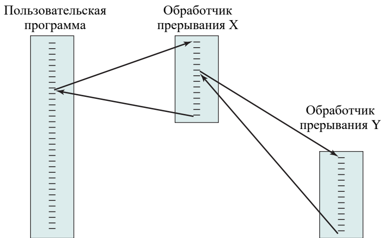
б) Вложенная обработка прерываний
