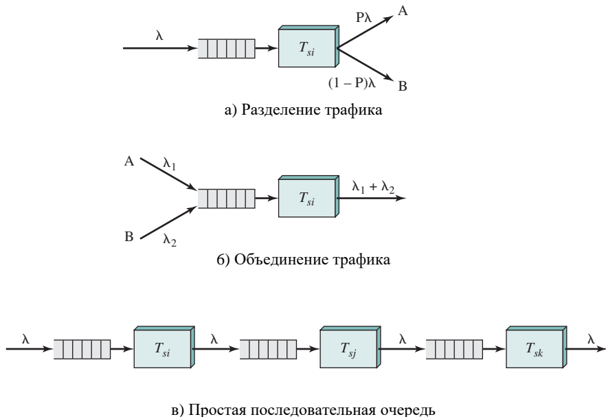
Рис. 21.8. Элементы сети очередей
