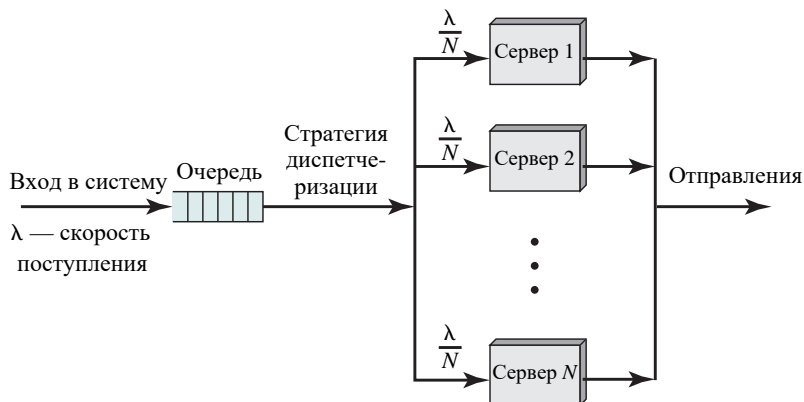
а) Многоканальная система массового обслуживания
