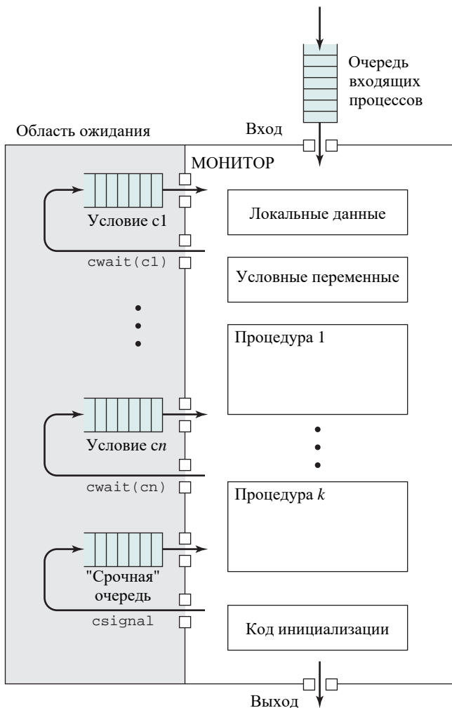
Рис. 5.18. Структура монитора
