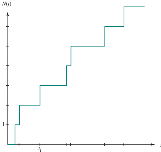
а) Пуассоновский процесс подсчета
