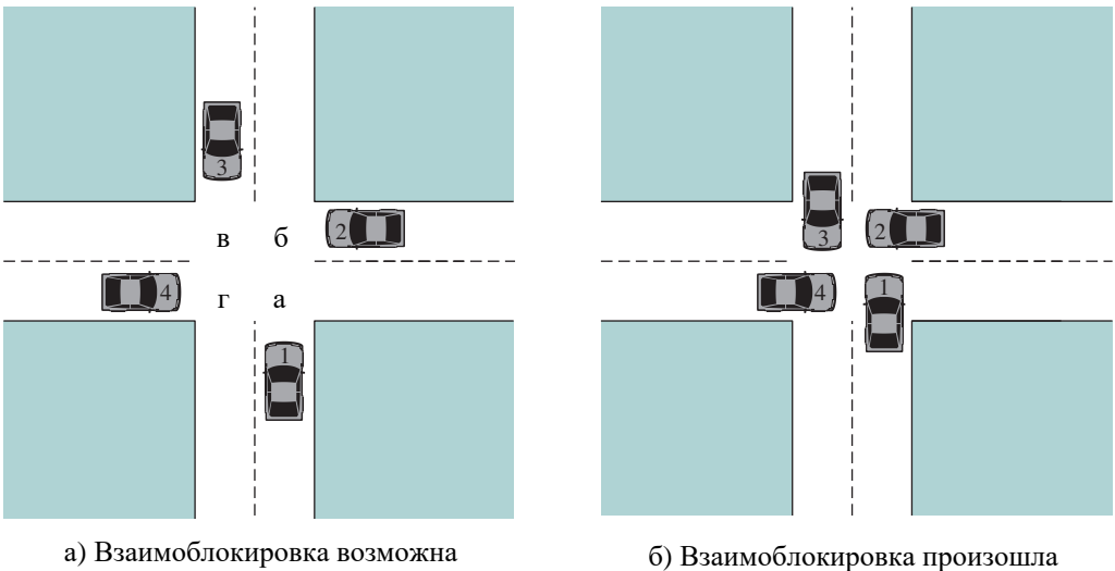
Рис. 6.1. Пример взаимоблокировки
