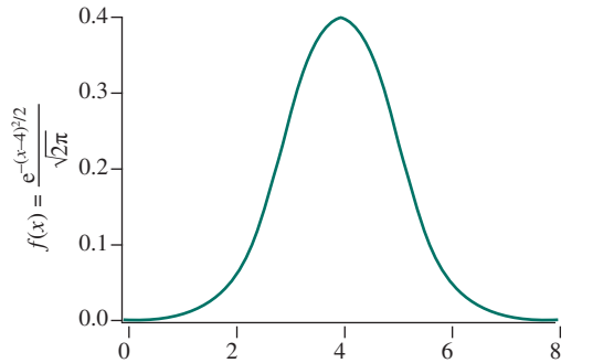
г) Плотность нормального распределения вероятности ( \mu = 4, \sigma = 1 )
