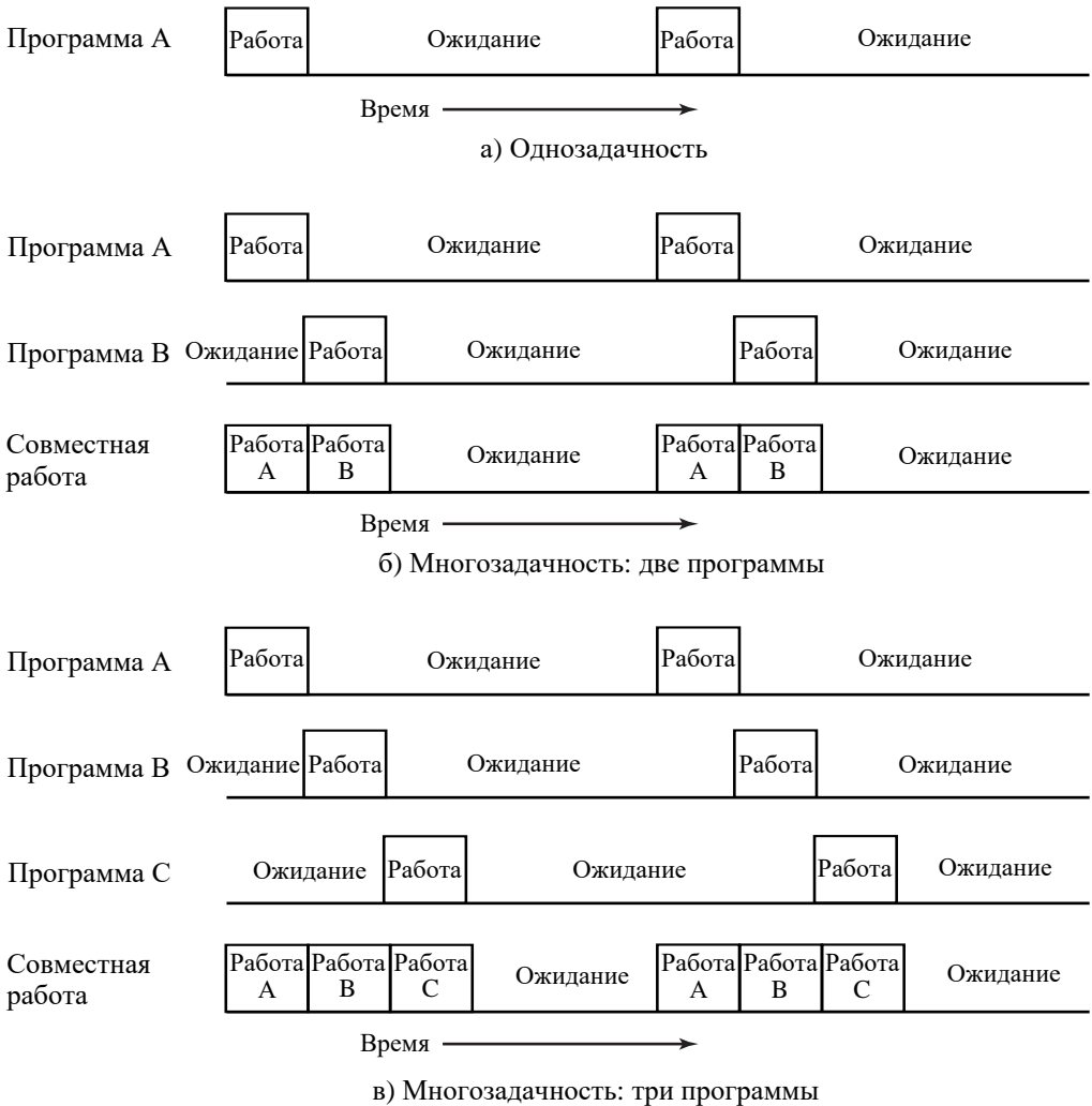
Рис. 2.5. Пример многозадачности
