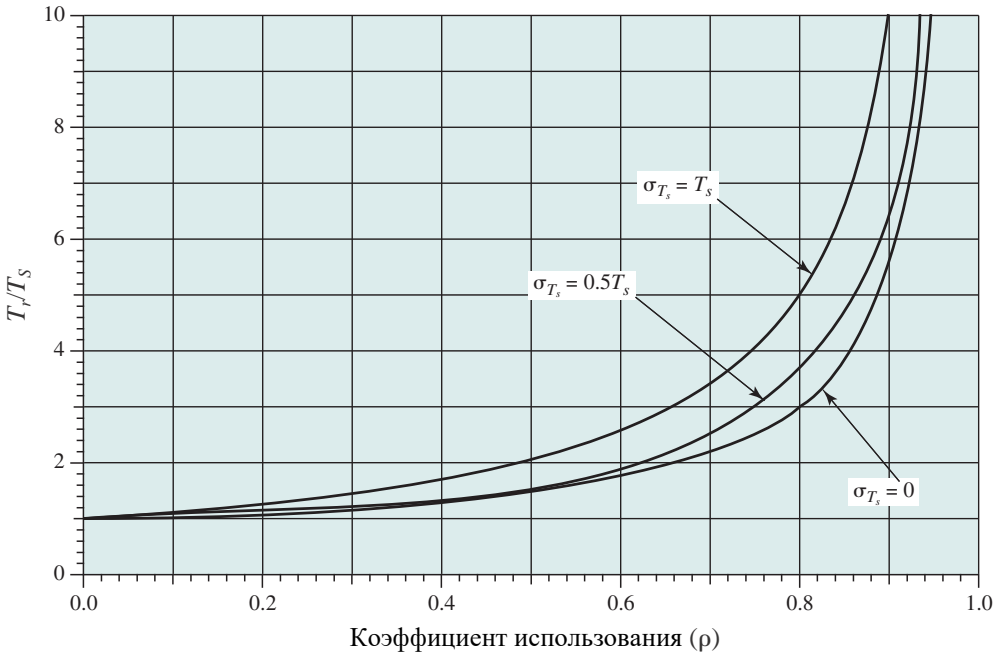
Рис. 21.6. Среднее время пребывания в одноканальной системе массового обслуживания
