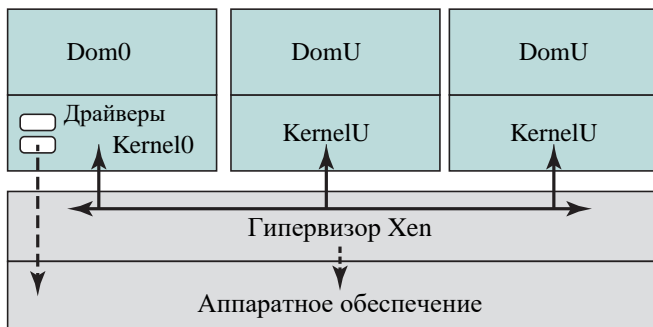
Рис. 14.10. Архитектура Xen
