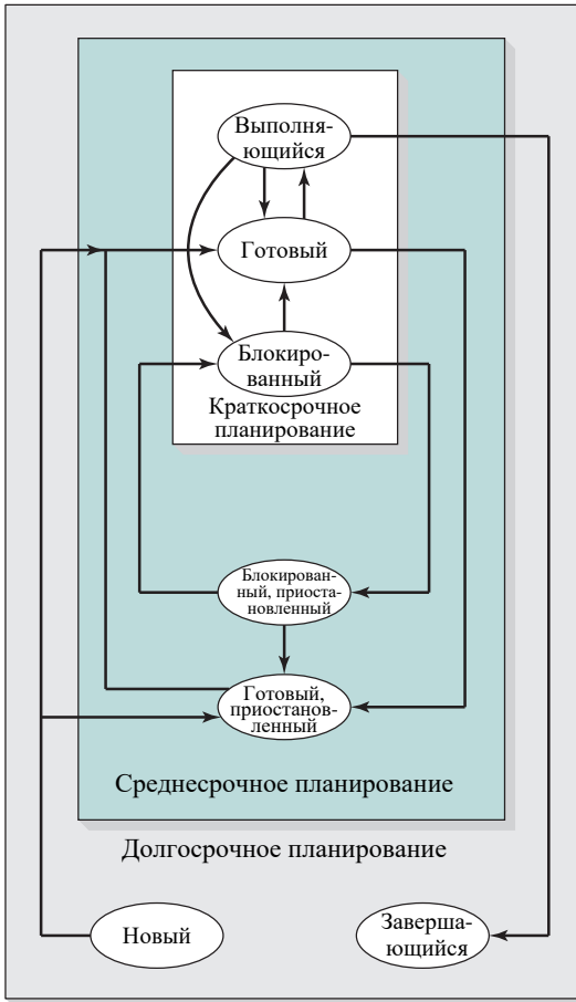
Рис. 9.2. Уровни планирования
