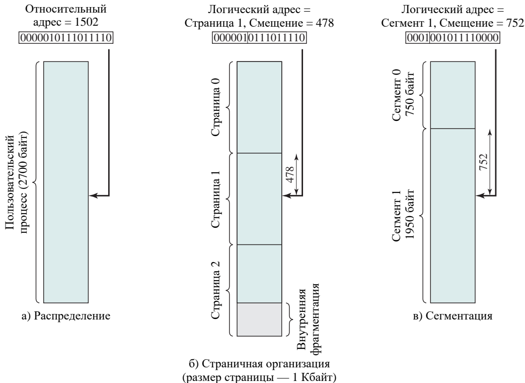
Рис. 7.11. Логические адреса
