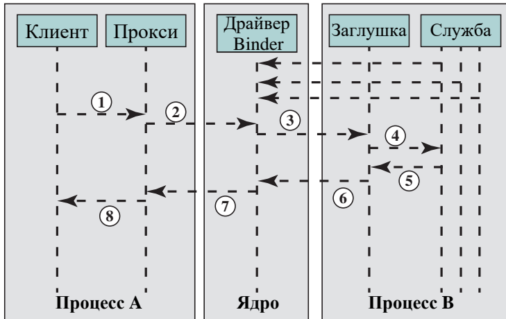
Рис. 6.16. Операции Binder
