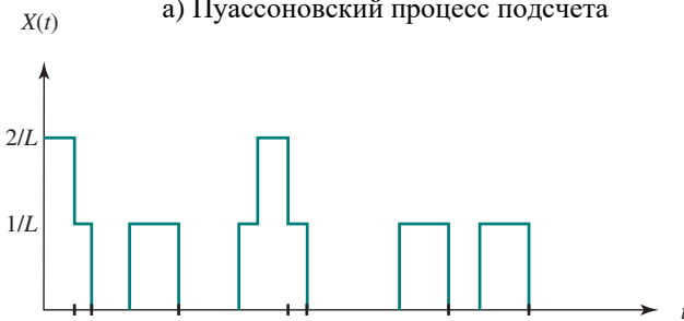
б) Пуассоновский процесс приращения
