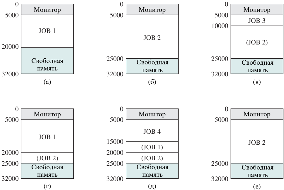
Рис. 2.7. Работа CTSS
