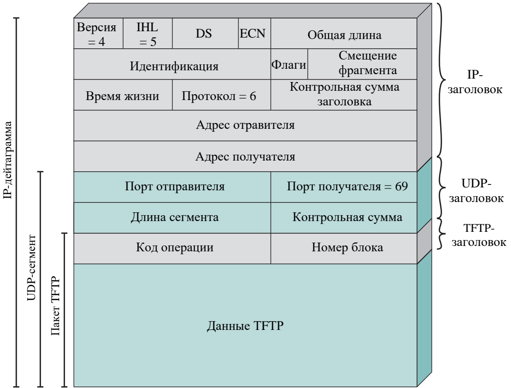
Рис. 17.10. Пакет TFTP
