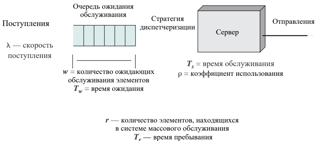
Рис. 21.2. Структура и параметры одноканальной системы массового обслуживания
