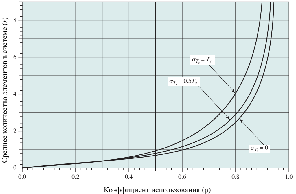
Рис. 21.5. Среднее количество элементов в одноканальной системе массового обслуживания
