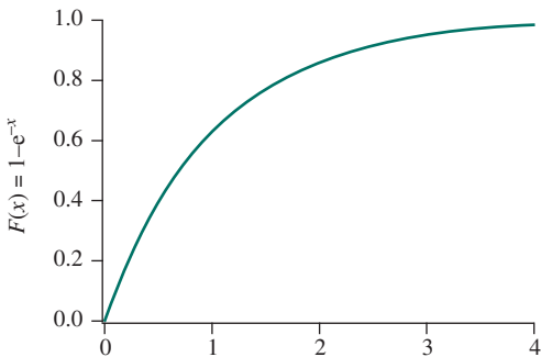
а) Экспоненциальное распределение вероятности ( \lambda = 1 )
