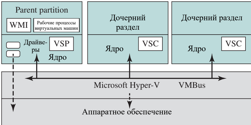
Рис. 14.11. Архитектура Hyper-V
