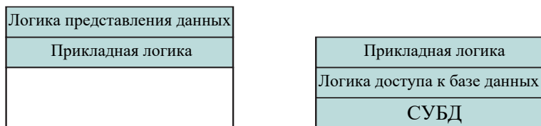
в) Совместная обработка данных
