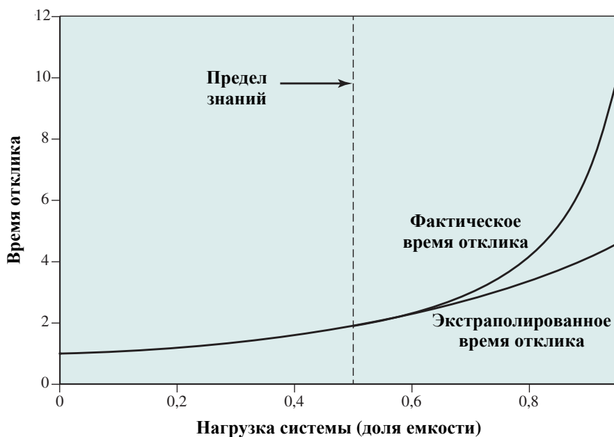
Рис. 3.1. Экстраполированное и фактическое время отклика
