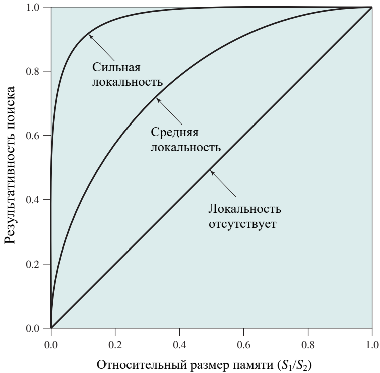
Рис. 1.24. Результативность поиска в зависимости от относительного размера памяти
