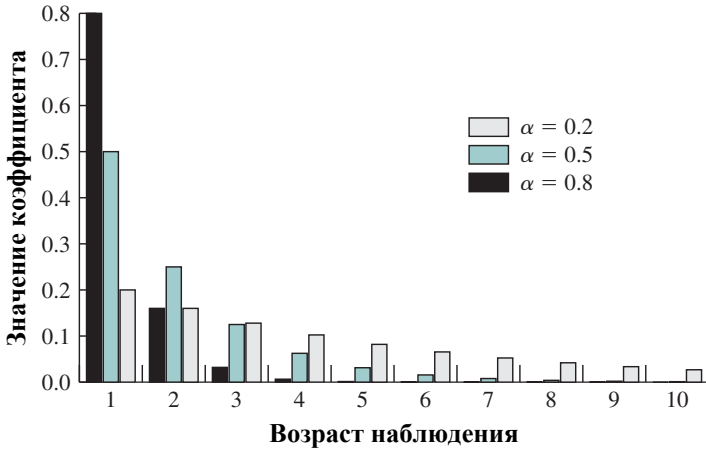
Рис. 9.8. Весовые коэффициенты при разных значениях \alpha
