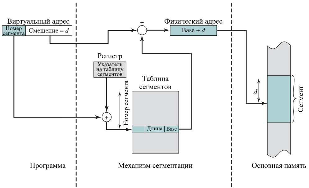
Рис. 8.11. Трансляция адреса в системе с сегментацией
