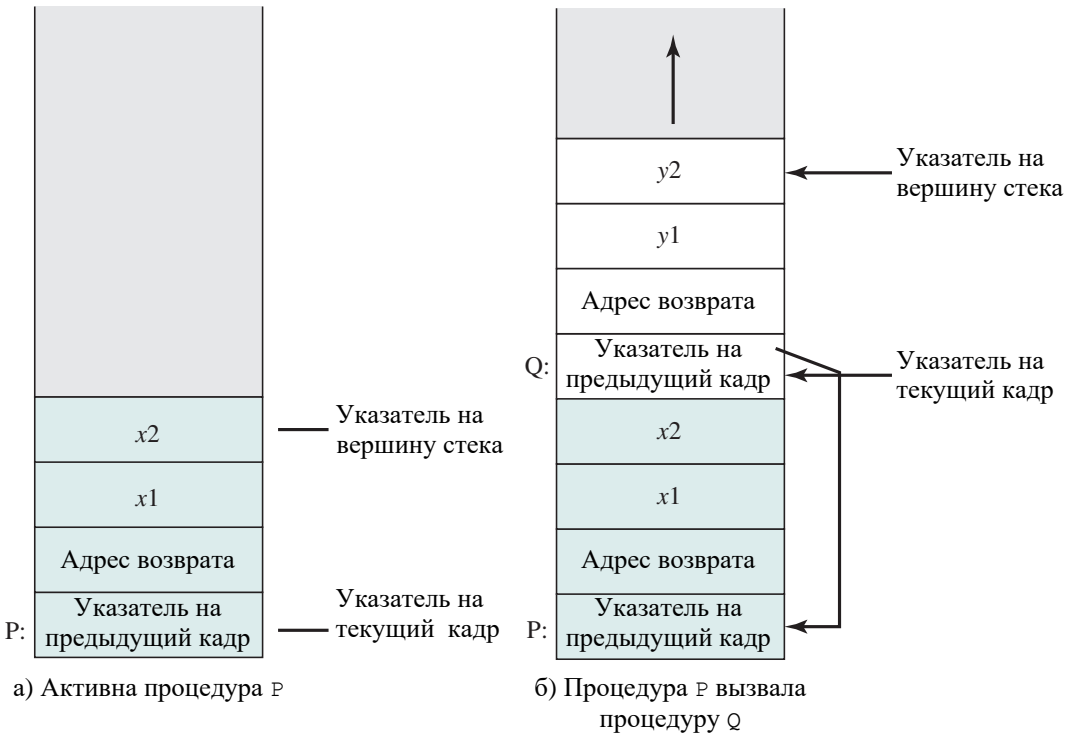
Рис. П.4. Рост стека при вызове процедур Р и Q
