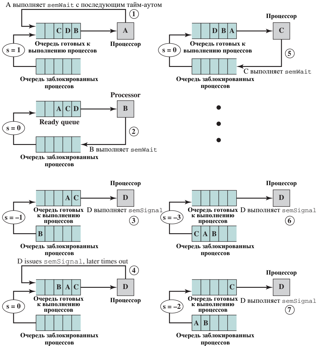
Рис. 5.8. Пример работы семафора
