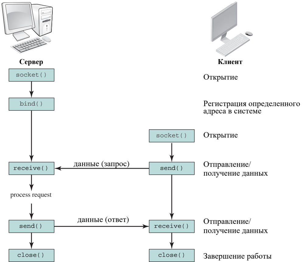
Рис. М.3. Системные вызовы сокетов для протокола без соединения
