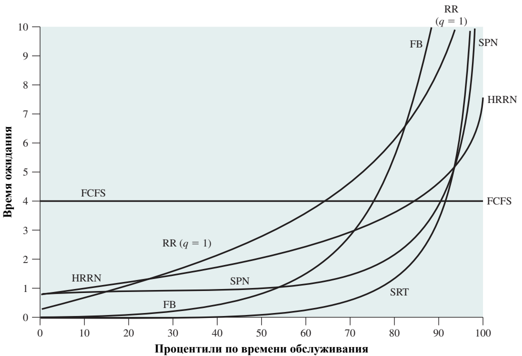
Рис. 9.15. Результаты имитационного моделирования для времени ожидания
