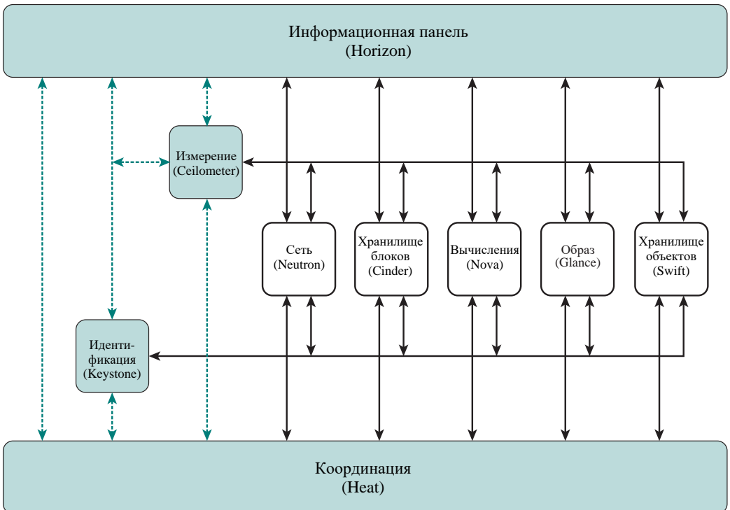
Рис. 16.9. Обобщенная архитектура ОС OpenStack
