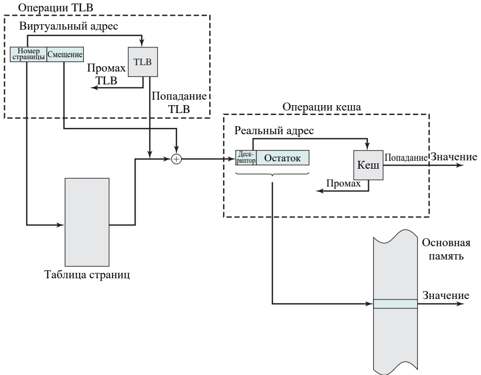
Рис. 8.9. Работа кеша и TLB
