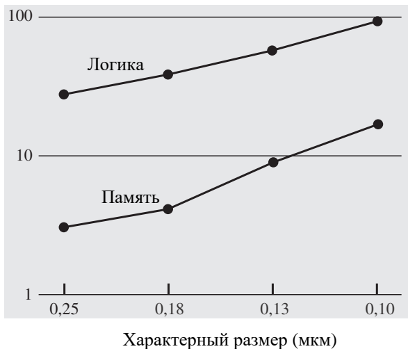
Рис. В.3. Энергопотребление процессоров
