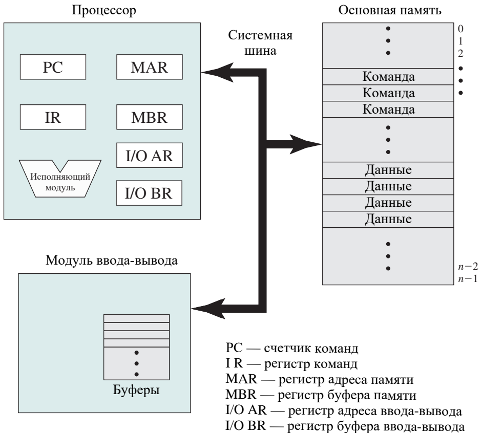
Рис. 1.1. Компоненты компьютера: общая структура
