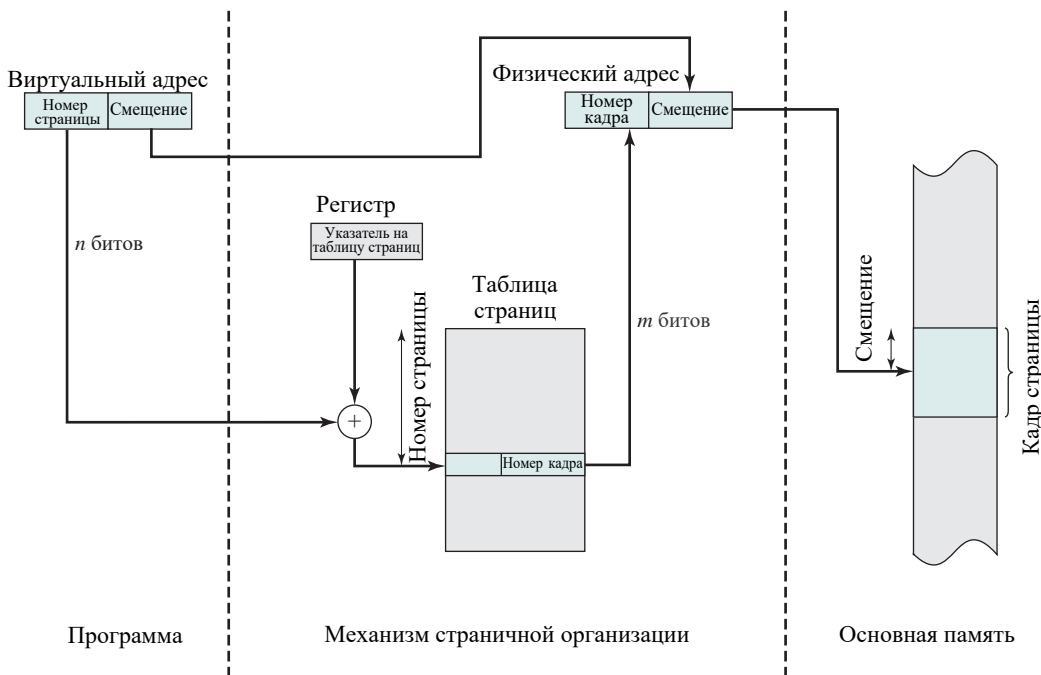
Рис. 8.2. Трансляция адреса в системе со страничной организацией
