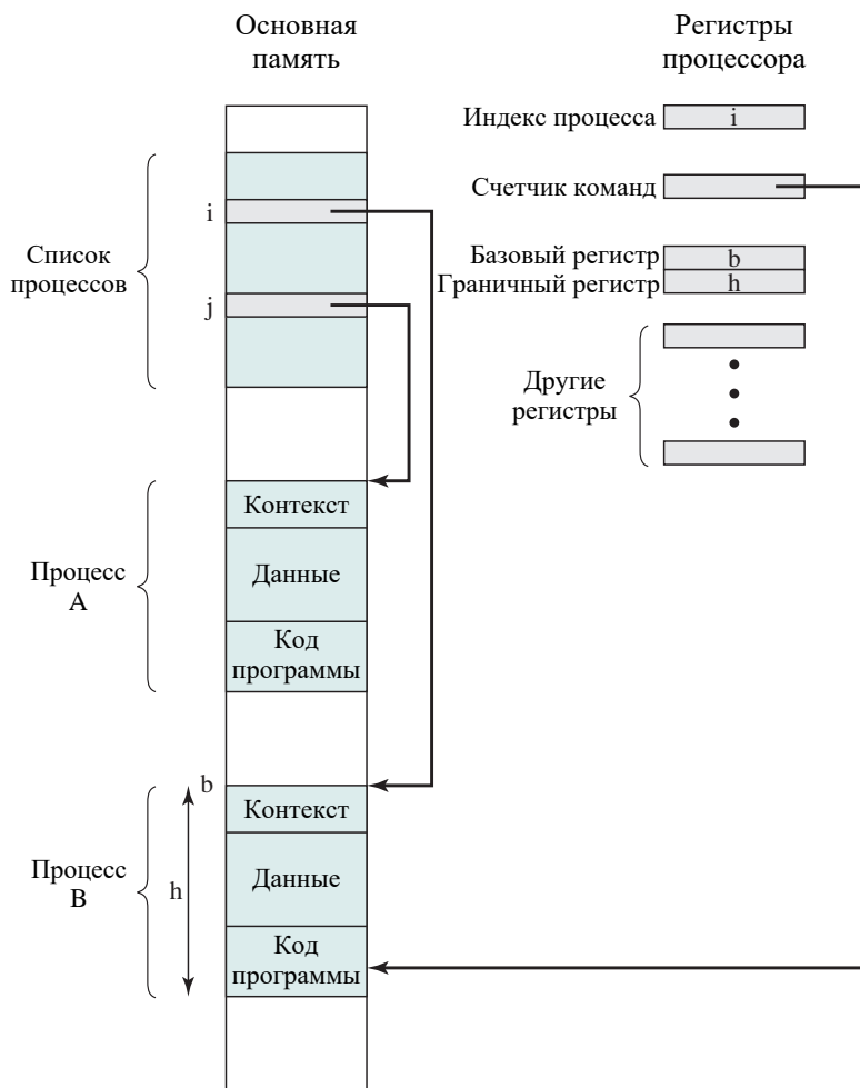
Рис. 2.8. Типичная реализация процессов
