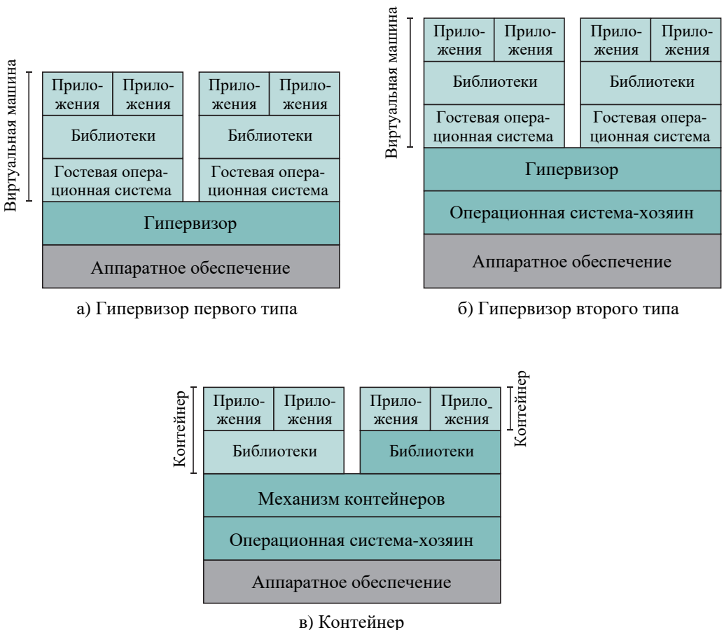
Рис. 14.4. Сравнение виртуальных машин и контейнеров
