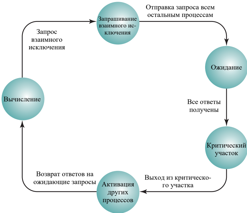
Рис. 19.10. Диаграмма перехода в разные состояния для алгоритма, предложенного в [201]
