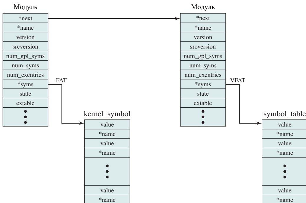
Рис. 2.18. Пример списка модулей ядра операционной системы Linux
