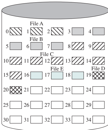
Рис. 12.10. Непрерывное размещение файлов (после уплотнения)
