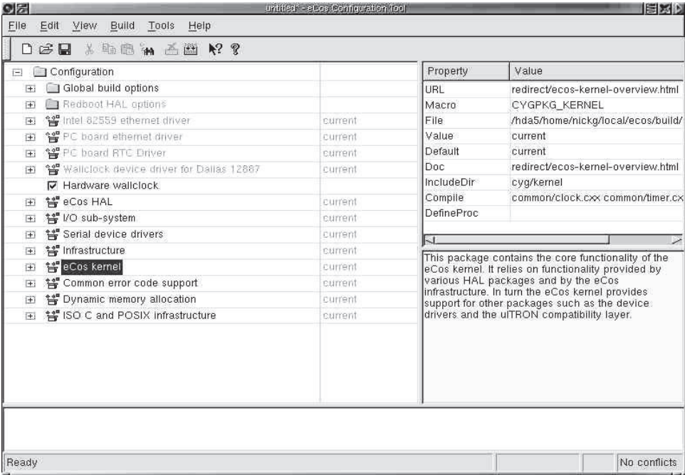
Рис. Р.1. Инструмент конфигурирования eCos: верхний уровень
