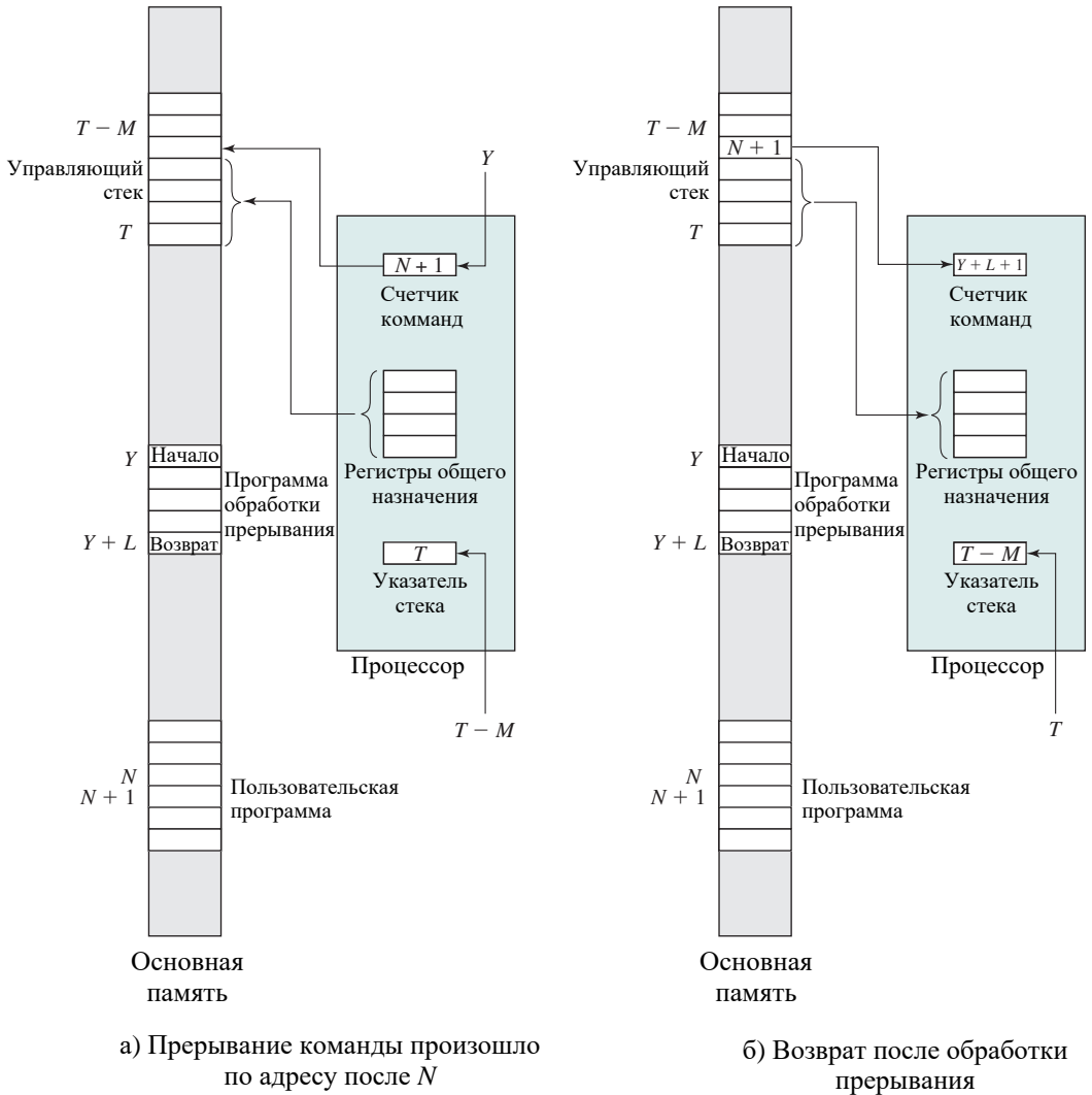
Рис. 1.11. Изменение памяти и регистров при обработке прерывания
