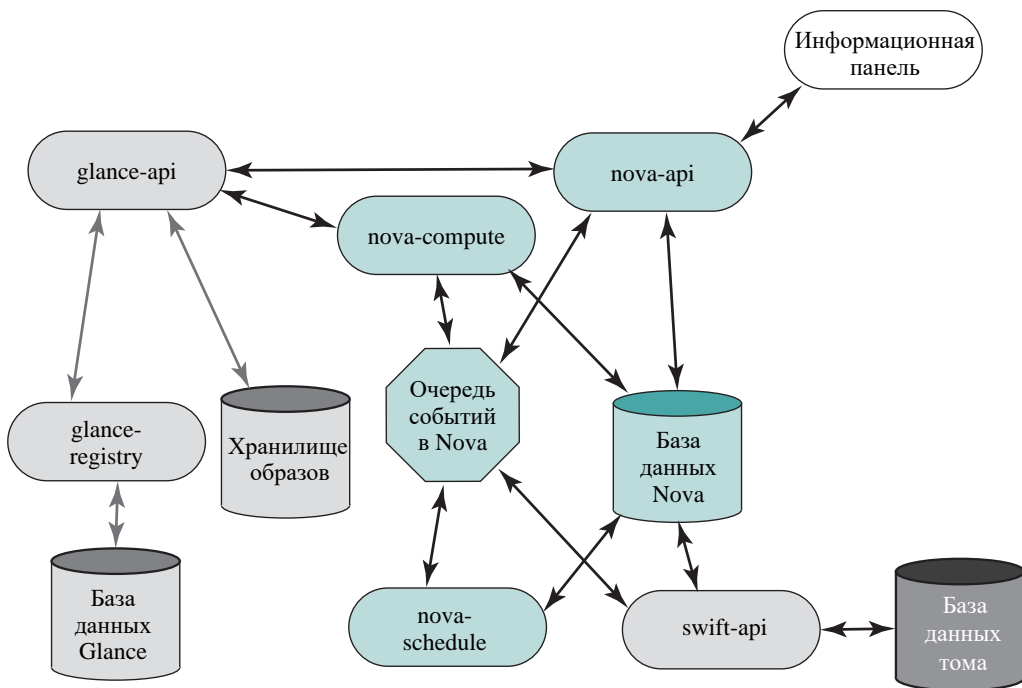
Рис. 16.10. Логическая архитектура компонента Nova
