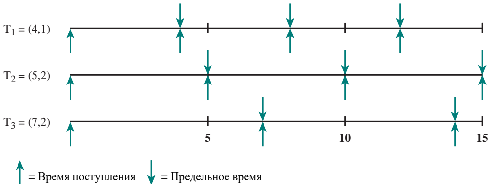
Рис. 10.7. Временная диаграмма периодического задания
