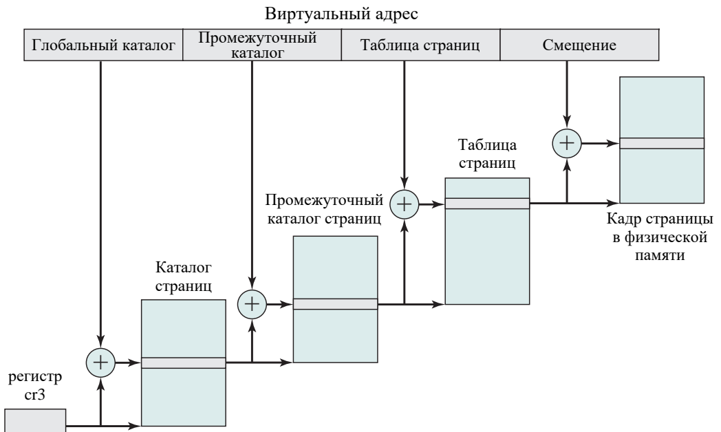
Рис. 8.23. Трансляция адреса в схеме виртуальной памяти Linux
