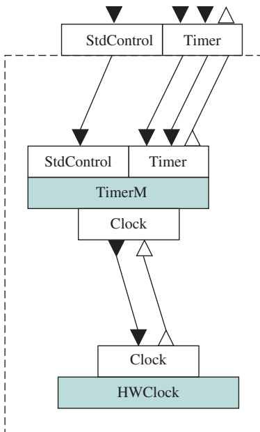
(b) Конфигурация TimerC
