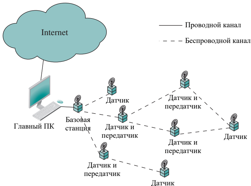
Рис. 13.8. Типичная топология сети беспроводных датчиков
