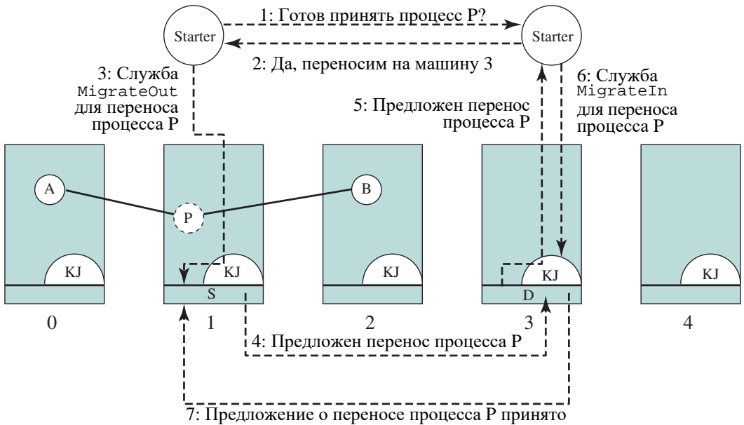
Рис. 19.2. Согласование переноса процессов
