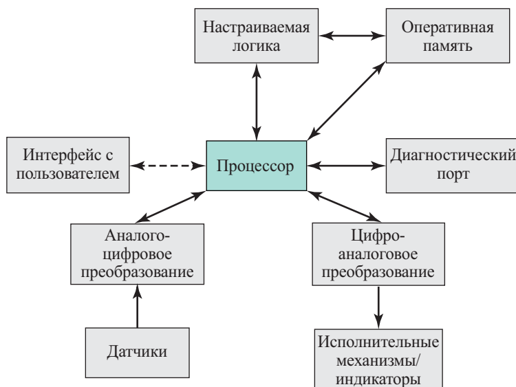
Рис. 13.1. Возможная организация встроенной системы
