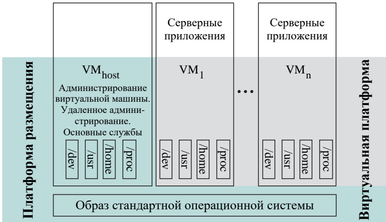
Рис. 14.12. Архитектура Linux VServer
