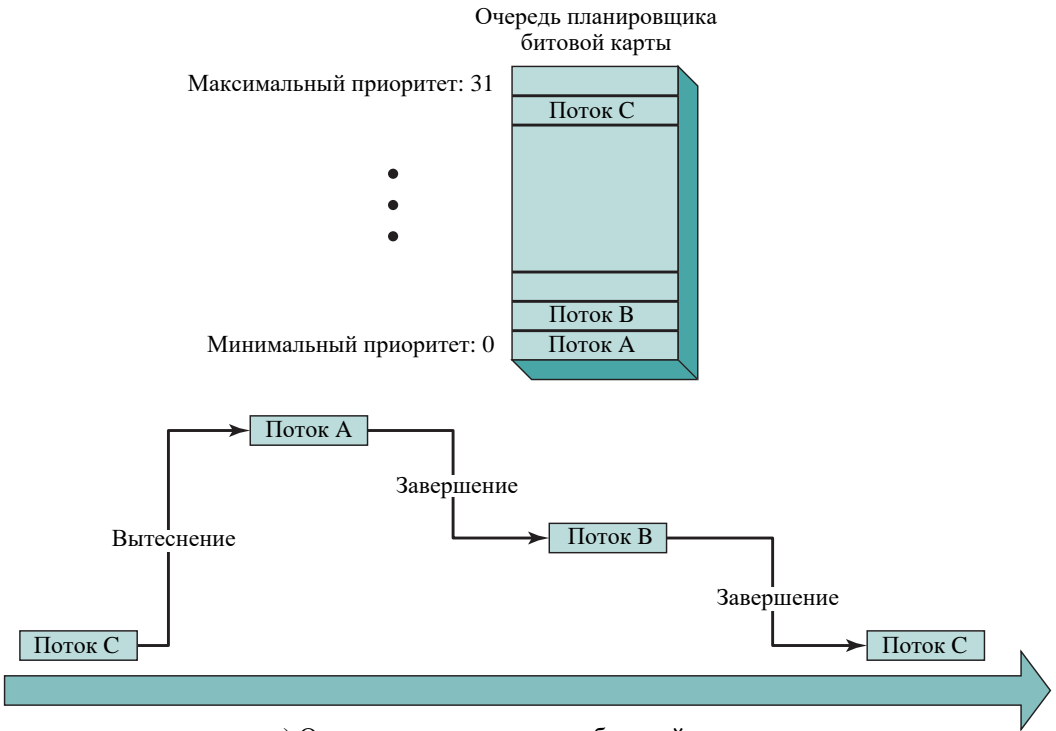
а) Операции планировщика битовой карты
