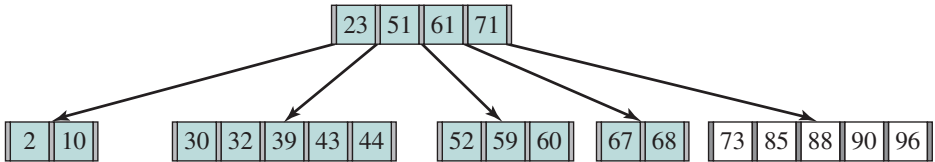
б) Вставлен ключ 90. Это простая вставка в узел
