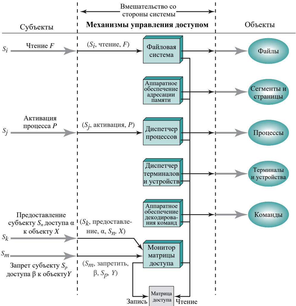
Рис. 15.5. Организация функционирования управления доступом
