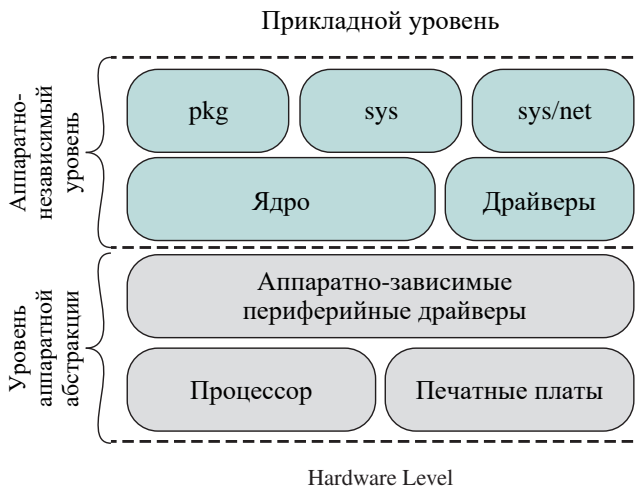
Рис. 16.14. Общая структура операционной системы RIOT
