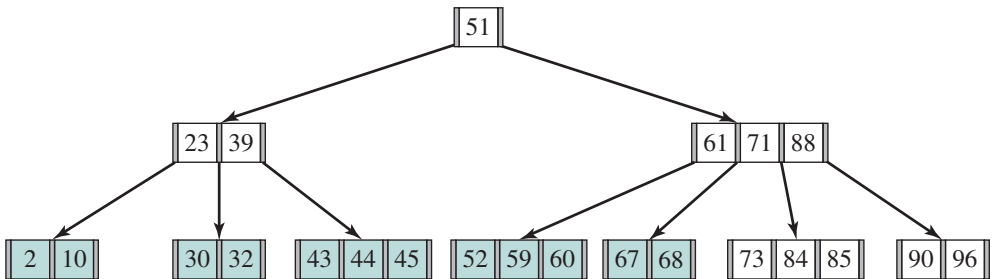
г) Вставлен ключ 84. Вставка требует разделения узла на две части и повышения одного ключа в корневой узел, что приводит к разделению корневой узла и созданию нового корня
