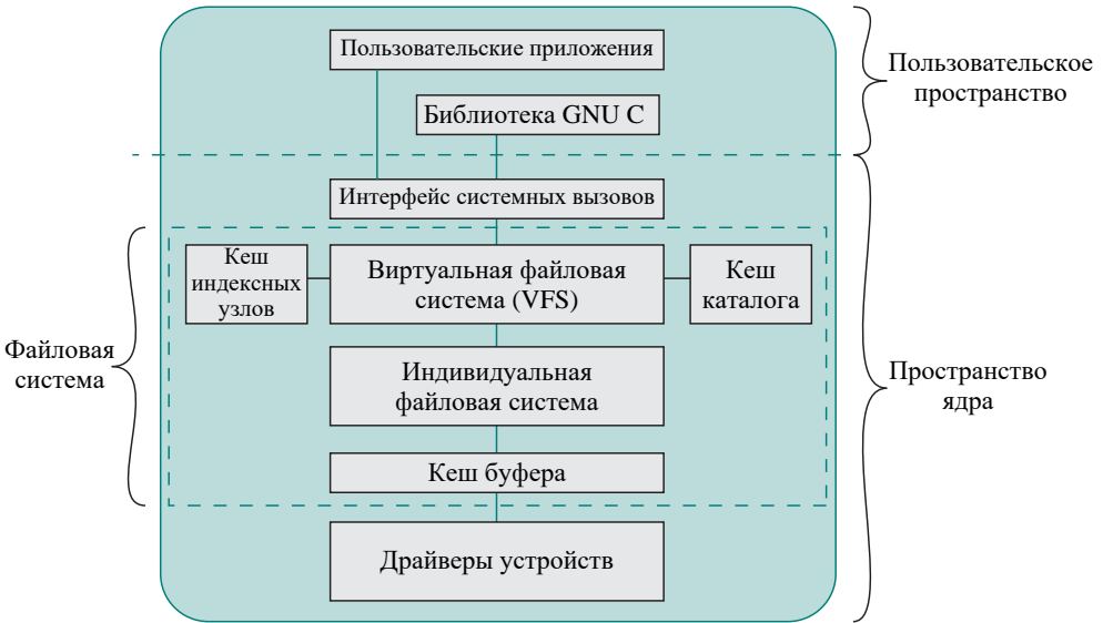
Рис. 12.17. Виртуальная файловая система Linux
