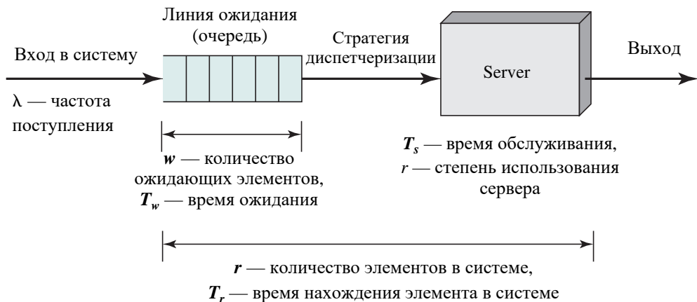
Рис. 3.2. Структура и параметры односерверной системы с очередью
