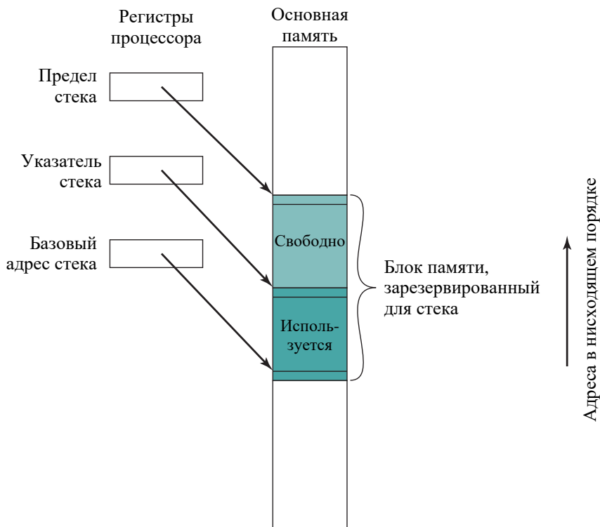
Рис. П.1. Типичная организация стека
