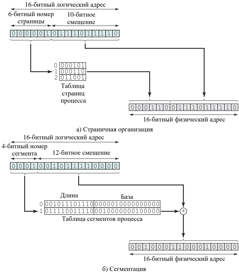
Рис. 7.12. Примеры трансляции логических адресов в физические
