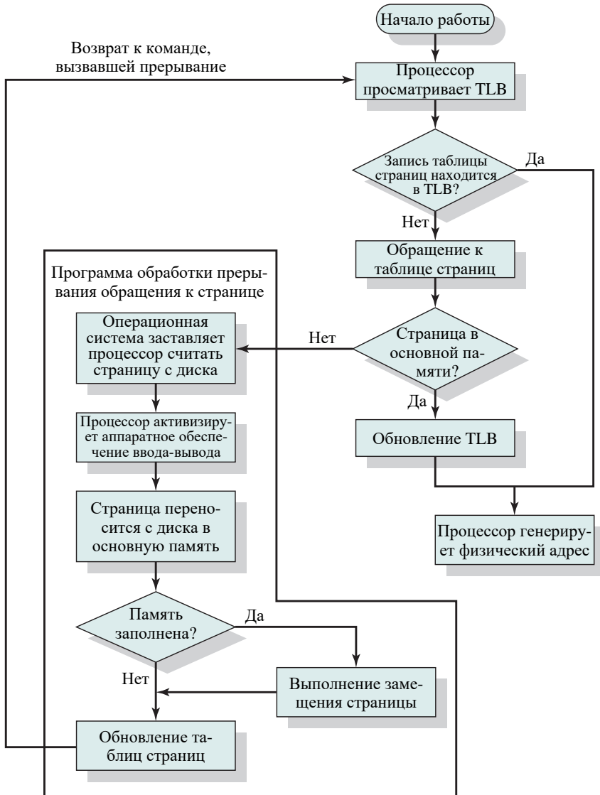
Рис. 8.7. Диаграмма трансляции адреса с использованием TLB
