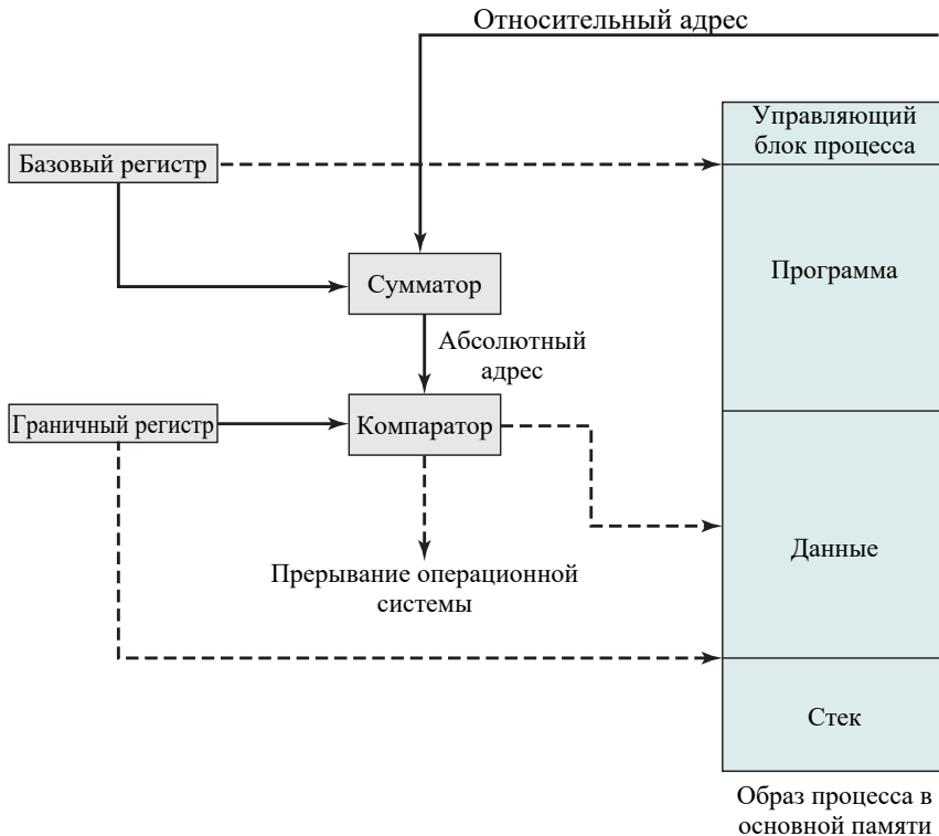
Рис. 7.8. Аппаратная поддержка перемещения
