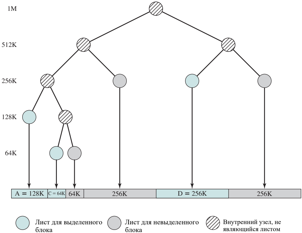
Рис. 7.7. Представление системы двойников в виде бинарного дерева
