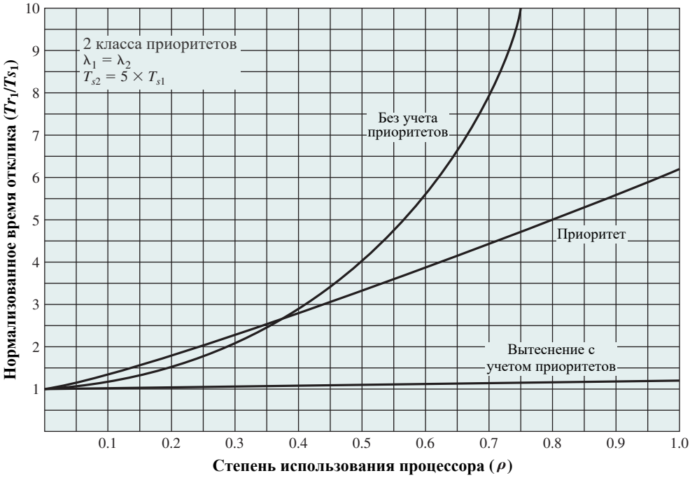
Рис. 9.12. Нормализованное время отклика для коротких процессов
