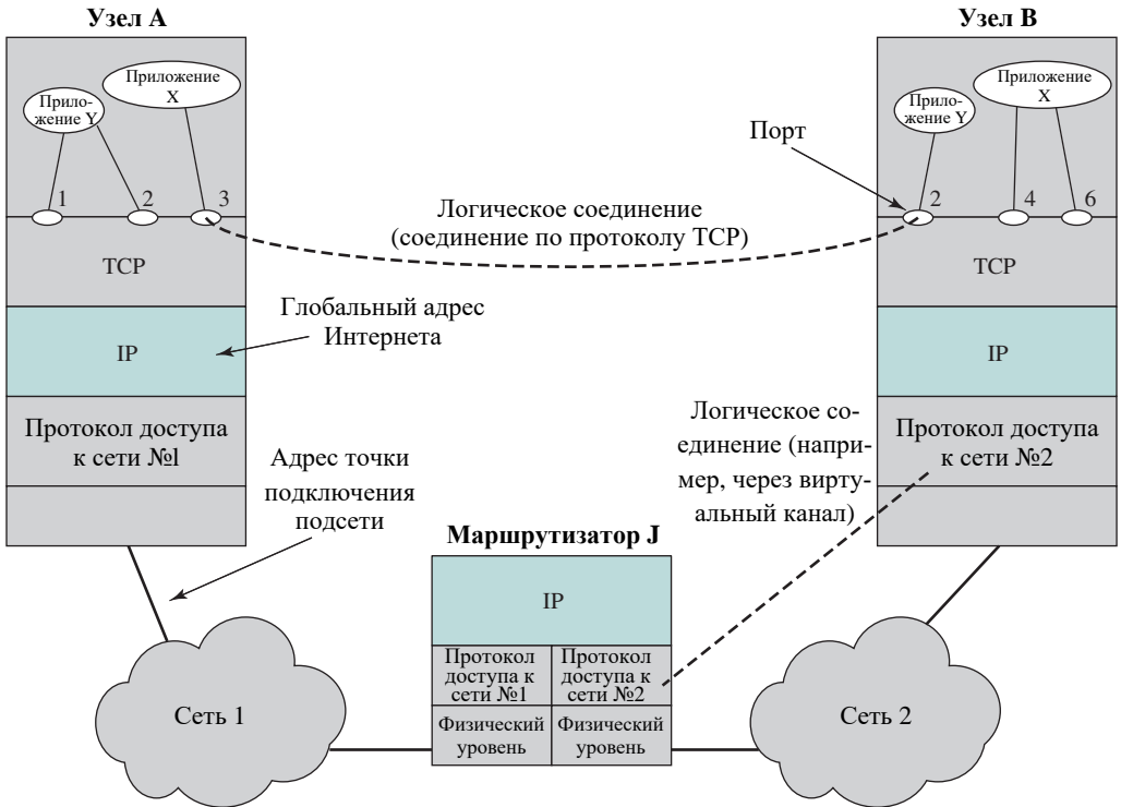
Рис. 17.4. Принципы действия протоколов TCP/IP
