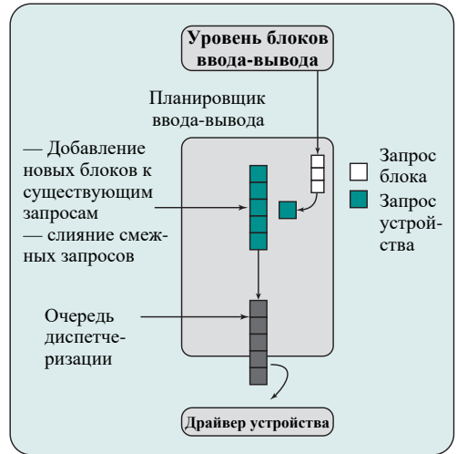
Планировщик NOOP
