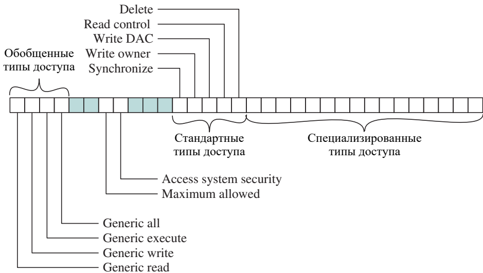
Рис. 15.10. Маски доступа
