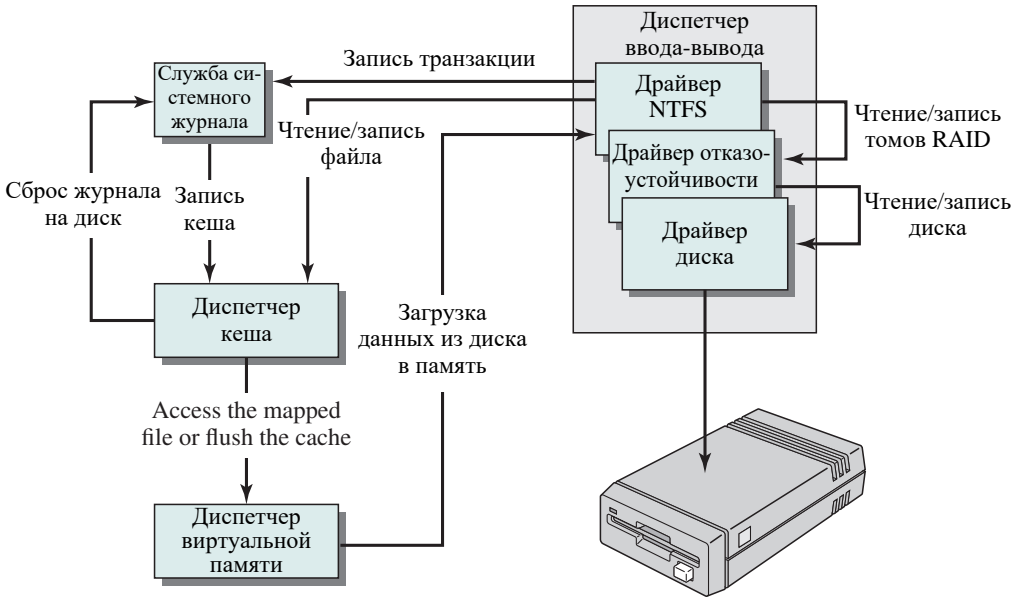
Рис. 12.20. Компоненты NTFS
