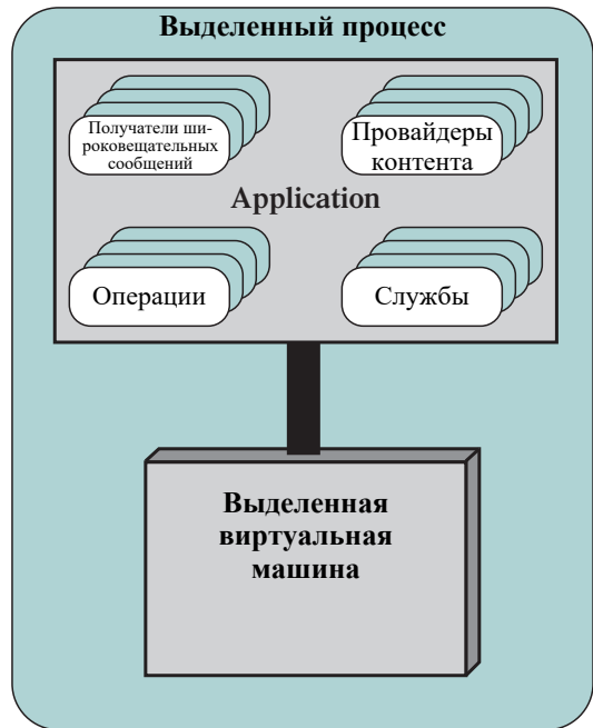
Рис. 4.16. Приложение Android
