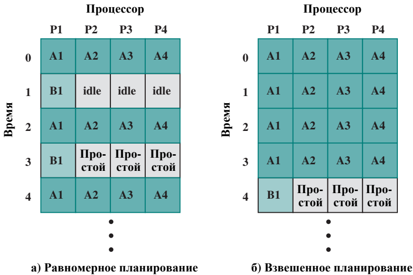
Рис. 10.2. Бригадное планирование
