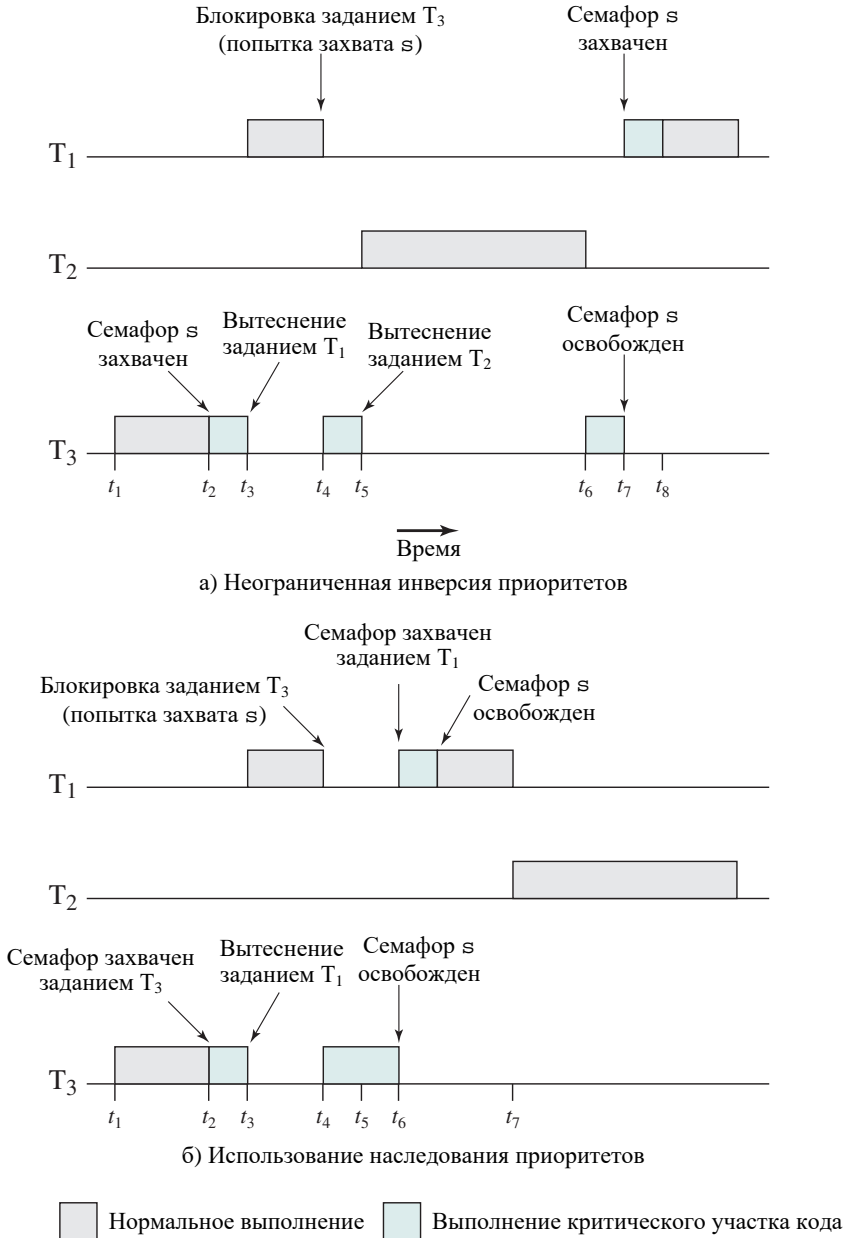
Рис. 10.9. Инверсия приоритетов
