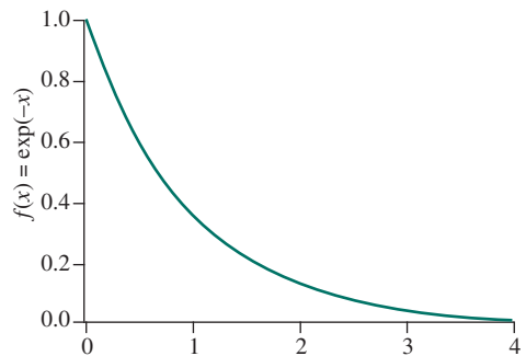
б) Плотность экспоненциального распределения вероятности ( \lambda = 1 )
