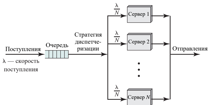
а) Многоканальная система массового обслуживания
