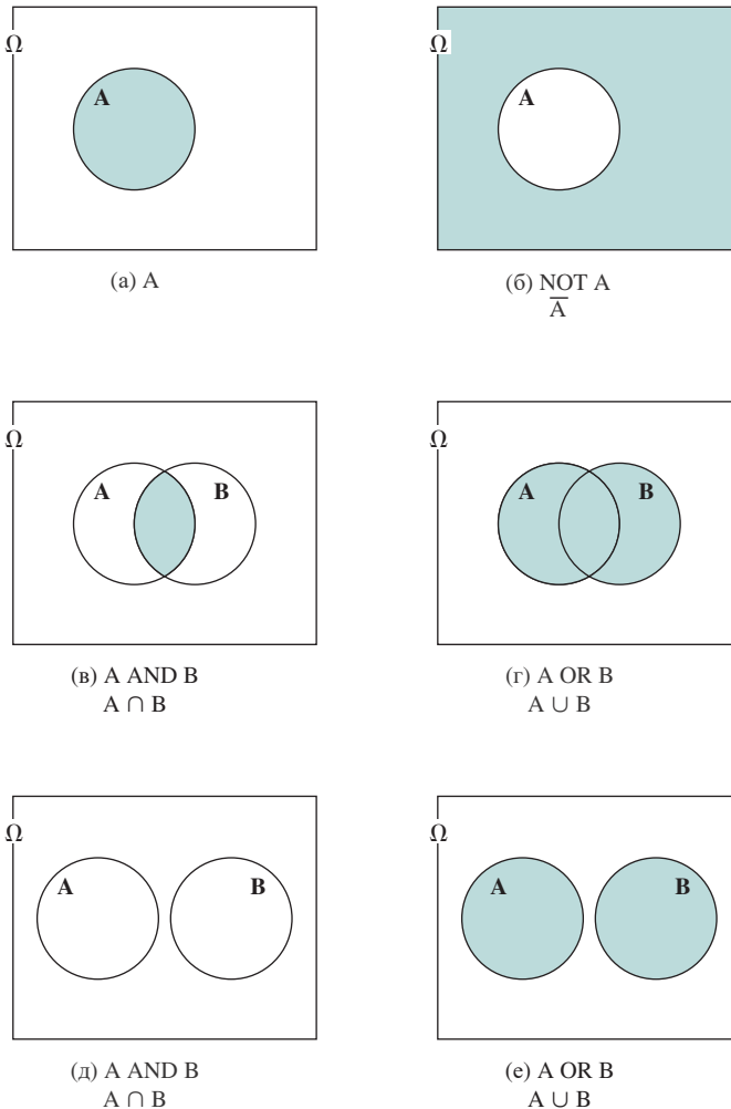
Рис. 20.1. Диаграммы Венна
