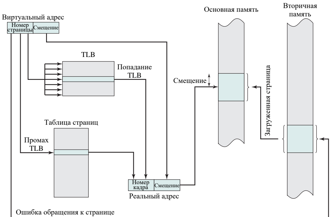
Рис. 8.6. Использование TLB
