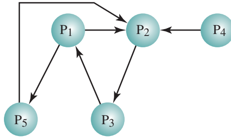
б) Взаимоблокировка
