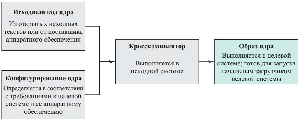
Рис. 13.5. Компиляция ядра
