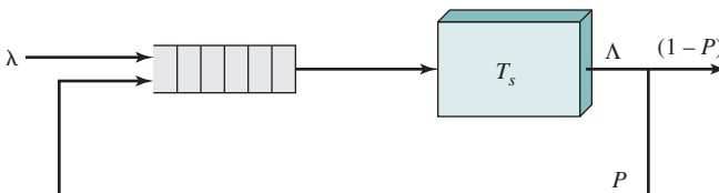
Рис. 21.11. Очередь с обратной связью
