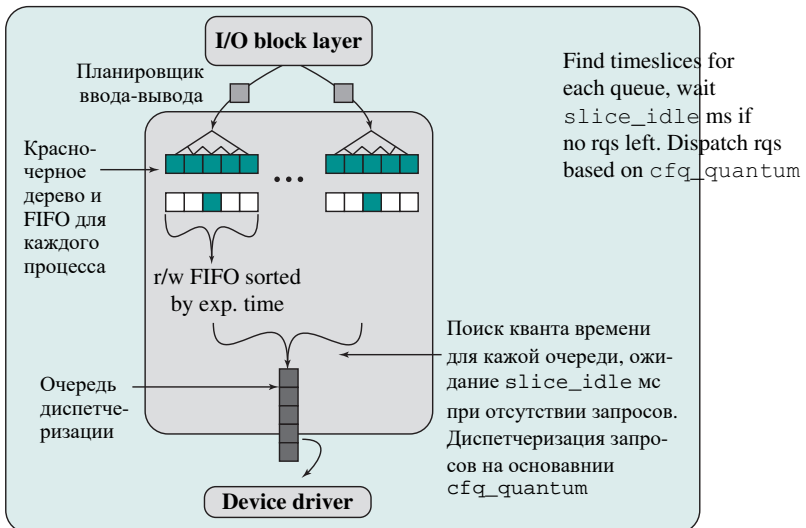
Планировщик CFQ
