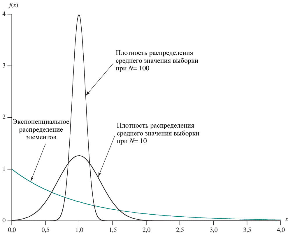
Рис. 21.9. Средние значения выборки для экспоненциального распределения
