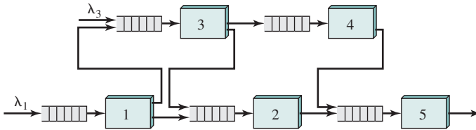
Рис. 21.7. Пример сети очередей
