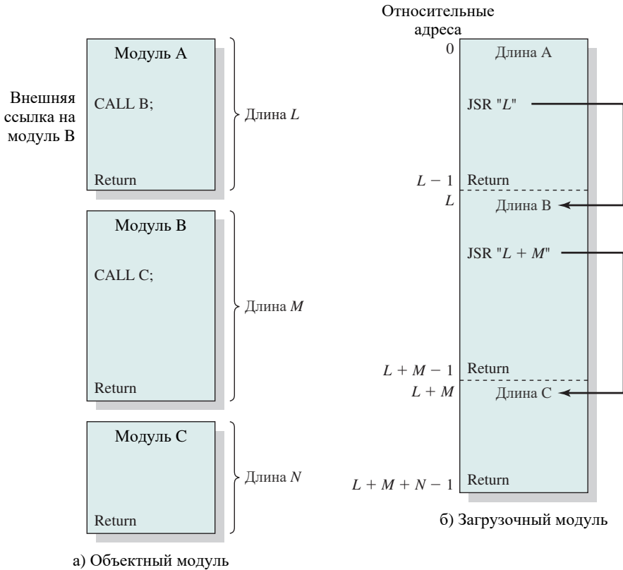
Рис. 7.16. Компоновка
