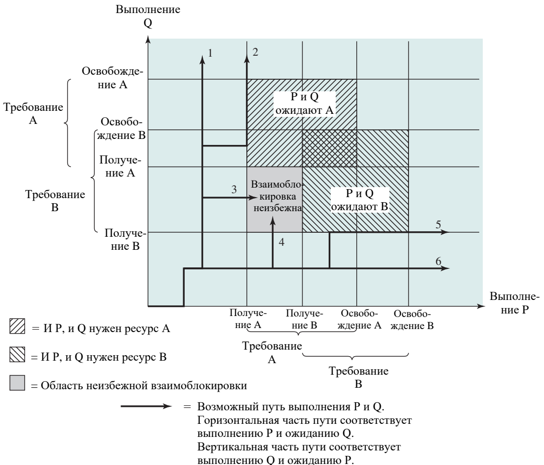
Рис. 6.2. Пример взаимоблокировки
