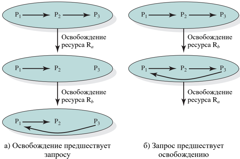
Рис. 19.12. Фантомная блокировка
