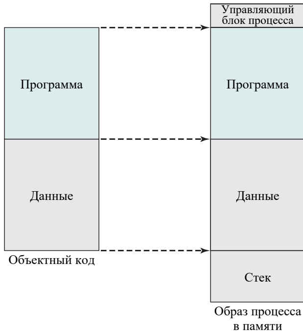
Рис. 7.13. Функция загрузки
