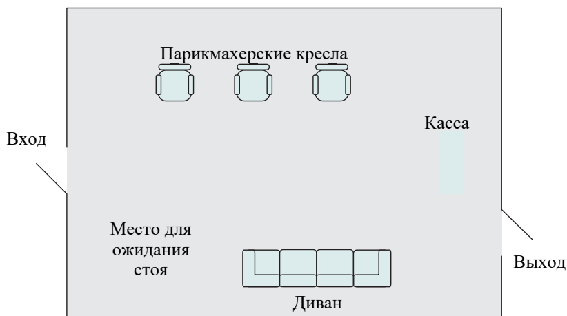
Рис. А.1. Парикмахерская
