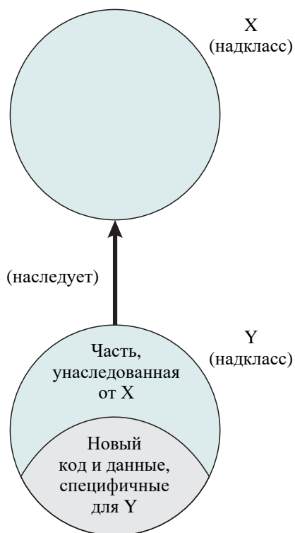
Рис. Г.3. Наследование
