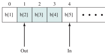
Рис. 5.11. Бесконечный буфер задачи “производитель/потребитель”
