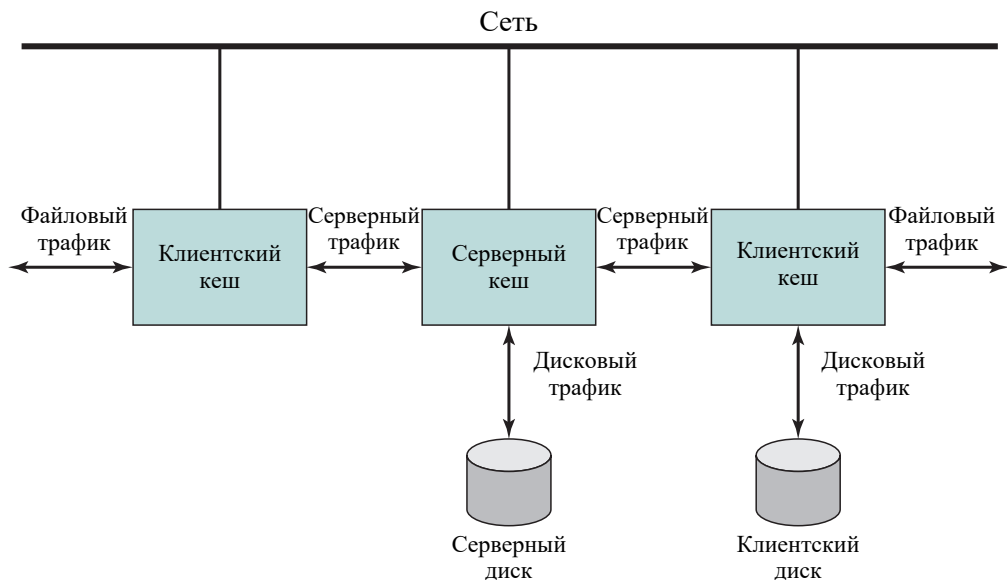
Рис. 18.7. Распределенное кеширование файлов в ОС Sprite
