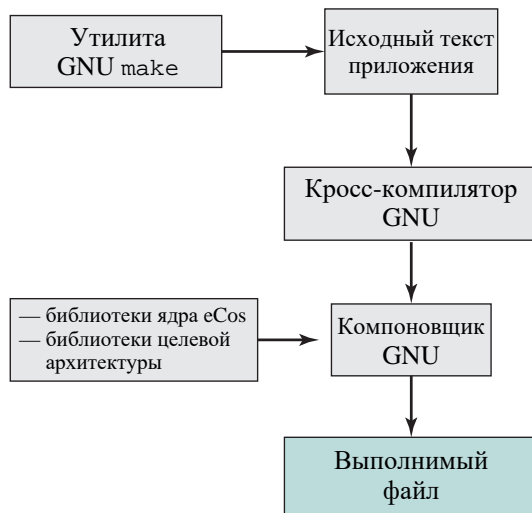
Рис. Р.3. Загрузка конфигурации eCos
