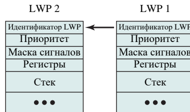
Рис. 4.13. Структура процесса в традиционном UNIX и в Solaris [154]
