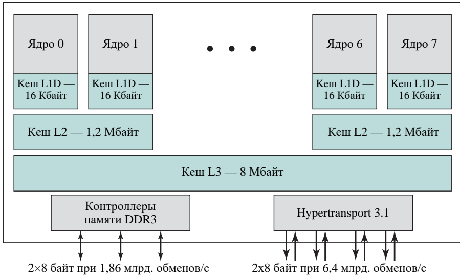
Рис. 10.3. Архитектура AMD Bulldozer
