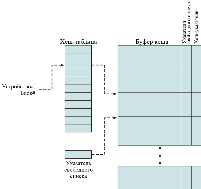
Рис. 11.13. Организация буфера кеша в UNIX
