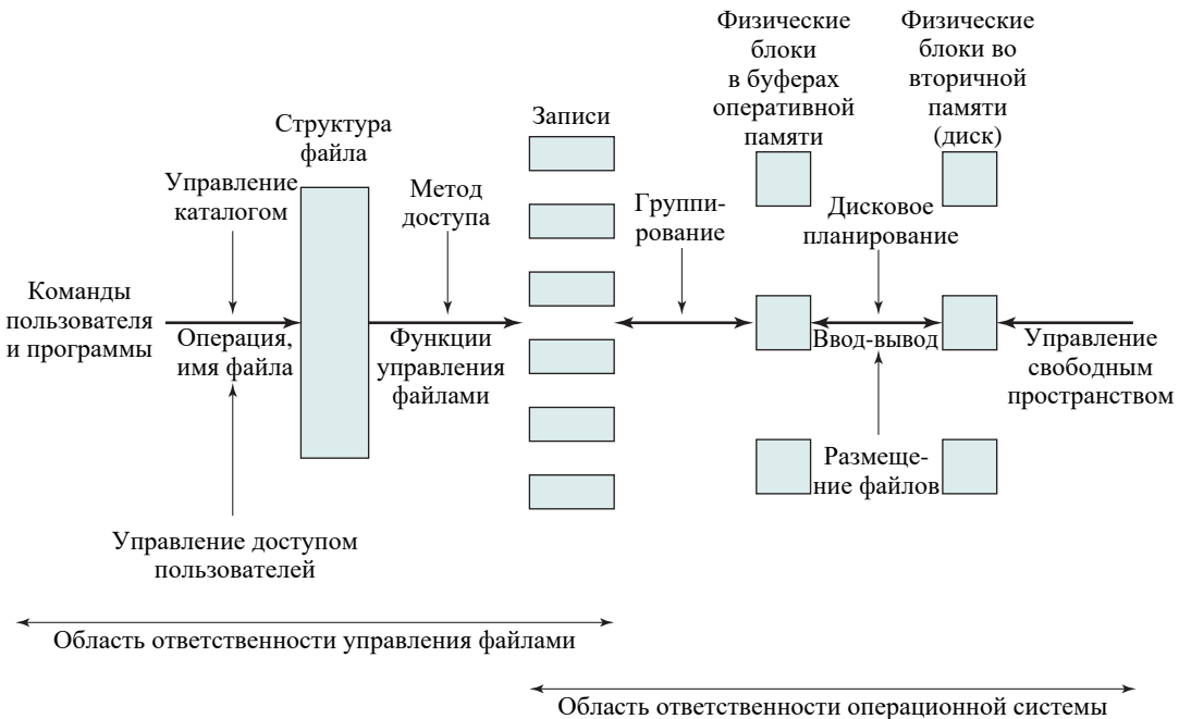
Рис. 12.2. Элементы управления файлами
