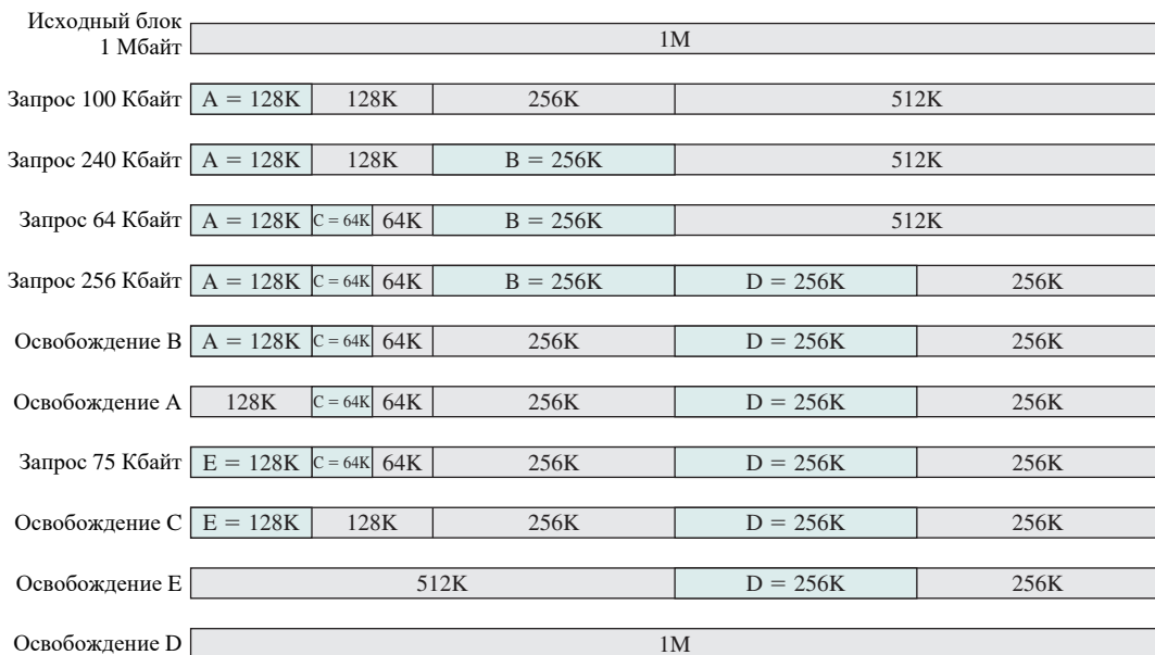
Рис. 7.6. Пример системы двойников
