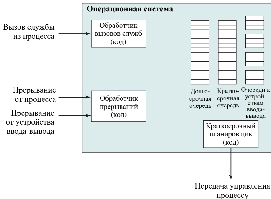
Рис. 2.11. Ключевые элементы многозадачной операционной системы
