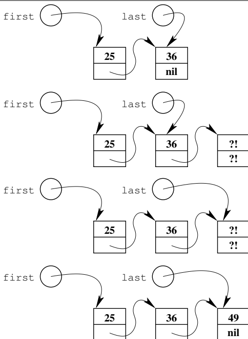
Рис. 2.10. Добавление нового элемента в конец списка
