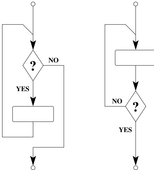
Рис. 2.2. Блок-схемы циклов с предусловием и постусловием
