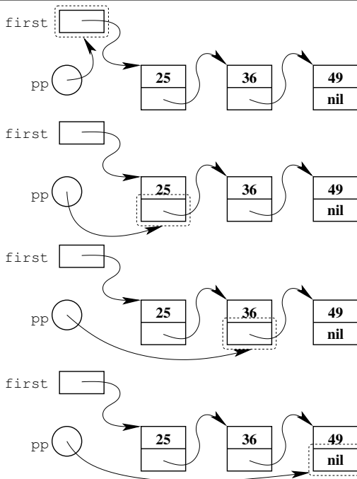
Рис. 2.11. Указатель на указатель в качестве переменной цикла
