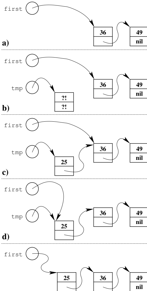
Рис. 2.7. Занесение нового элемента в начало односвязного списка
