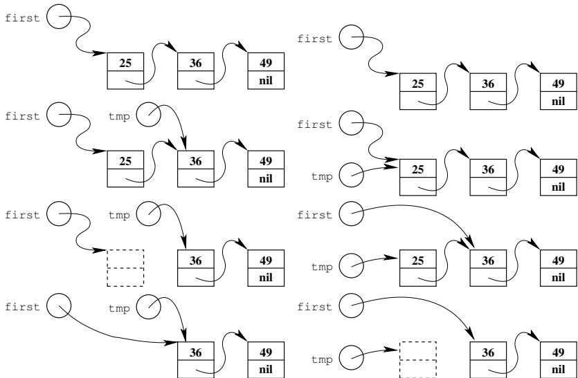
Рис. 2.9. Два способа удаления первого элемента односвязного списка
