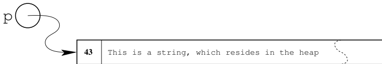
Рис. 2.4. Указатель на строку в динамической памяти
