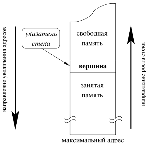
Рис. 3.4. Стек
