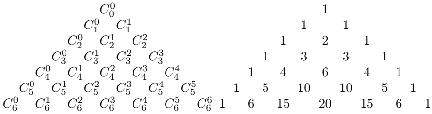
Рис. 1.9. Треугольник Паскаля
