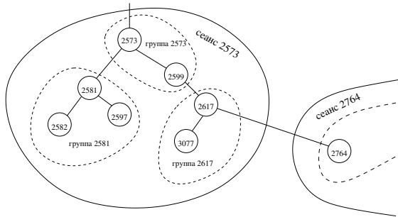
Рис. 5.9. Сеансы и группы процессов
