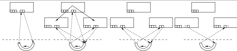
Рис. 5.5. Связывание двух процессов-потомков через именованный канал
