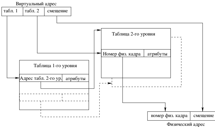
Рис. 8.8. Двухуровневая схема страничного преобразования
