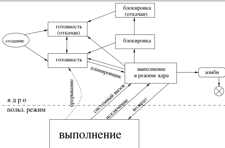
Рис. 8.2. Жизненный цикл процесса
