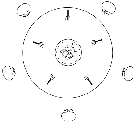
Рис. 7.6. Обедающие философы
