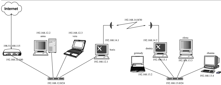
Рис. 6.5. Пример назначения ip-адресов
