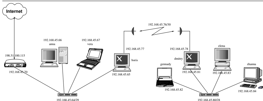
Рис. 6.6. Более компактное использование ip-адресов
