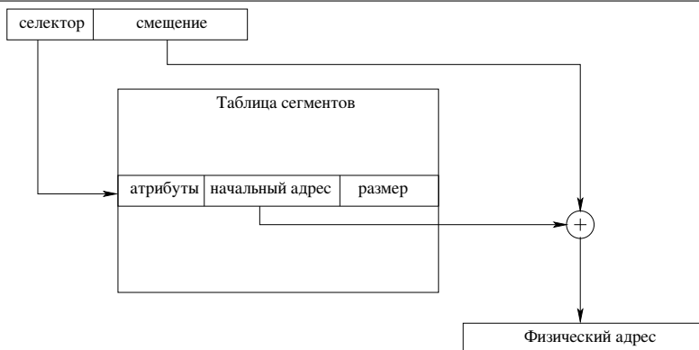
Рис. 8.5. Сегментная организация памяти
