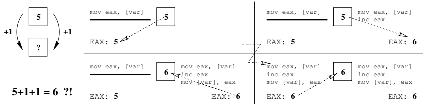
Рис. 7.1. Одновременное увеличение разделяемой переменной
