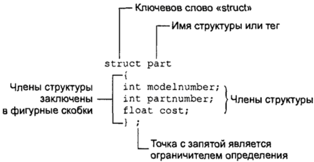
Рис. 4.1. Синтаксис определения структуры
