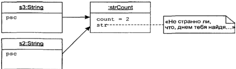
Рис. 11.8. Конструктор копирования в STRIMEM
