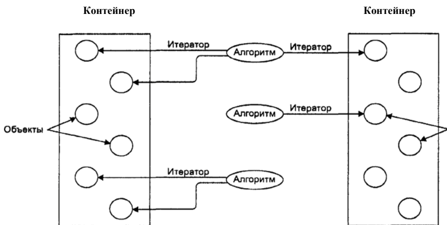
Алгоритмы используют итераторы для работы с объектами контейнеров.
