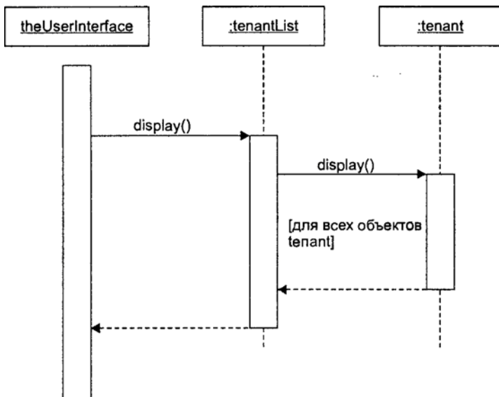
Рис. 16.12. Диаграмма последовательностей для варианта использования Вывод списка жильцов
