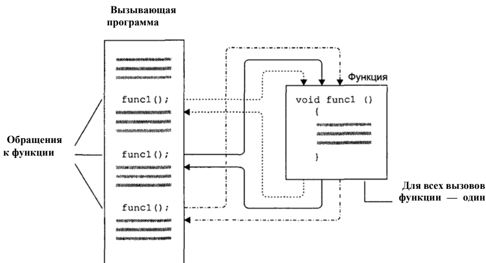
Рис. 5.1. Управление вызовами функции
