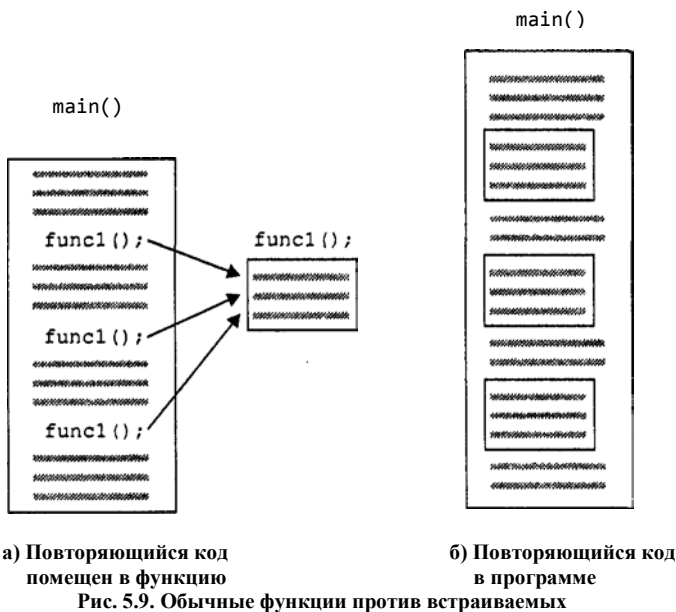
Рис. 5.9. Обычные функции против встраиваемых
