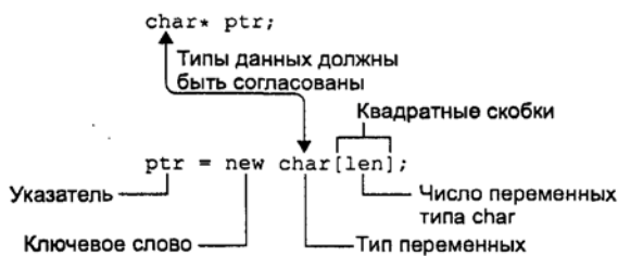
Рис. 10.13. Синтаксис операции new
