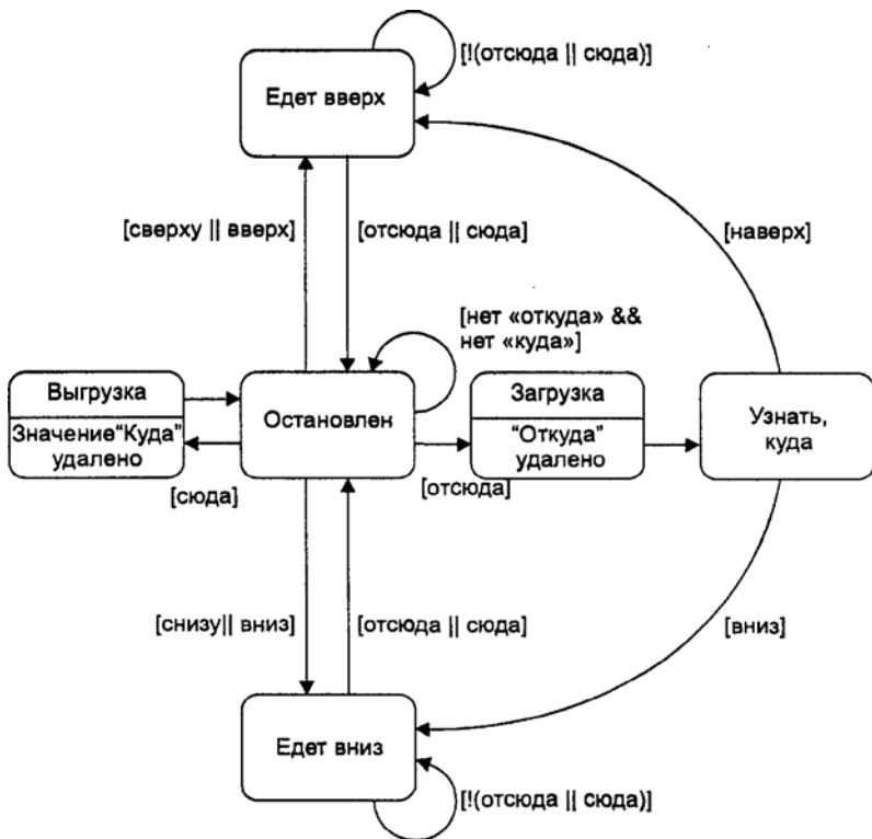
Рис. 13.6. Диаграмма состояний объекта elevator
