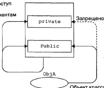
Рис. 9.3. Спецификаторы доступа в ситуации без наследования
