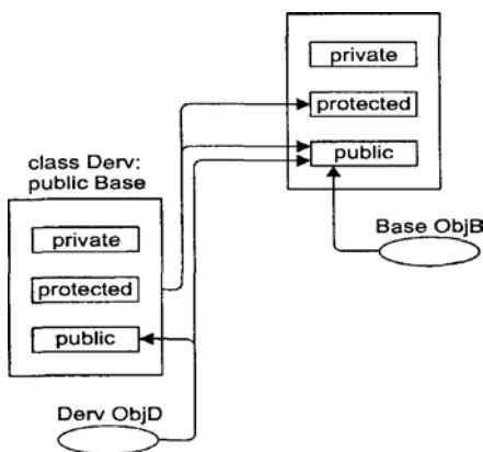
Рис. 9.4. Спецификаторы доступа в ситуации с наследованием
