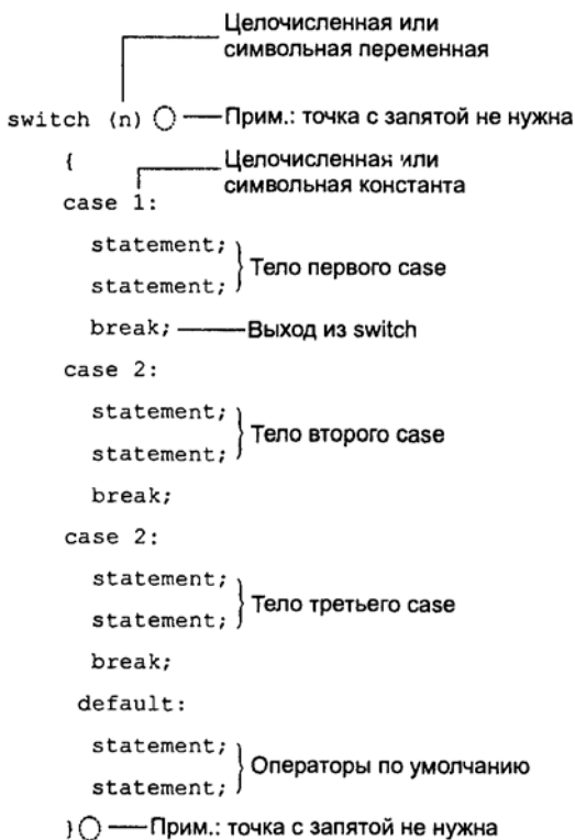
Рис. 3.12. Синтаксис оператора switch
