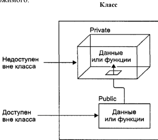
Рис. 6.2. Скрытые и общедоступные классы
