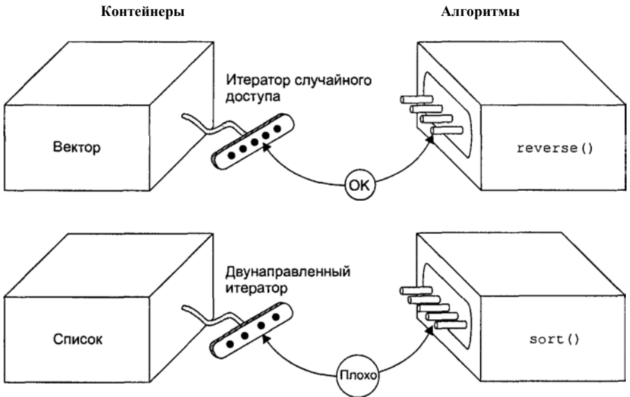
Рис. 15.4. Итераторы, соединяющие контейнеры и алгоритмы
