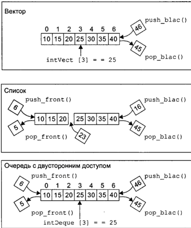
Рис. 15.2. Последовательные контейнеры
