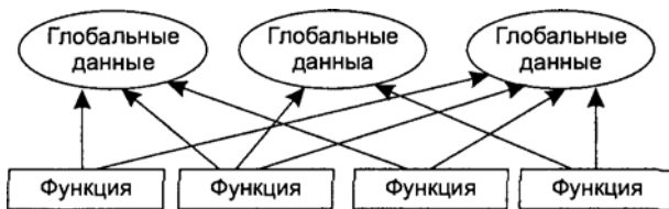
Рис. 1.2. Процедурный подход
