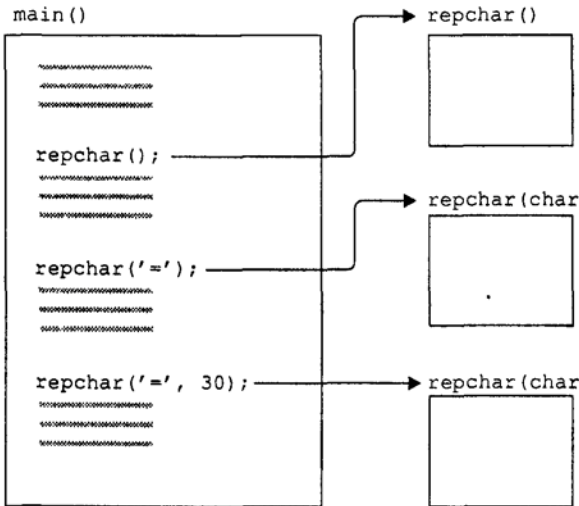
Рис. 5.8. Перегруженные функции
