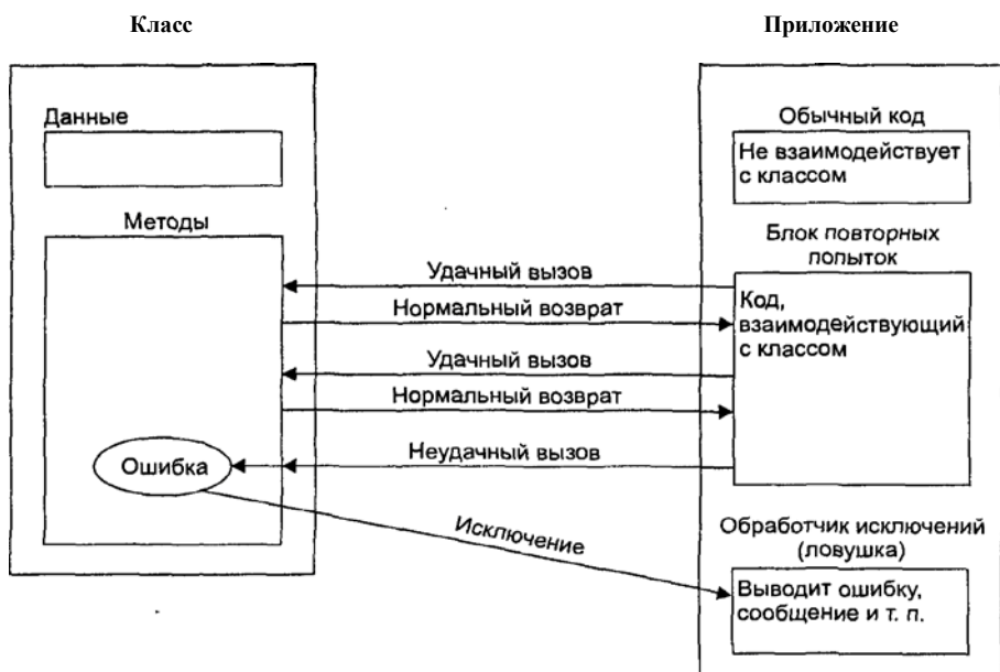
Рис. 14.4. Механизм исключений
