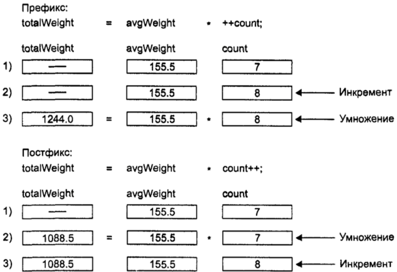
Рис. 2.11. Операция инкремента
