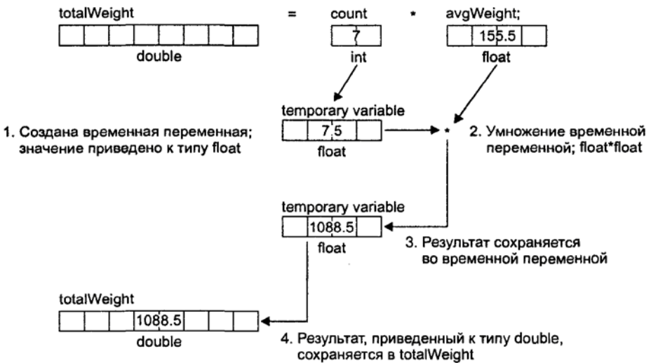
Рис. 2.9. Преобразования типов
