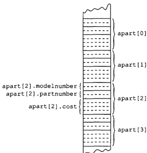
Рис. 7.5. Массив структур
