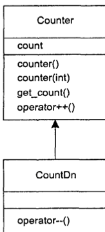
Рис. 9.2. Диаграмма классов UML для примера COUNTEN
