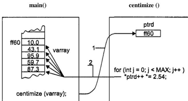
Рис. 10.7. Доступ к массиву из функции
