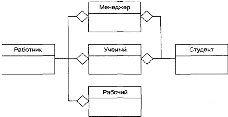
Рис. 9.12. Диаграмма классов UML для программы ЕРМCONT
