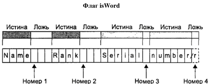
Рис. 4.10. Работа программы WDCOUNT
