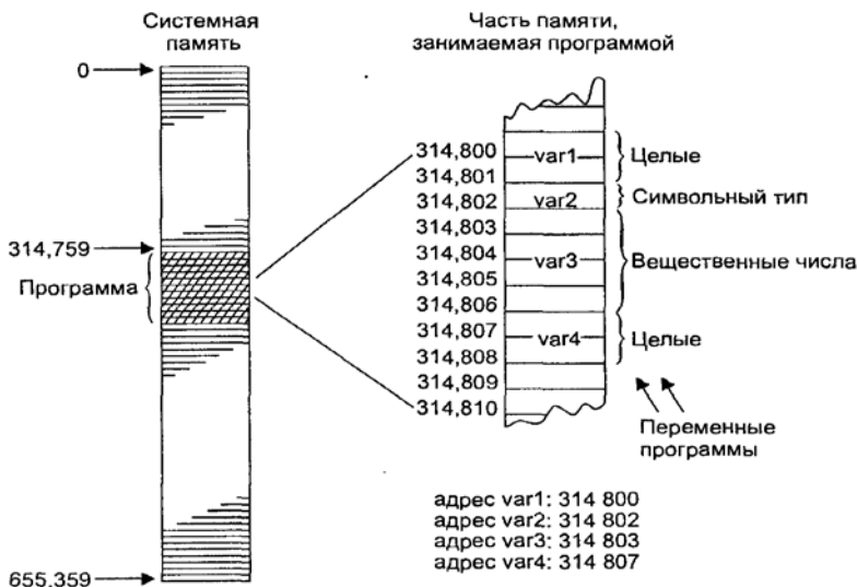
Рис. 10.1. Адреса в памяти
