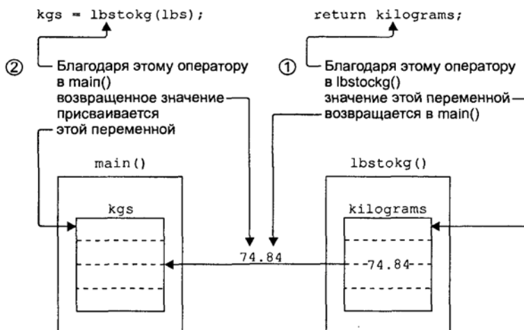
Рис. 5.6. Возврат значения
