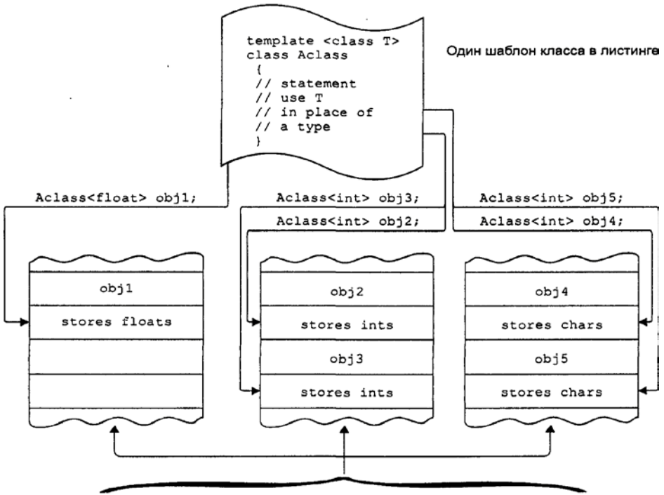
Рис. 14.2. Шаблон класса
