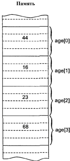
Рис. 7.2. Элементы массива
