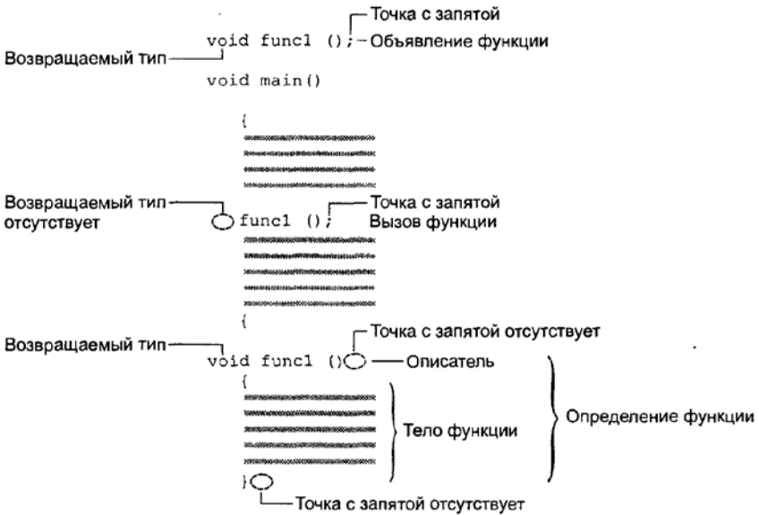
Рис. 5.2. Синтаксис функции
