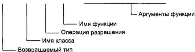
Рис. 6.5. Операция разрешения
