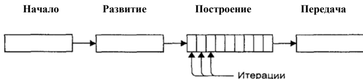
Рис. 16.2. Унифицированный процесс
