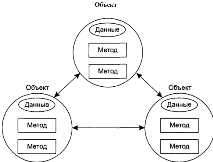
Рис. 1.3. Объектно-ориентированный подход
