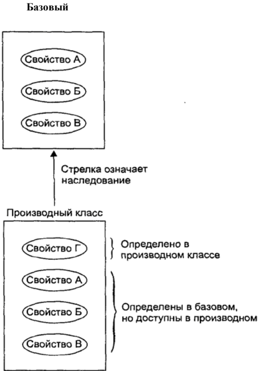
Рис. 9.1. Наследование
