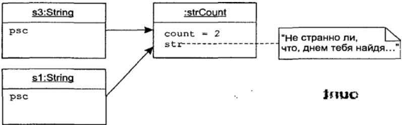
Рис. 11.7. Оператор присваивания в STRIMEM
