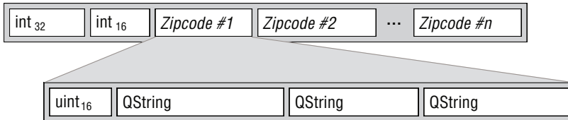
Рис. 3.4. Формат файла почтовых индексов
