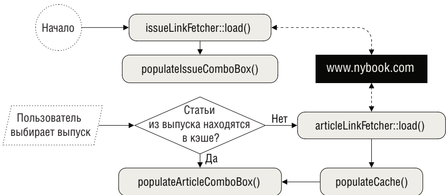
Рис. 1.10. Блок-схема приложения The New York Review of Books Viewer
