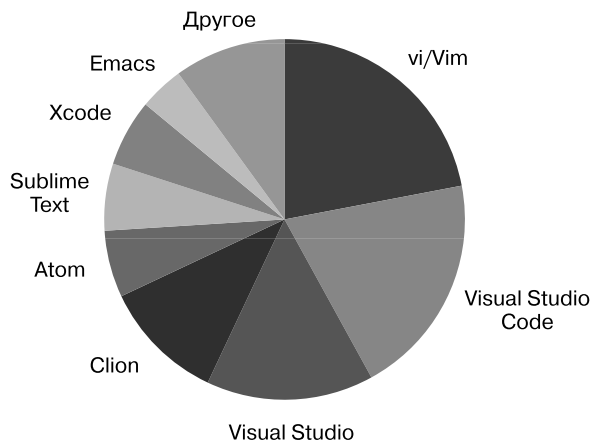
Рис. 1.1. Использование IDE/редакторов
