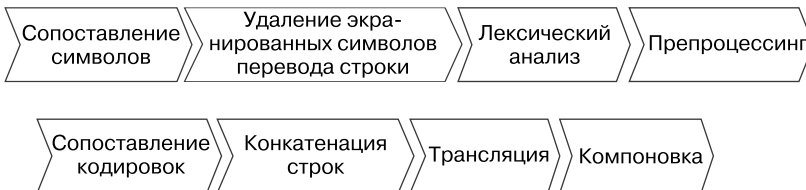
Рис. 9.1. Этапы компиляции
