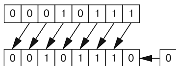
Рис. 4.1. Логический сдвиг влево на один бит
