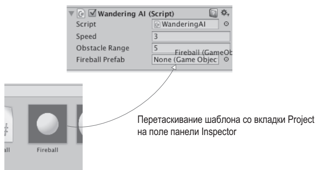
Рис. 3.11. Соединение огненного шара со сценарием
