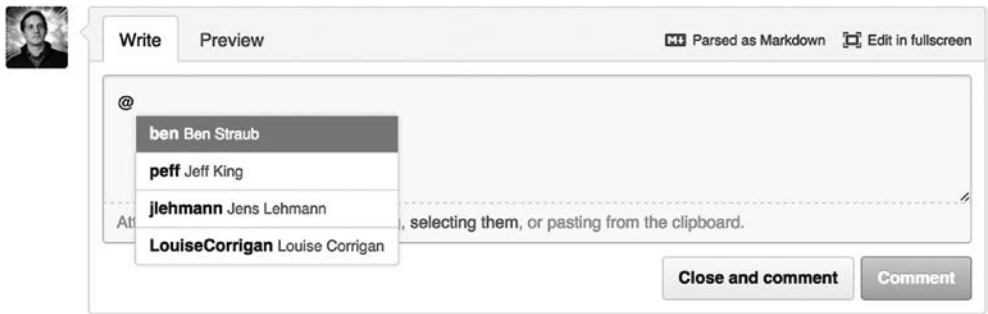
Рис. 6.38. Наберите символ @, чтобы упомянуть конкретного пользователя
