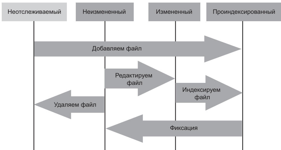
Рис. 2.1. Жизненный цикл состояния файлов
