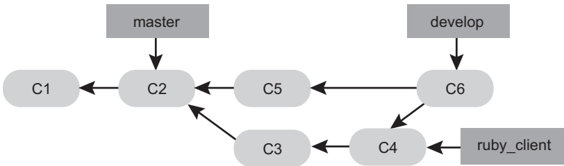
Рис. 5.23. После слияния с тематической веткой
