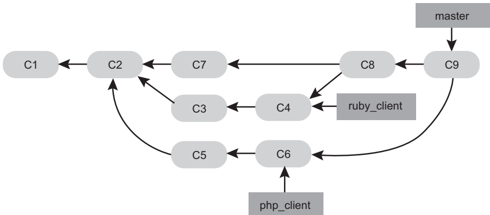
Рис. 5.21. Вид после слияния тематических веток
