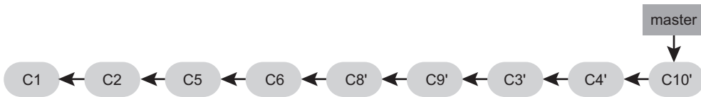
Рис. 3.35. Окончательный вид истории коммитов
