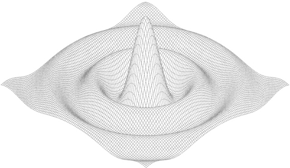
Рис. 3.1. Чертеж поверхности функции \sin(r)/r
