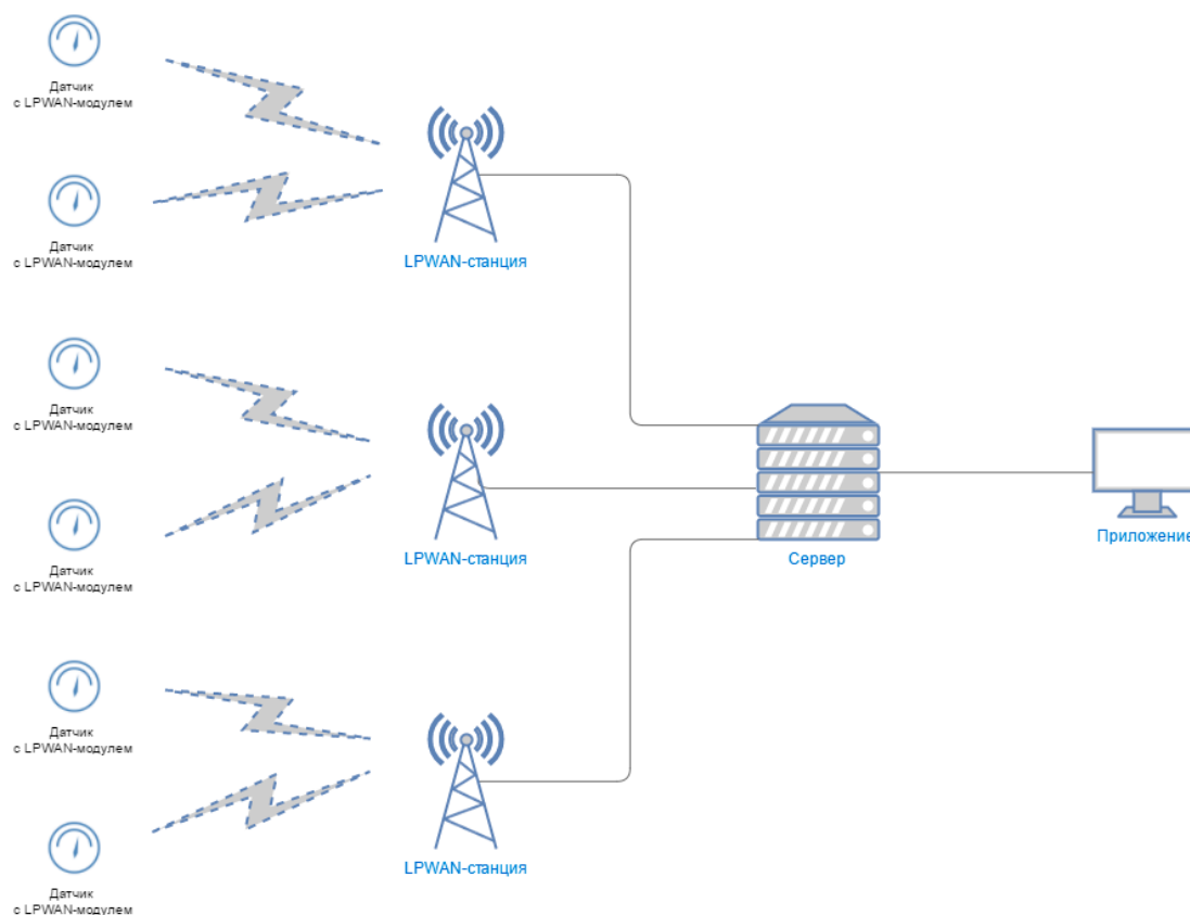
Рис. 24 – Топология LPWAN-сетей
