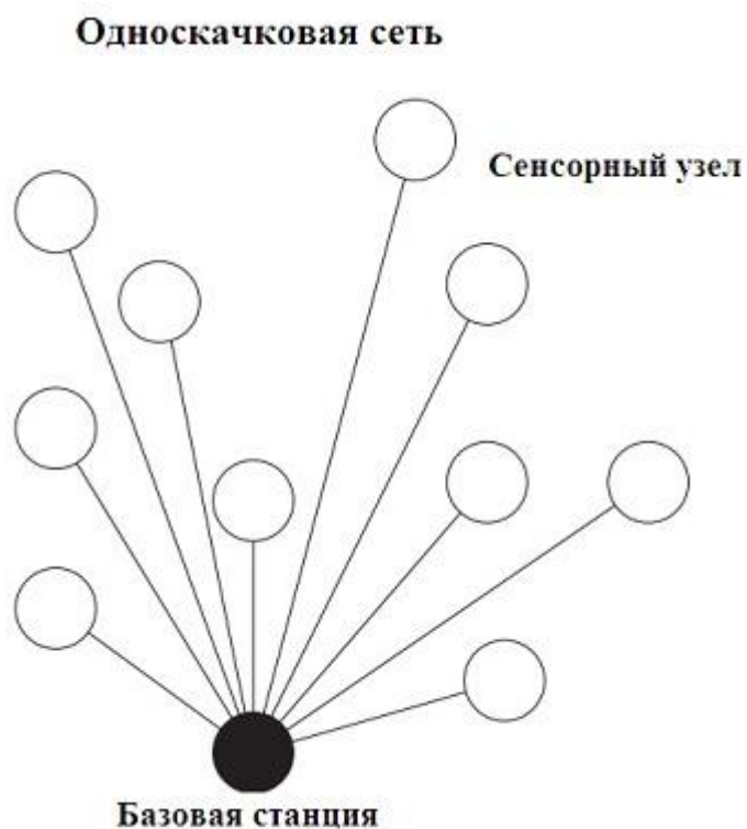
Рис.20 – Схема односкачковой сенсорной сети
