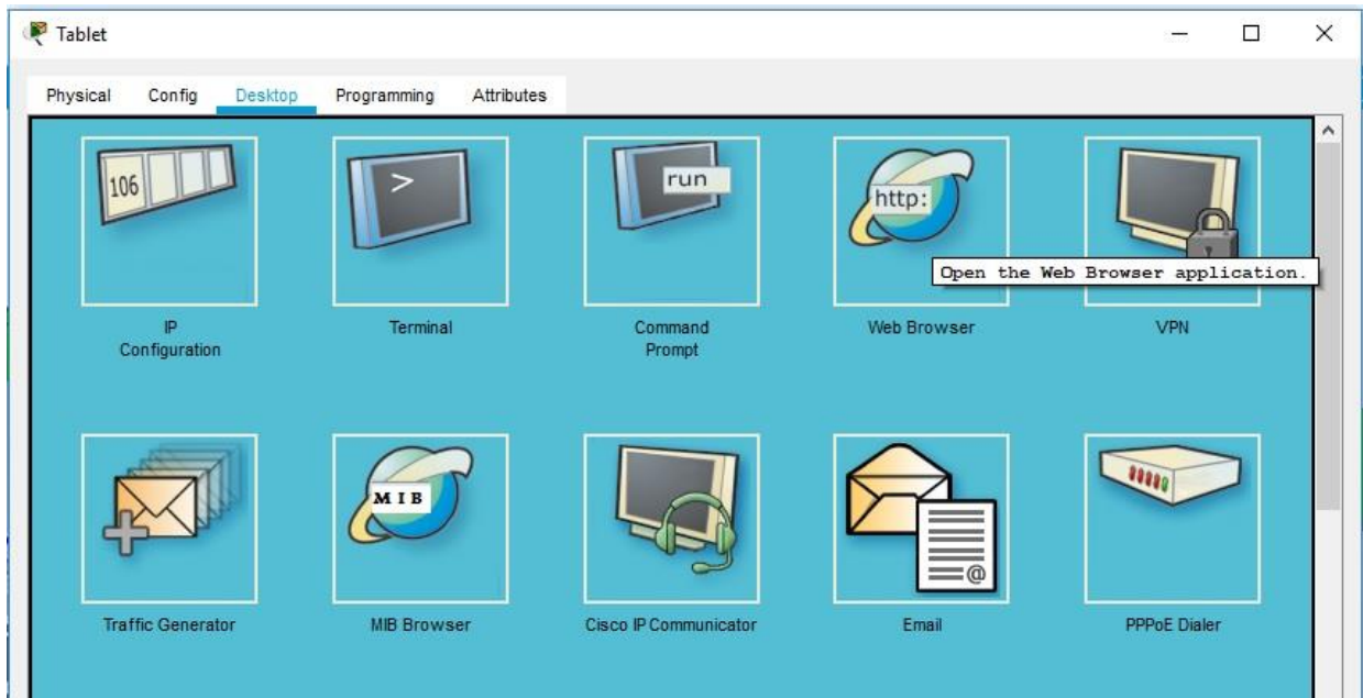
Рис. 33 – вкладка Desktop
