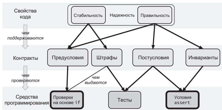
Рис. 6.1. Отношения между атрибутами надежности, спецификациями на базе контрактов и средствами программирования
