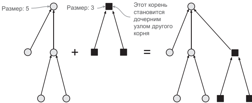
Рис. 3.7. Слияние двух деревьев в соответствии с политикой связывания по размеру. Меньшее дерево присоединяется к корню большего дерева
