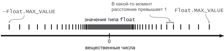
Рис. 4.9. Отношения между вещественными числами и значениями типа float
