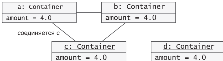
Рис. 2.6. Диаграмма объектов UML для Reference (абстрактная версия)
