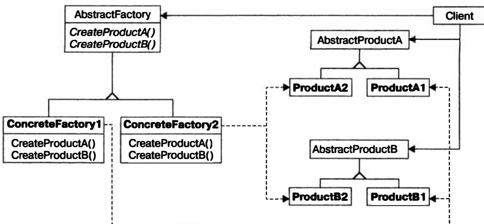
Рис. 6.2. Вы можете использовать паттерн «Абстрактная фабрика» для группировки существующих фабрик и инкапсуляции того, как вы к ним обращаетесь
