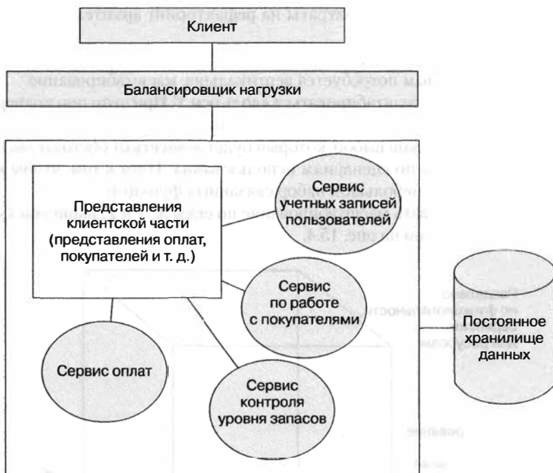
Рис. 15.3. Монолитная архитектура
