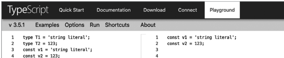
Рис. 2.9. Песочница TypeScript демонстрирует сгенерированный JavaScript-код. Символы на первых двух строках удаляются, следовательно, они относились к пространству типов
