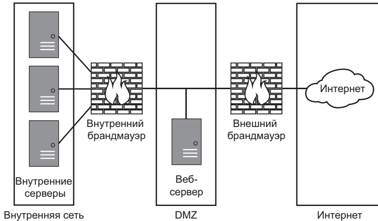
Рис. 10.2. DMZ
