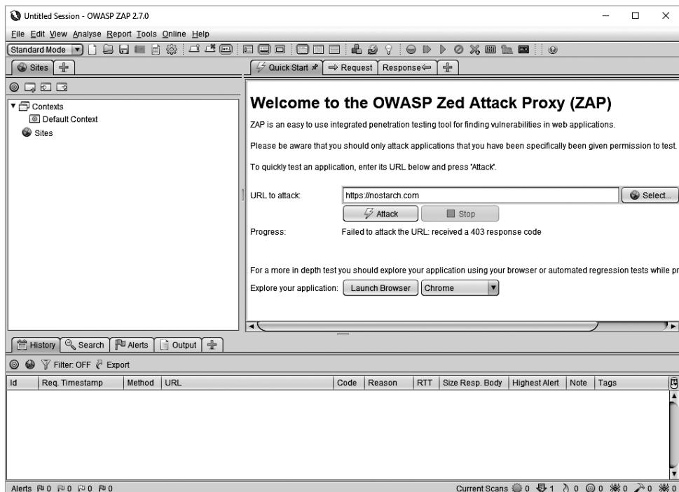
Рис. 13.5. ZAP
