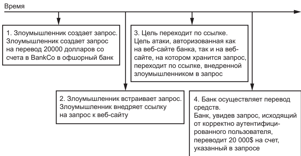
Рис. 3.4. Пример CSRF-атаки
