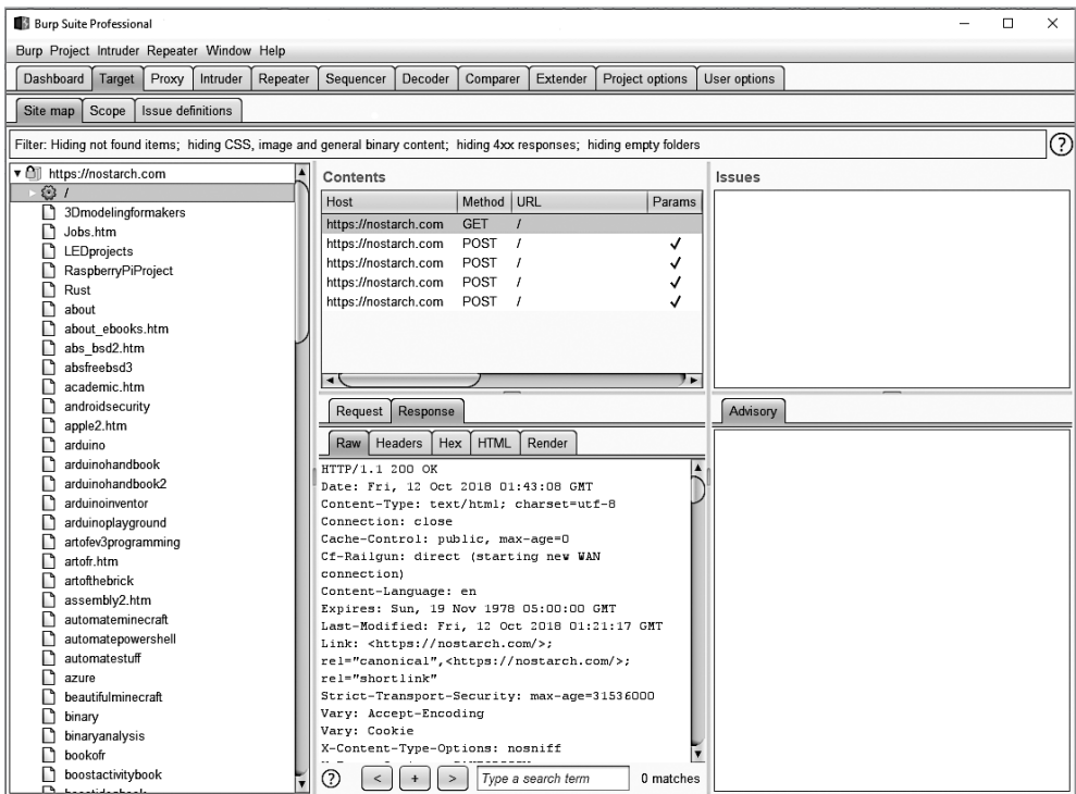
Рис. 13.6. Burp Suite
