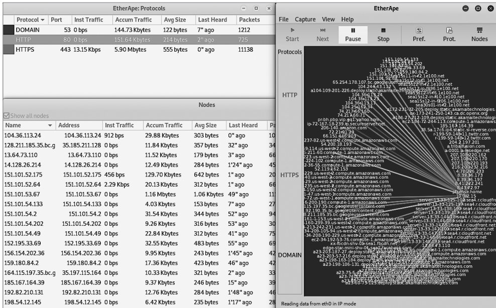
Рис. 13.4. EtherApe
