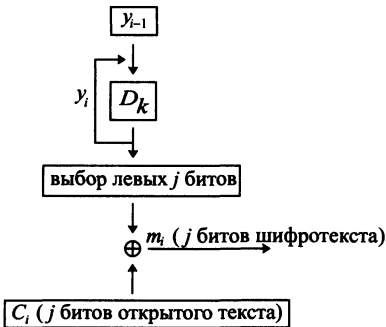
Рис. 5.13. Расшифрование в режиме OFB
