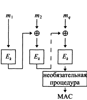
Рис. 5.15. Схема работы СВС-MAC
