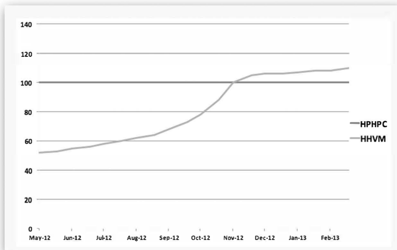
Рис. 12.1. Сравнение производительности HHVM с производительностью HHPC
