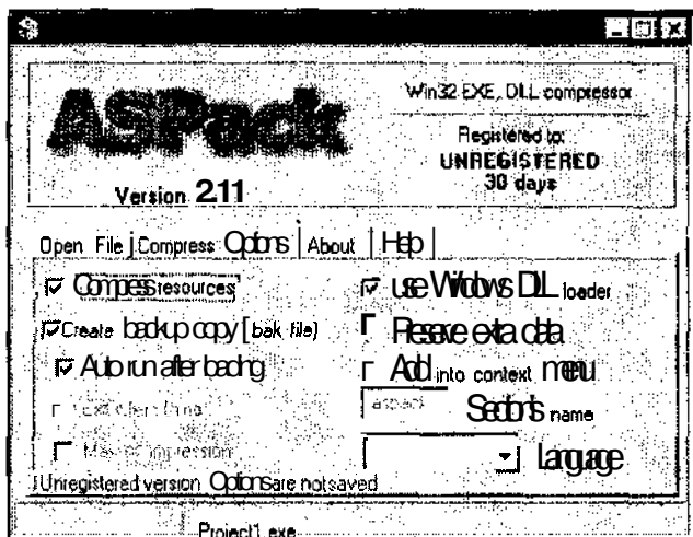
Рис. 1.3. Настройки ASPack
