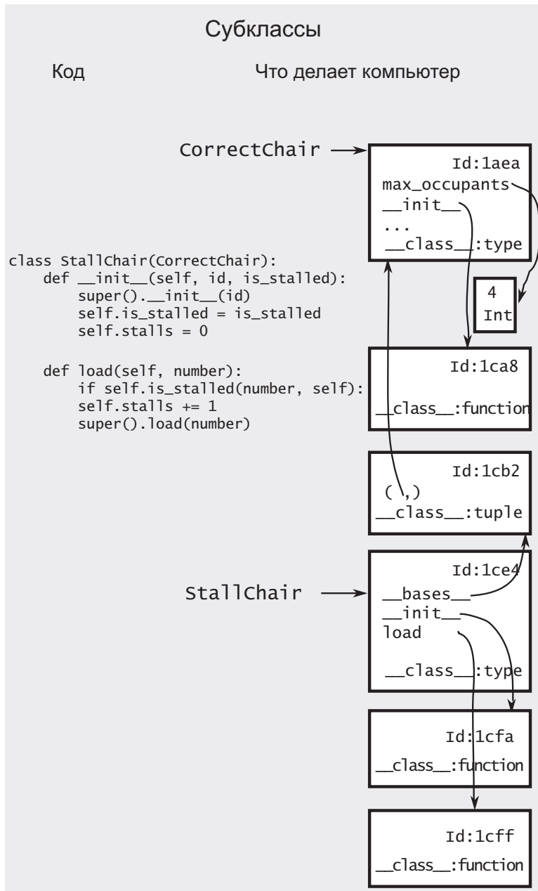
Рис. 22.3. Код создания subclasses с измененными методами. Обратите внимание на использование super() для вызова метода родительского класса. Диаграмма показывает, какие объекты создаются при создании класса, который является subclassом
