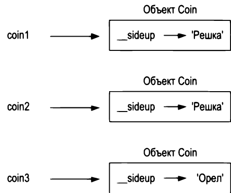
РИС. 10.9. Объекты после метода toss ()
