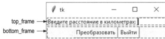
РИС. 13.14. Окно, сформированное рамками Frame
