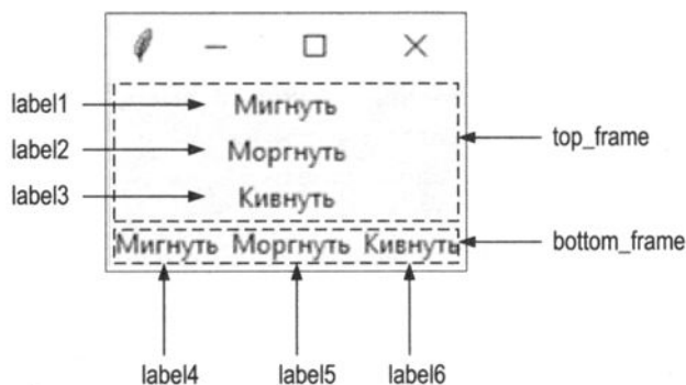
РИС. 13.9. Расположение элементов интерфейса
