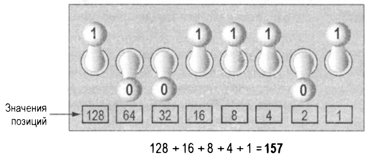
РИС. 1.11. Комбинация двоичных разрядов для числа 157
