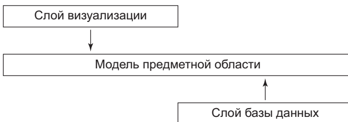
Рис. 2.3. Луковая архитектура
