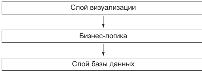
Рис. 2.2. Многослойная архитектура
