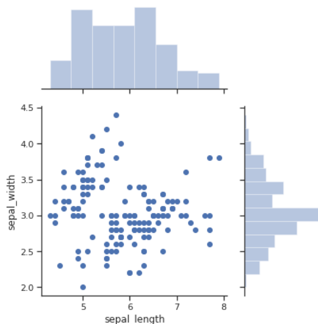
Рисунок 12.30 — Демонстрация работы с параметром ratio функции jointplot()
