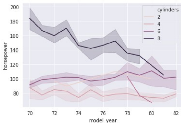
Рисунок 8.31 — Представление сокращённого набора значений признака в легенде
