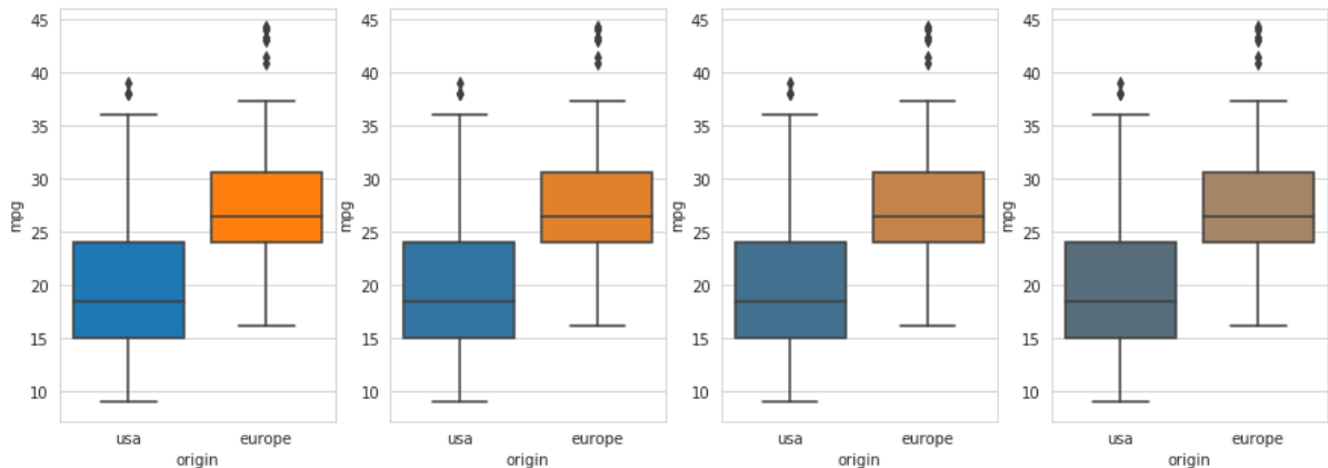
Рисунок 9.24 — Демонстрация работы с параметром saturation
