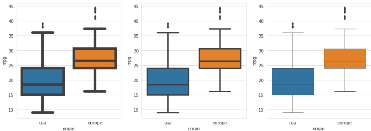
Рисунок 9.25 — Демонстрация работы с параметром linewidth
