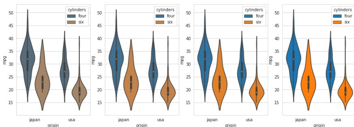
Рисунок 9.37 — Демонстрация работы с параметром saturation функции violinplot()
