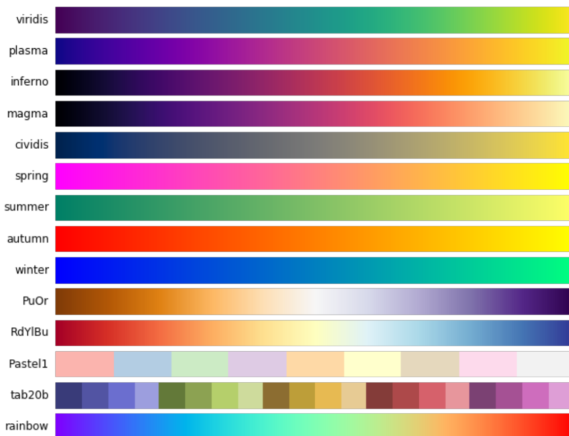
Рисунок 4.29 — Цветовые карты
