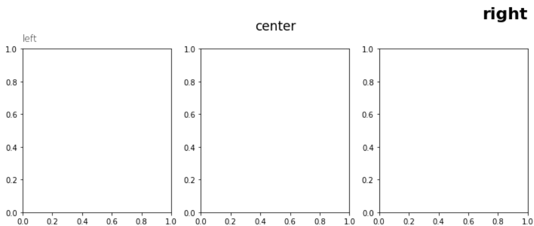
Рисунок 3.12 — Заголовок графика
