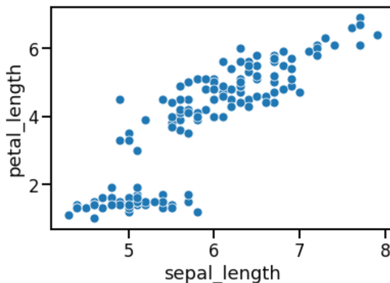
Рисунок 7.9 — Контекст talk
