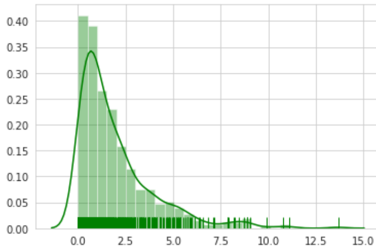
Рисунок 10.7 — Демонстрация работы функции distplot() с параметром color
