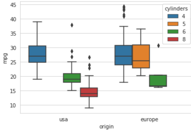
Рисунок 9.26 — Демонстрация работы с параметром hue
