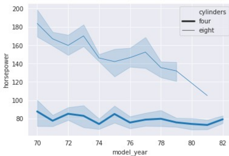
Рисунок 8.17 — Демонстрация работы с параметром size_order
