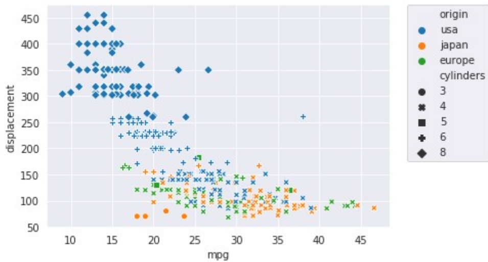
Рисунок 8.25 — Демонстрация работы с параметром style
