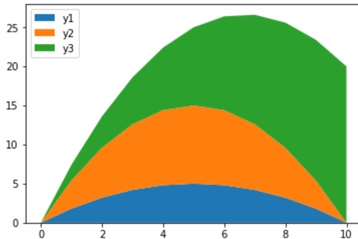
Рисунок 4.13 — Стековый график
