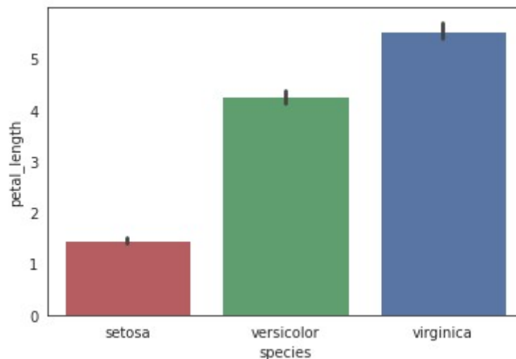
Рисунок 7.20 — Палитра deep
