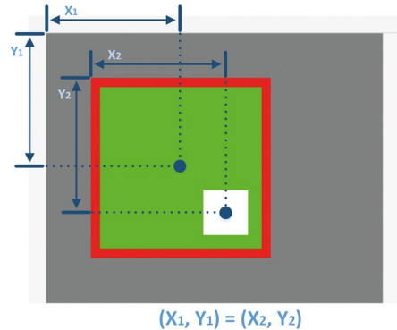
Рис. 16.17. Ошибка в совмещении центров представлений
