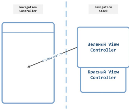
Рис. 9.14. Два View Controller в навигационном стеке
