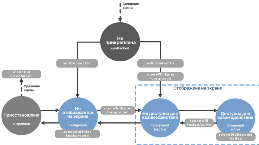
Рис. 5.8. Схема жизненного цикла сцены
