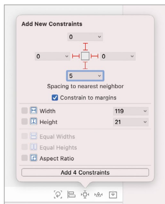
Рис. 14.24. Создание ограничений для верхней метки
