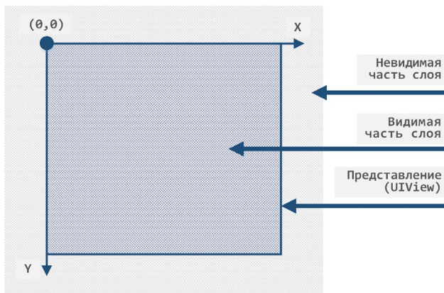
Рис. 16.18. UIView и CALayer
