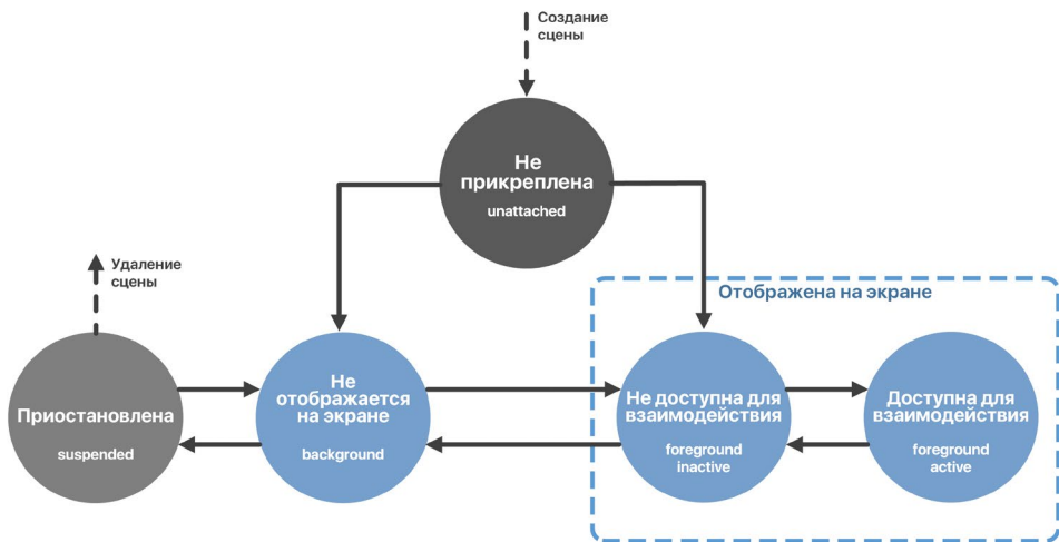
Рис. 5.7. Схема жизненного цикла сцены
