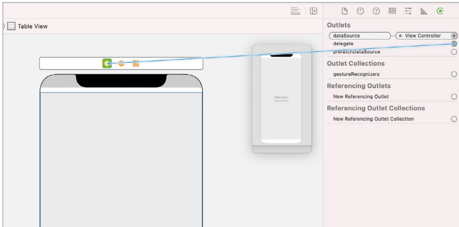
Рис. 7.32. Связь View Controller и Table View
