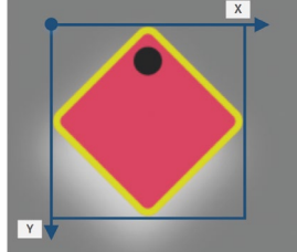
Рис. 16.34. Размеры view после поворота
