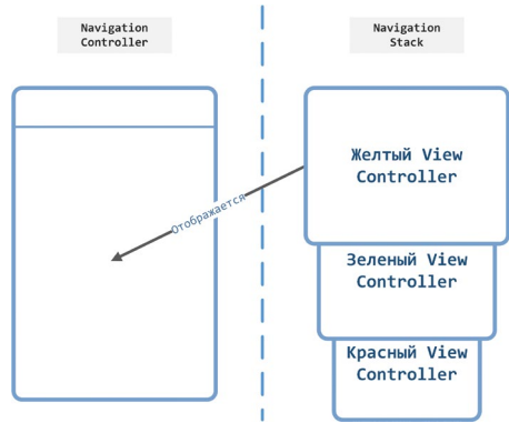
Рис. 9.15. Три View Controller в навигационном стеке
