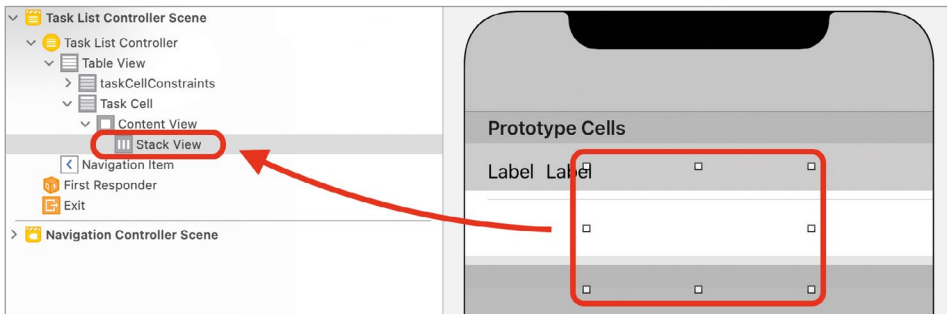
Рис. 12.13. Горизонтальный стек в ячейке
