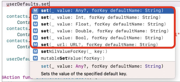
Рис. 8.2. Автодополнение для метода set
