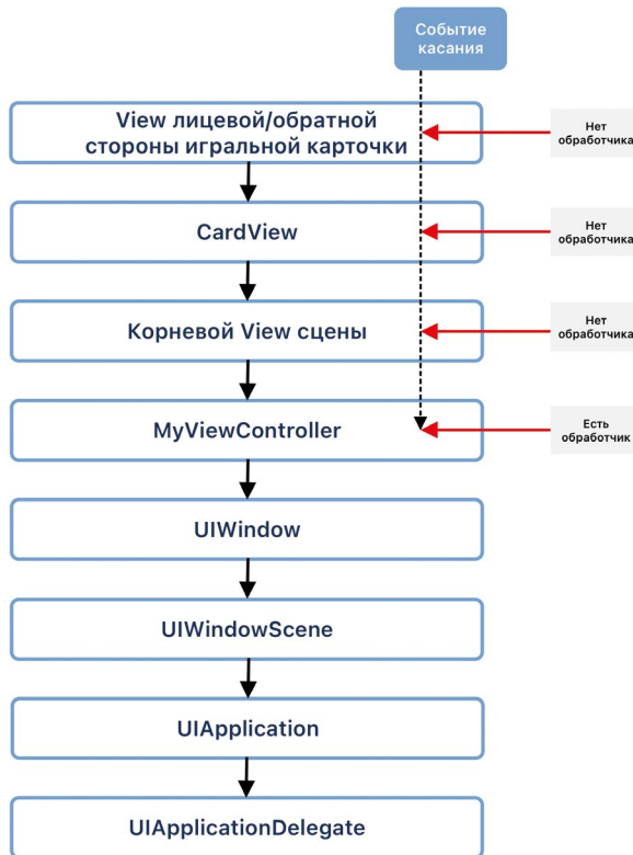
Рис. 19.4. Пример Responder Chain
