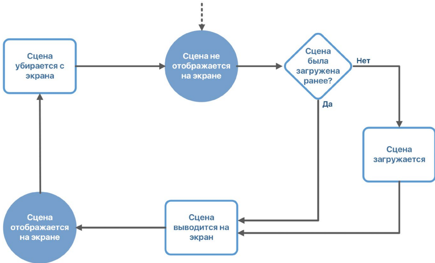
Рис. 3.2. Жизненный цикл View Controller
