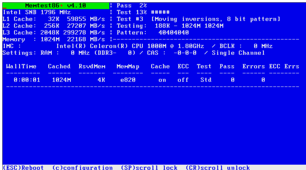
Рис. 11.11. Программа memtest86+
