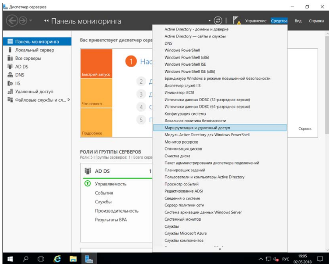
Рис. 5.3. Диспетчер серверов
