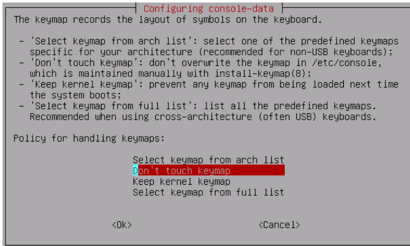
Рис. 6.18. Выбор раскладки
