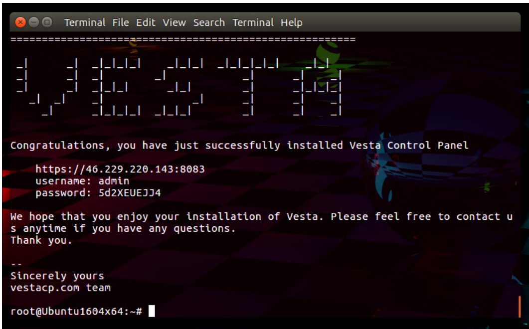
Рис. 8.27. Установка завершена
