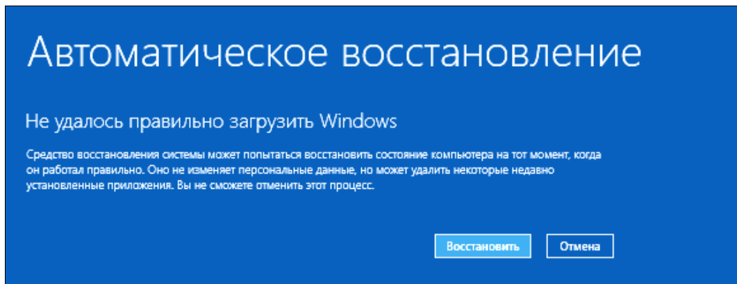
Рис. 11.12. Автоматическое восстановление
