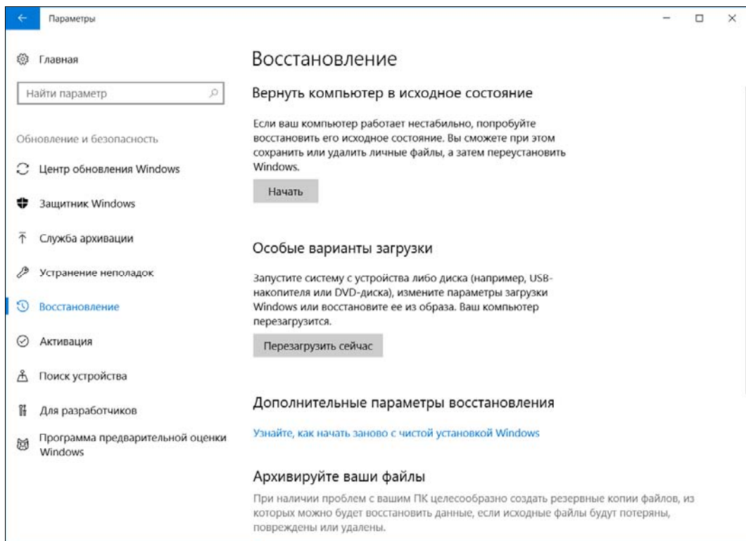
Рис. 11.20. Раздел Восстановление
