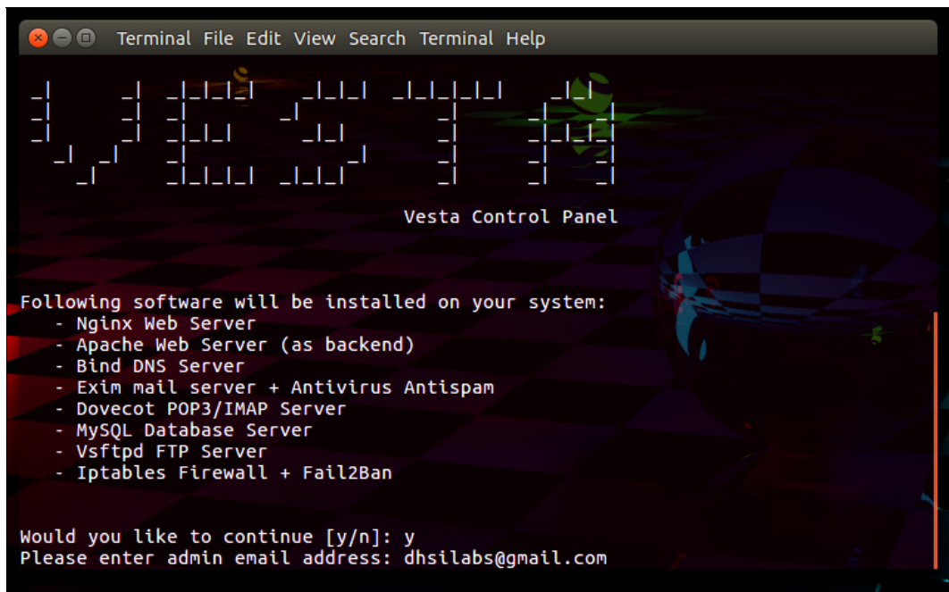
Рис. 8.25. Подтверждение установки
