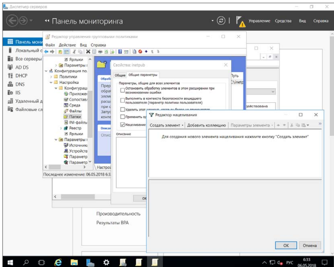
Рис. 6.9. Редактор нацеливания
