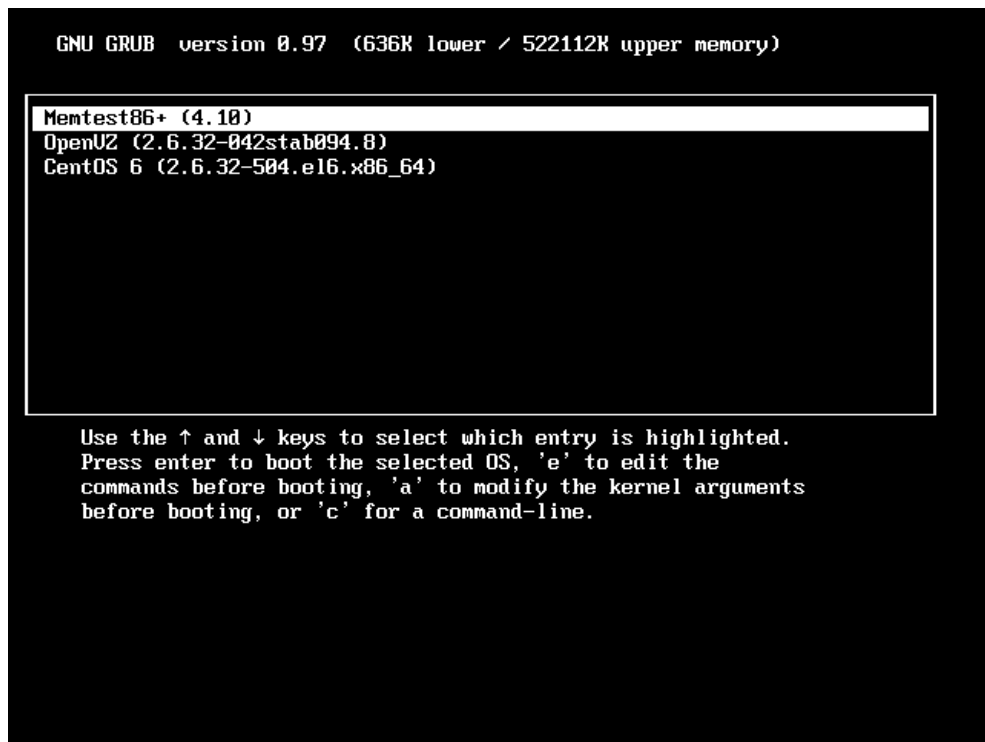
Рис. 11.10. Загрузчик Linux
