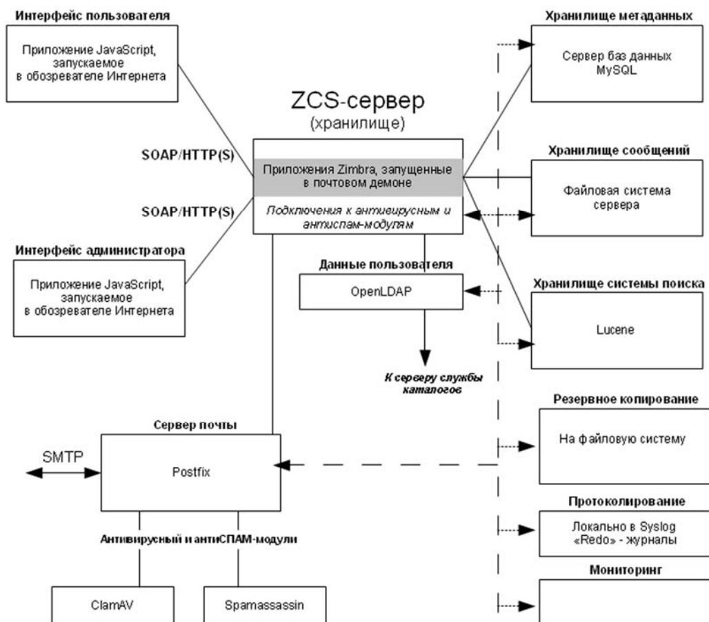
Рис. 2.8. Архитектура ZCS
