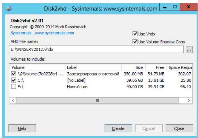
Рис. 8.22. Утилита Disk2vhd
