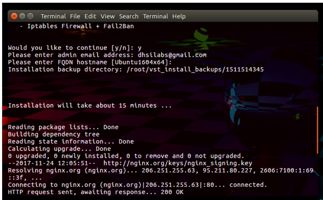
Рис. 8.26. Началась установка
