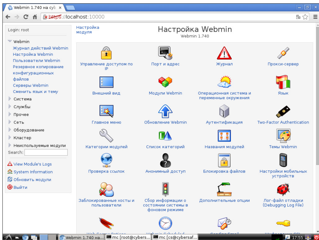
Рис. 2.10. Веб-интерфейс Webmin
