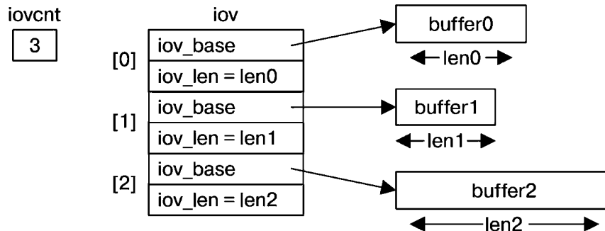
Рис. 5.3. Пример массива iov и связанных с ним буферов
