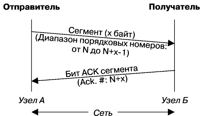
Рис. 57.3. Подтверждения в протоколе TCP
