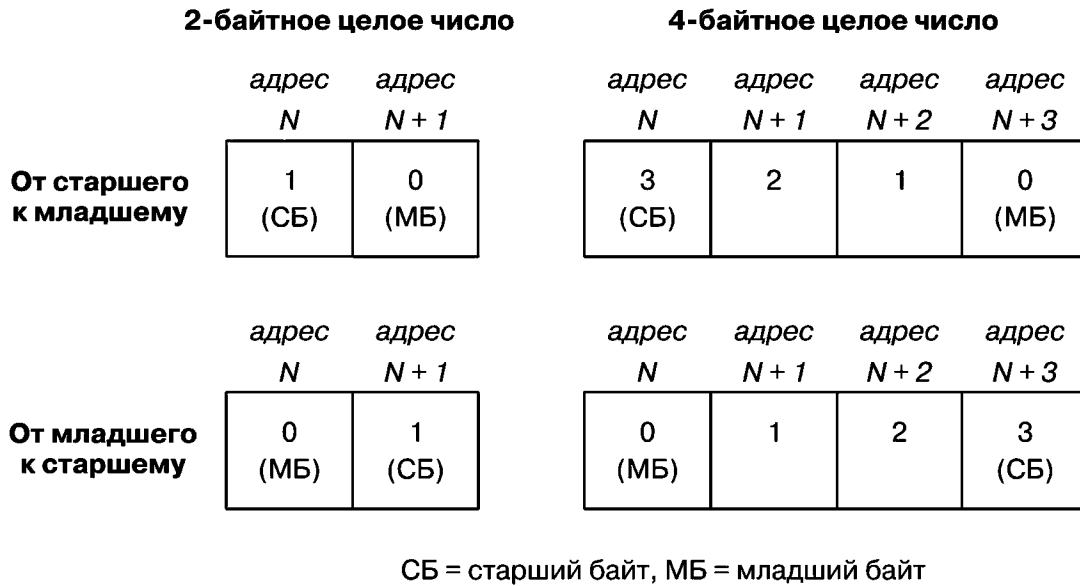
Рис. 55.1. Разный порядок следования байтов в 2- и 4-байтных целых числах
