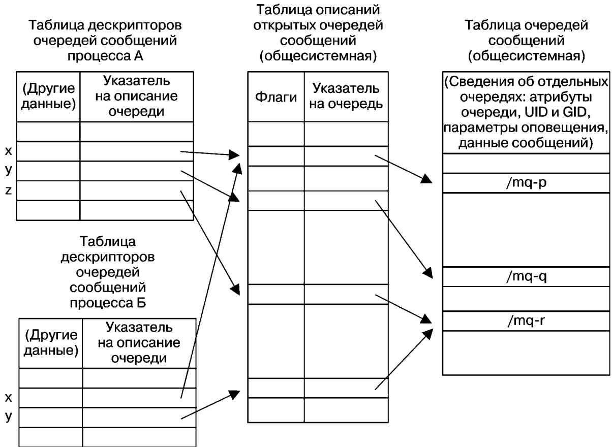
Рис. 48.1. Связь между структурами данных ядра для очередей POSIX-сообщений
