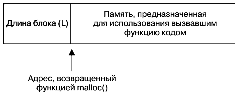
Рис. 7.1. Блок памяти, возвращенный функцией malloc()
