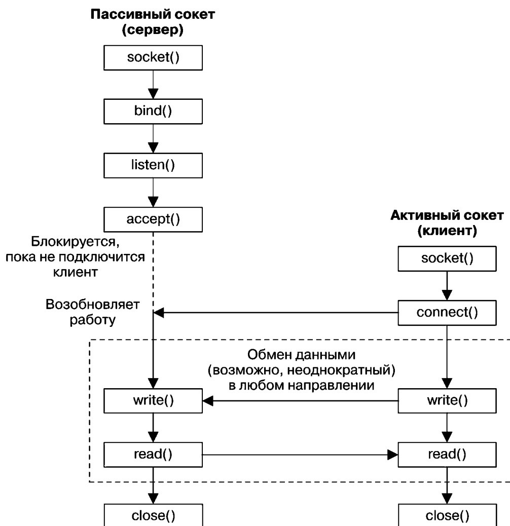
Рис. 52.1. Общая схема системных вызовов, применяемых для работы с потокосыми сокетами
