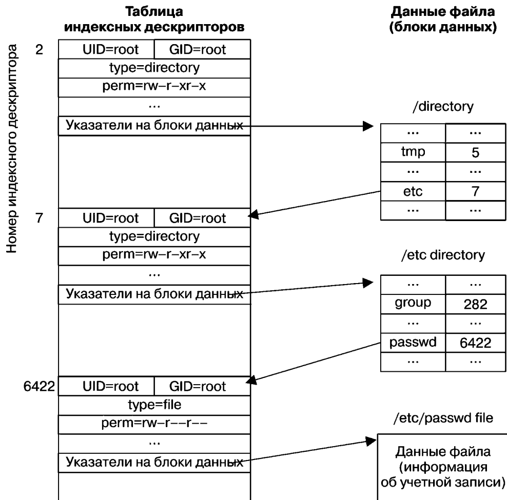
Рис. 18.1. Взаимосвязь между структурами индексных дескрипторов и каталогов для файла /etc/passwd
