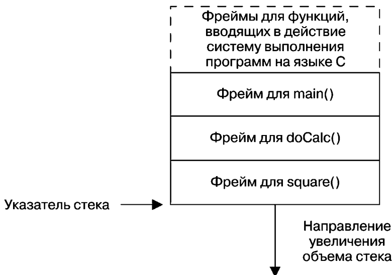
Рис. 6.3. Пример стека процесса
