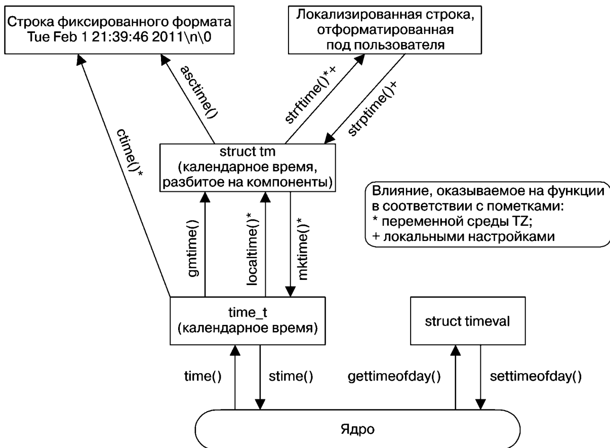
Рис. 10.1. Функции для извлечения календарного времени и работы с ним
