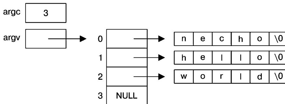
Рис. 6.4. Значения argc и argv для команды necho hello world
