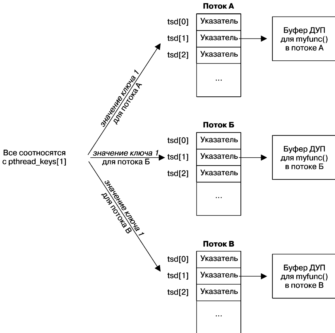
Рис. 31.3. Структура данных, которая используется для реализации указателей на данные уровня потока (ДОП)
