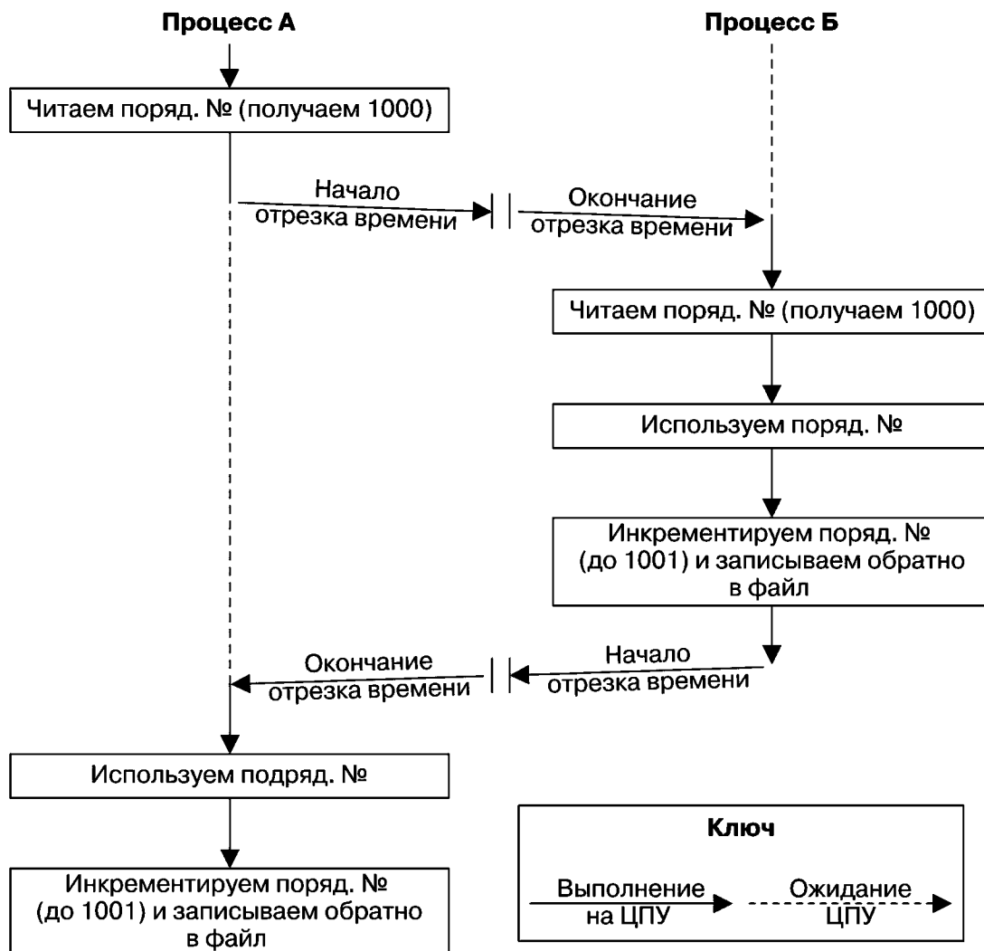
Рис. 51.1. Два процесса одновременно обновляют файл без синхронизации
