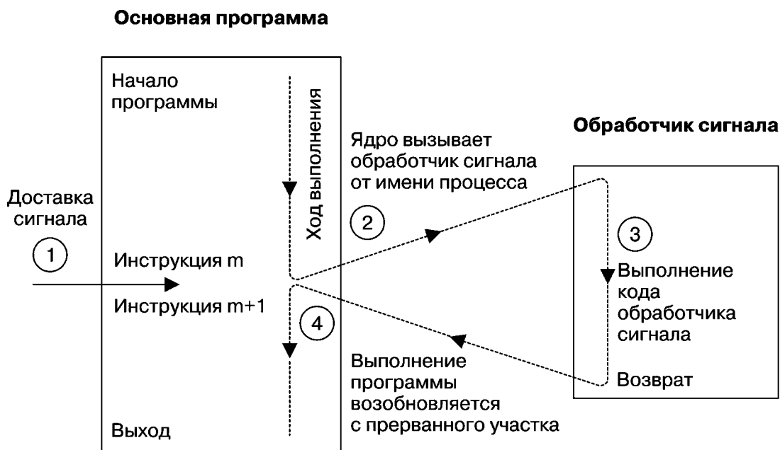
Рис. 20.1. Доставка сигнала и выполнение обработчика
