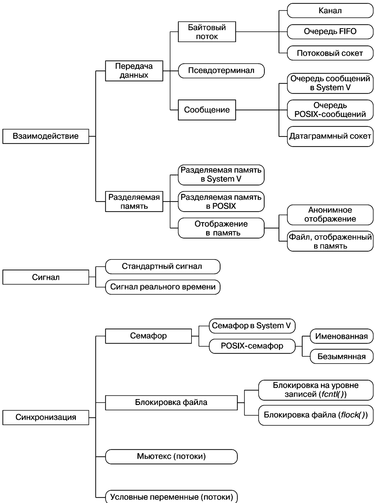
Рис. 43.1. Классификация IPC-механизмов в UNIX
