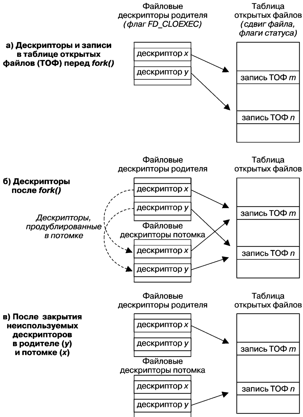
Рис. 24.2. Дублирование файловых дескрипторов во время вызова fork() и закрытие тех из них, которые не используются
