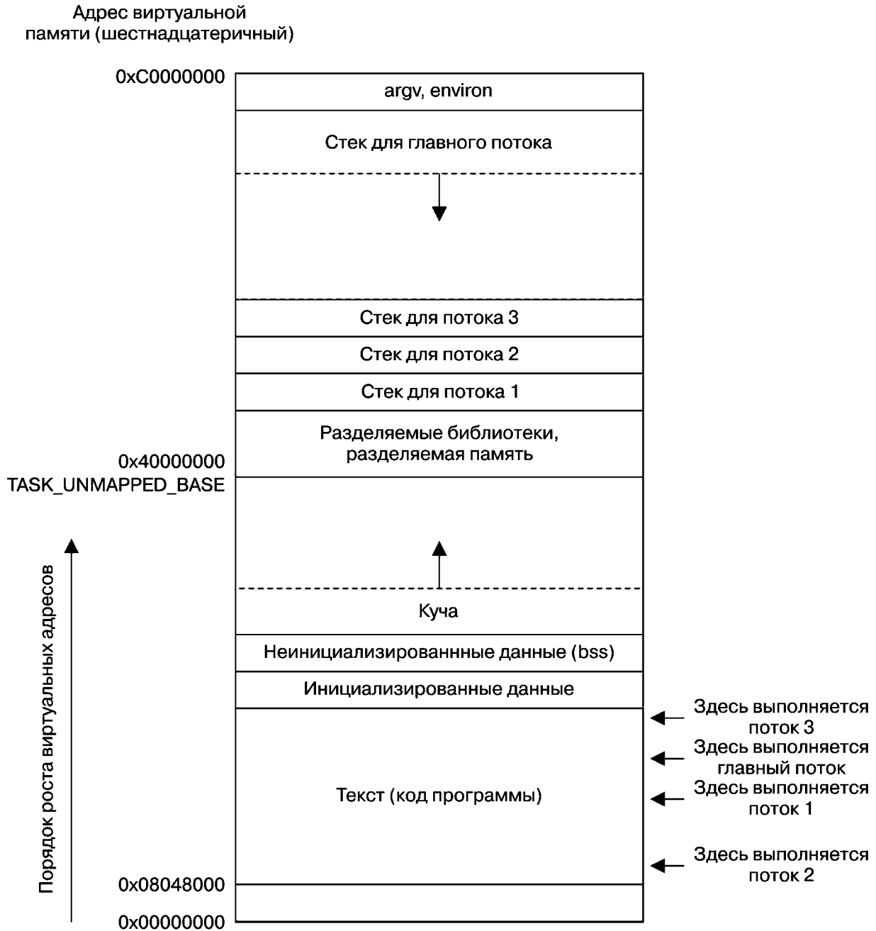
Рис. 29.1. Четыре потока, выполняющиеся внутри процесса (Linux/x86-32)
