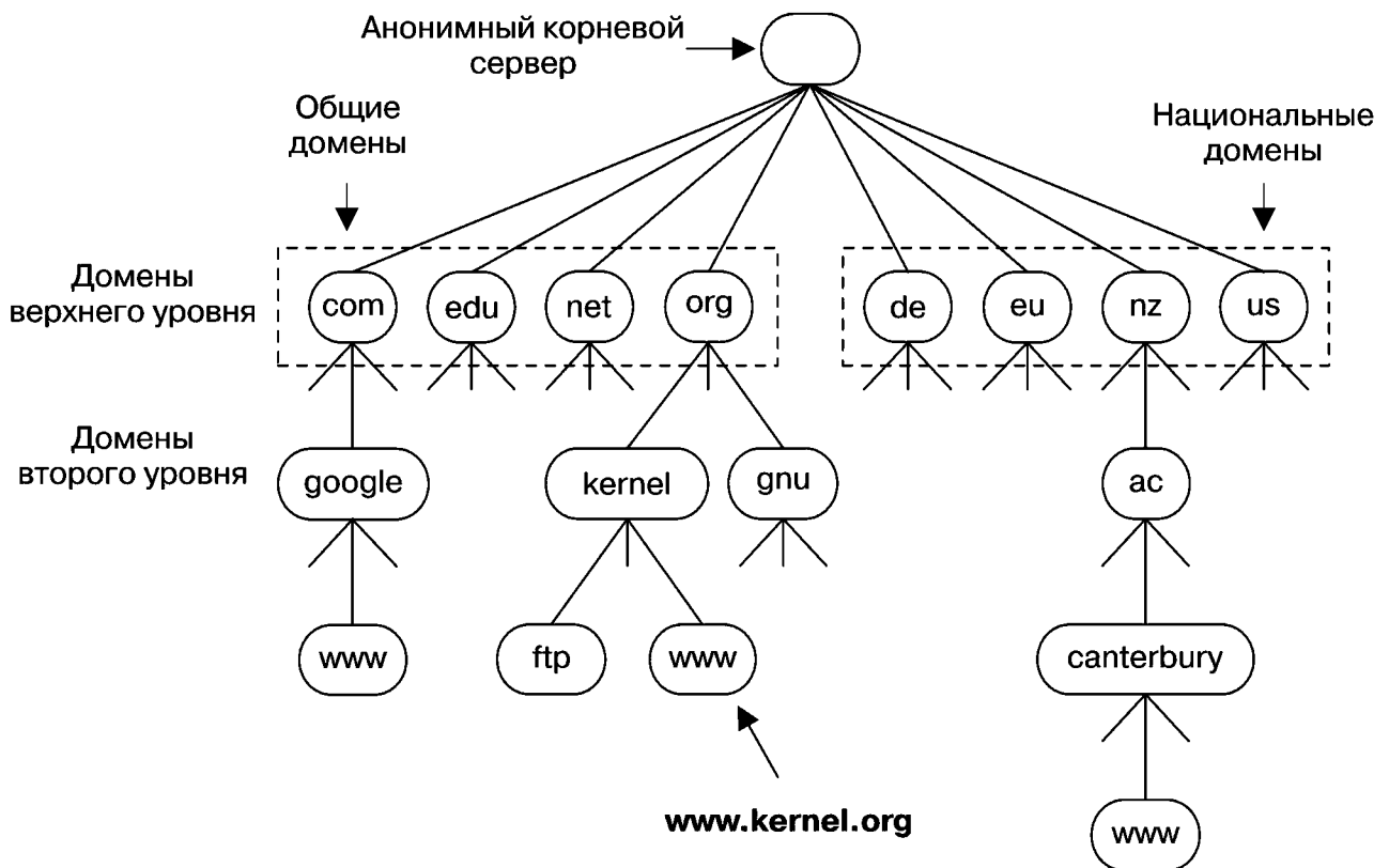
Рис. 55.2. Часть иерархии DNS
