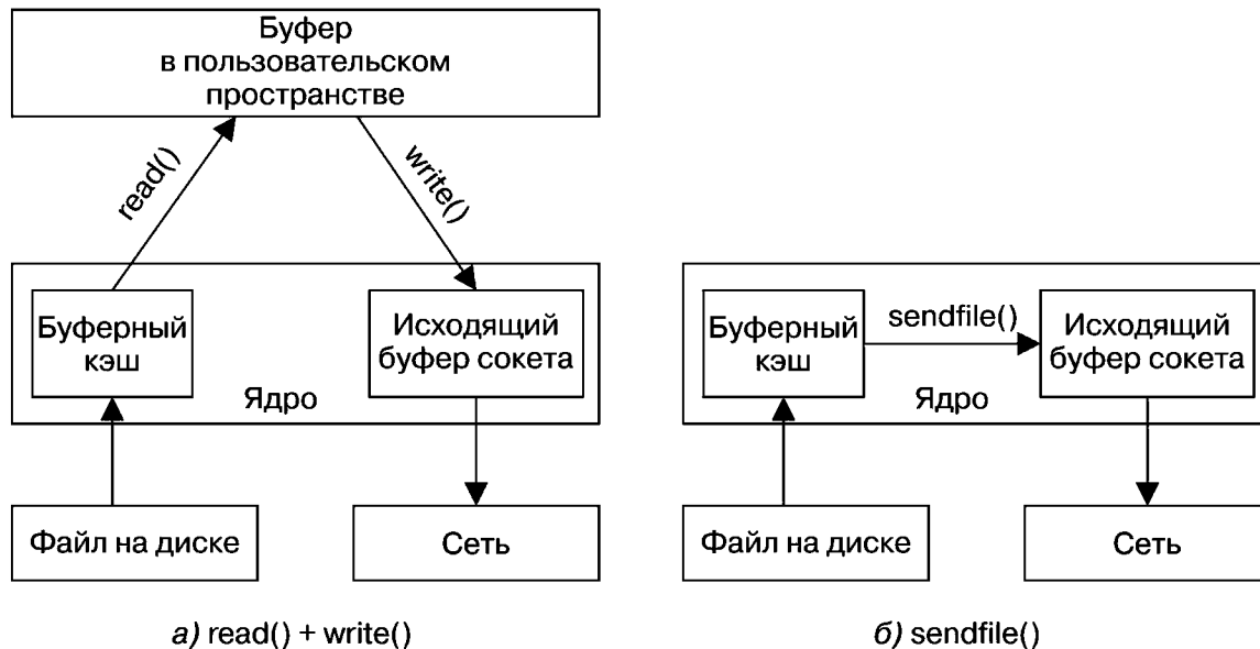
Рис. 57.1. Передача содержимого файла через сокет
