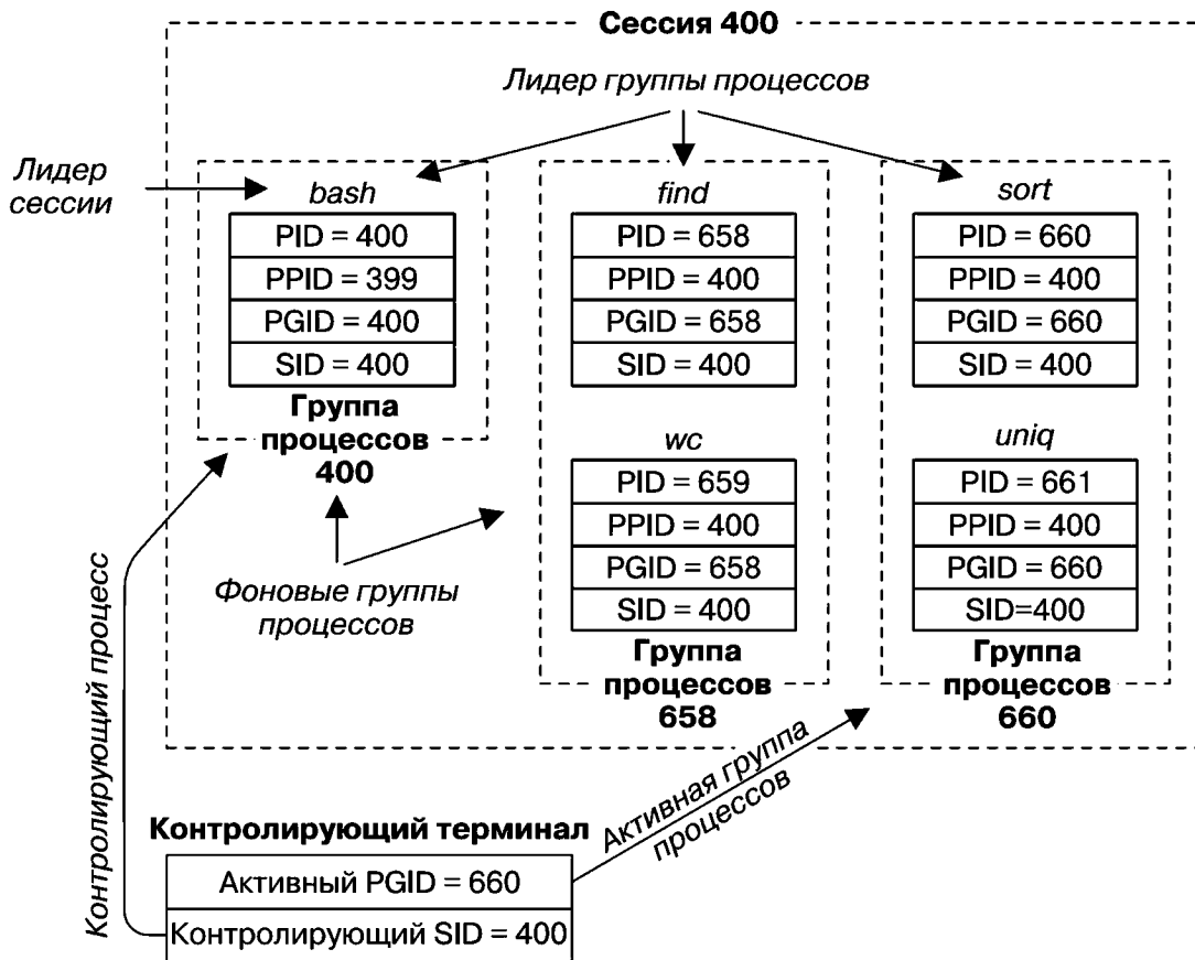
Рис. 34.1. Отношения между группой процессов, сессиями и контролирующим терминалом
