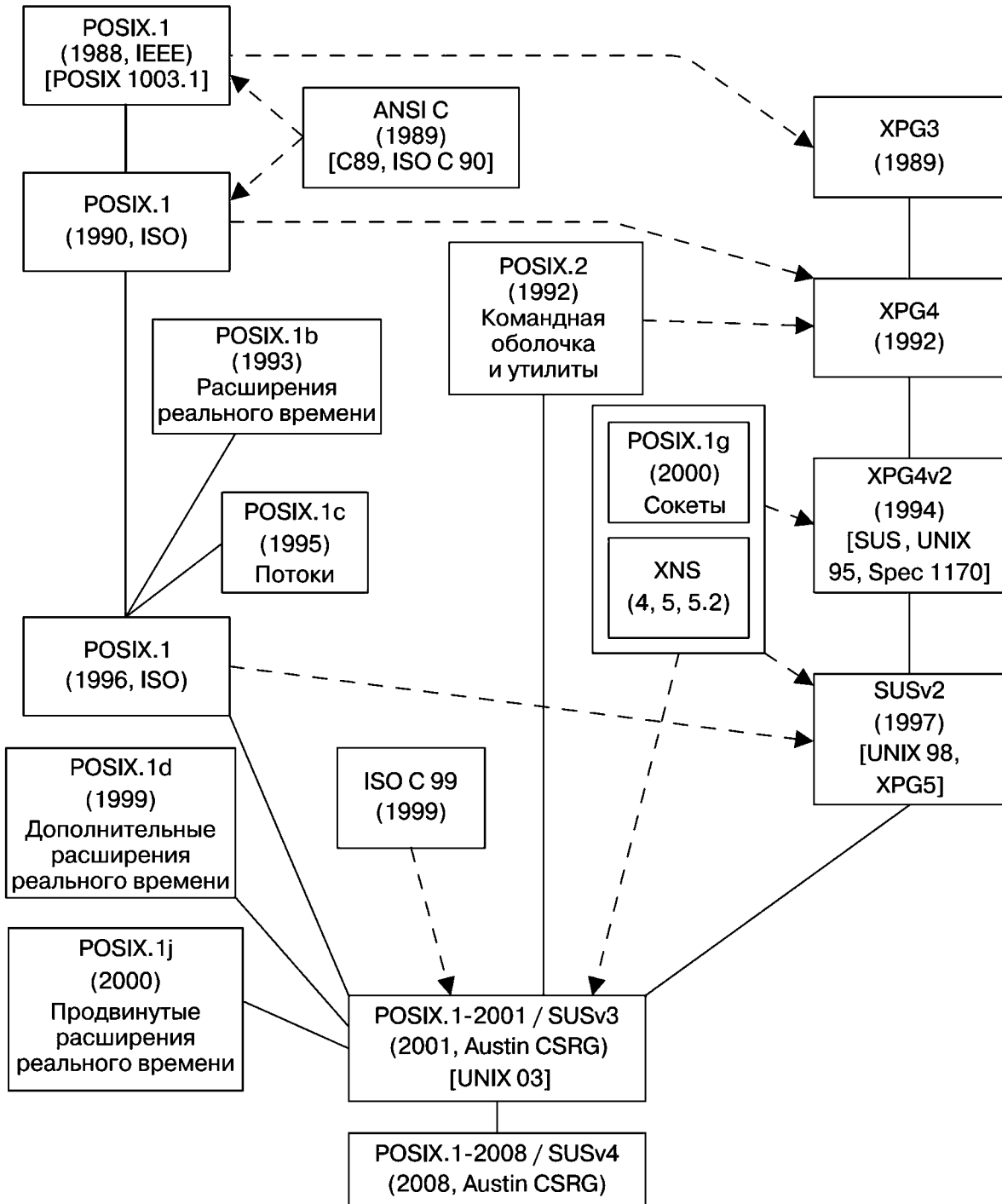
Рис. 1.1. Взаимоотношения между различными стандартами UNIX и C
