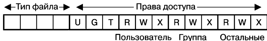
Рис. 15.1. Битовая маска поля st_mode
