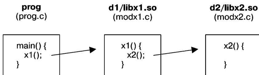
Рис. 41.4. Разделяемая библиотека, зависящая от другой разделяемой библиотеки
