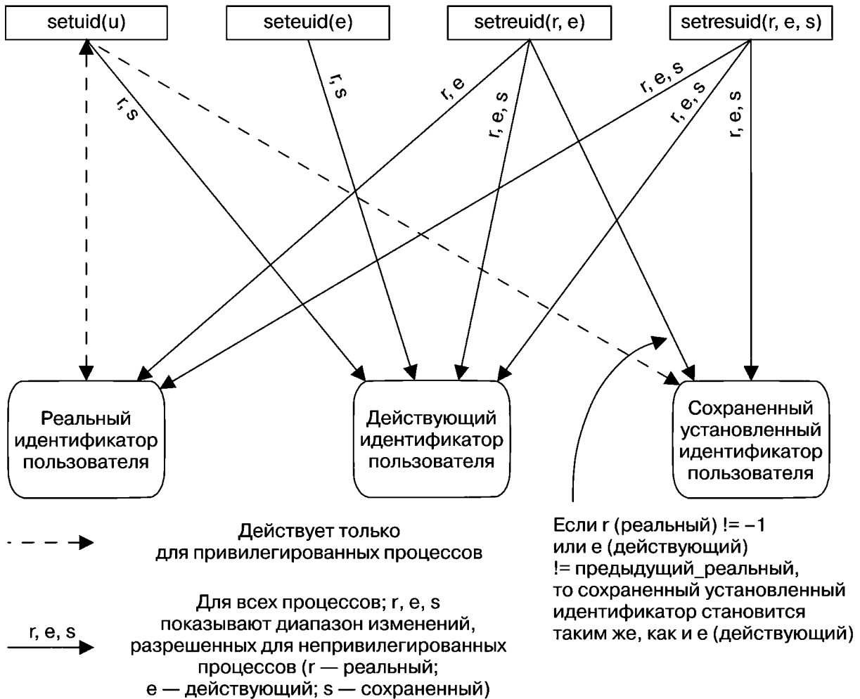
Рис. 9.1. Действия функций, изменяющих полномочия процесса, связанные с его пользовательскими идентификаторами
