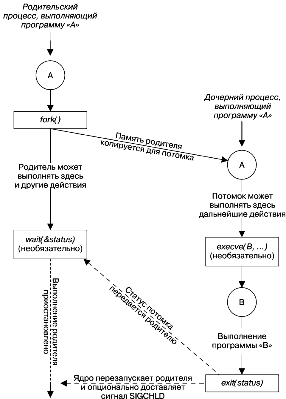
Рис. 24.1. Обор вызовов fork() , exit() , wait() и execve()
