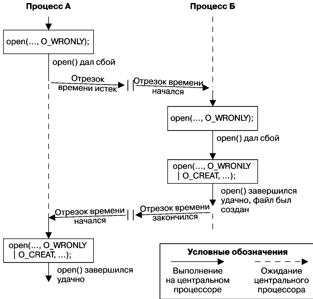
Рис. 5.1. Неудачная попытка эксклюзивного создания файла
