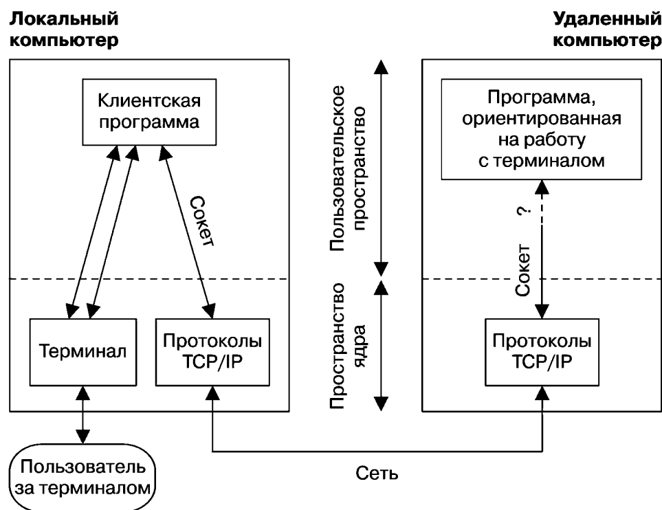
Рис. 60.1. Как управлять по сети программой, ориентированной на работу с терминалом?
