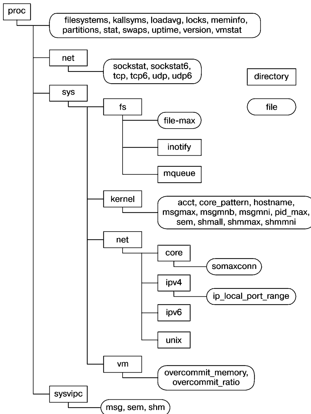
Рис. 12.1. Отдельные файлы и подкаталоги, находящиеся в /proc
