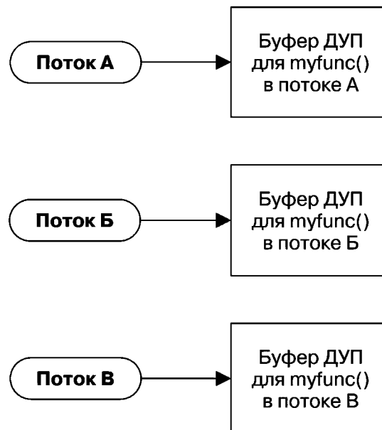
Рис. 31.1. Данные уровня потока (ДУП) предоставляют функции хранилище, относящееся к отдельному потоку
