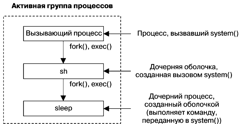
Рис. 27.2. Организация процессов во время выполнения system("sleep 20")
