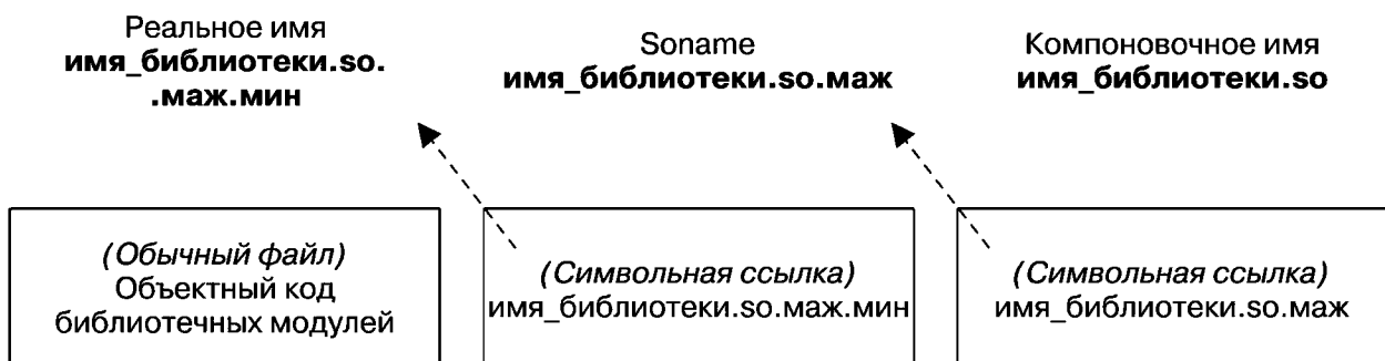
Рис. 41.3. Традиционная структура имен разделяемой библиотеки
