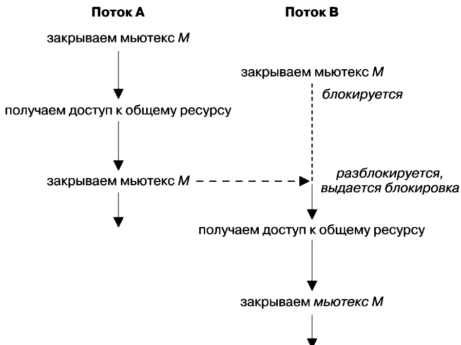
Рис. 30.2. Использование мьютекса для защиты критического участка
