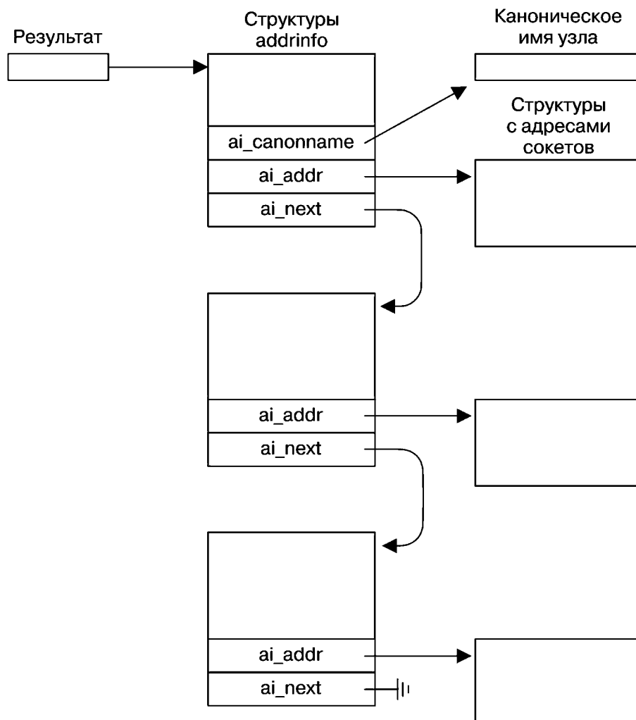
Рис. 55.3. Структуры, выделяемые и возвращаемые функцией getaddrinfo()
