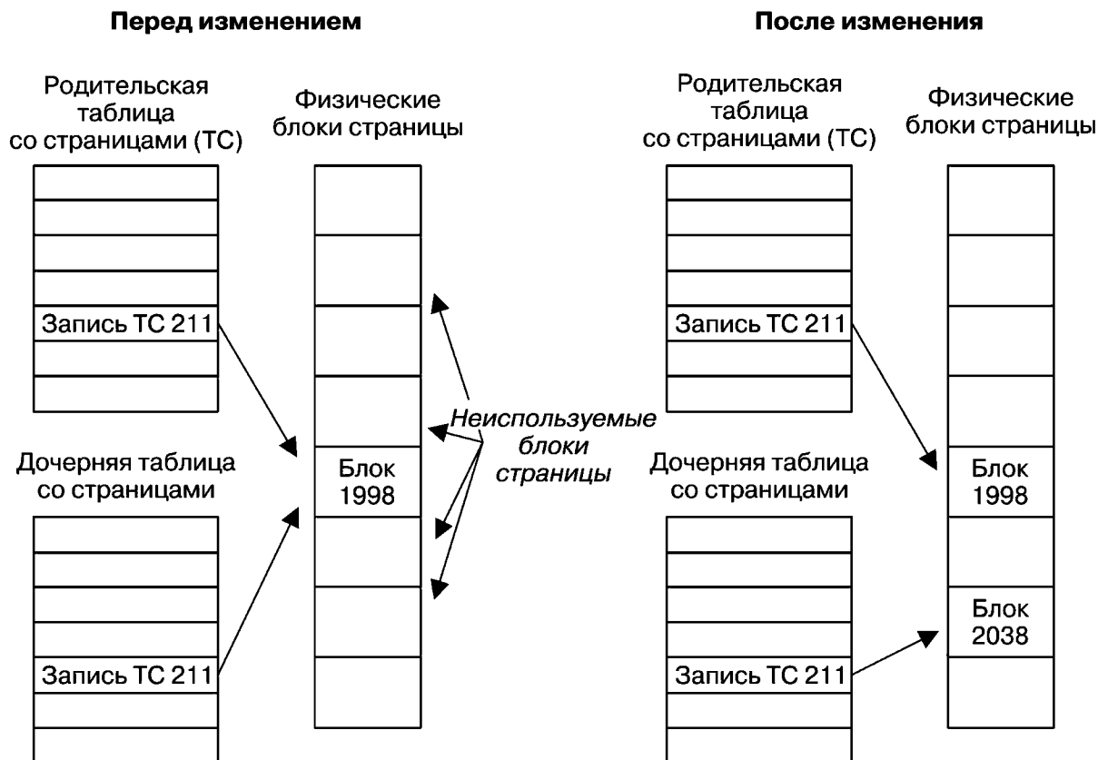
Рис. 24.3. Таблицы со страницами памяти до и после изменения общей страницы, копируемой при записи
