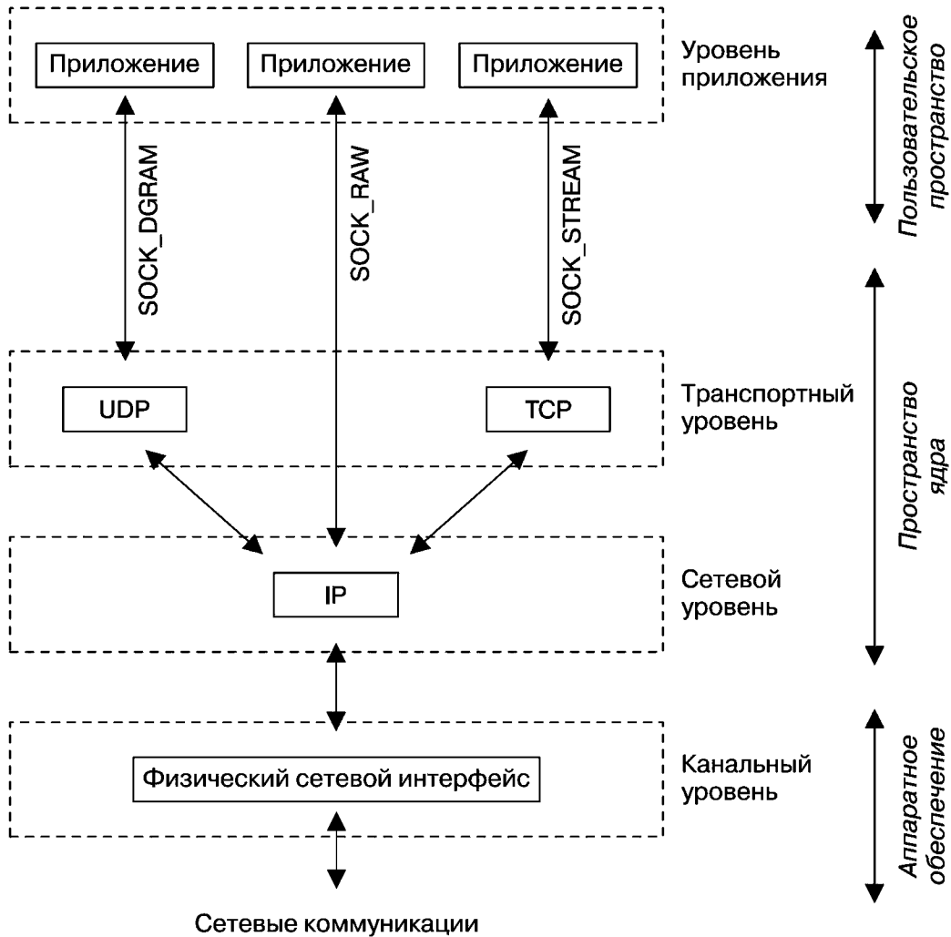
Рис. 54.2. Протоколы семейства TCP/IP
