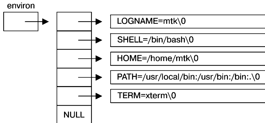
Рис. 6.5. Пример структуры данных в отношении списка переменных среды для процесса
