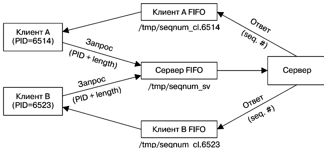
Рис. 44.6. Применение очередей FIFO в приложении с одним сервером и несколькими клиентами
