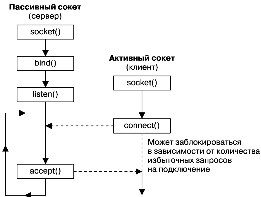
Рис. 52.2. Отложенное соединение с сокетом
