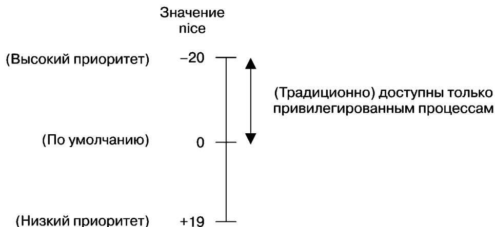
Рис. 35.1. Диапазон и интерпретация значений nice
