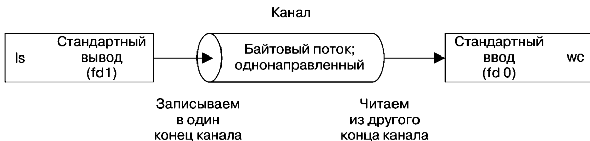
Рис. 44.1. Использование канала для соединения двух процессов
