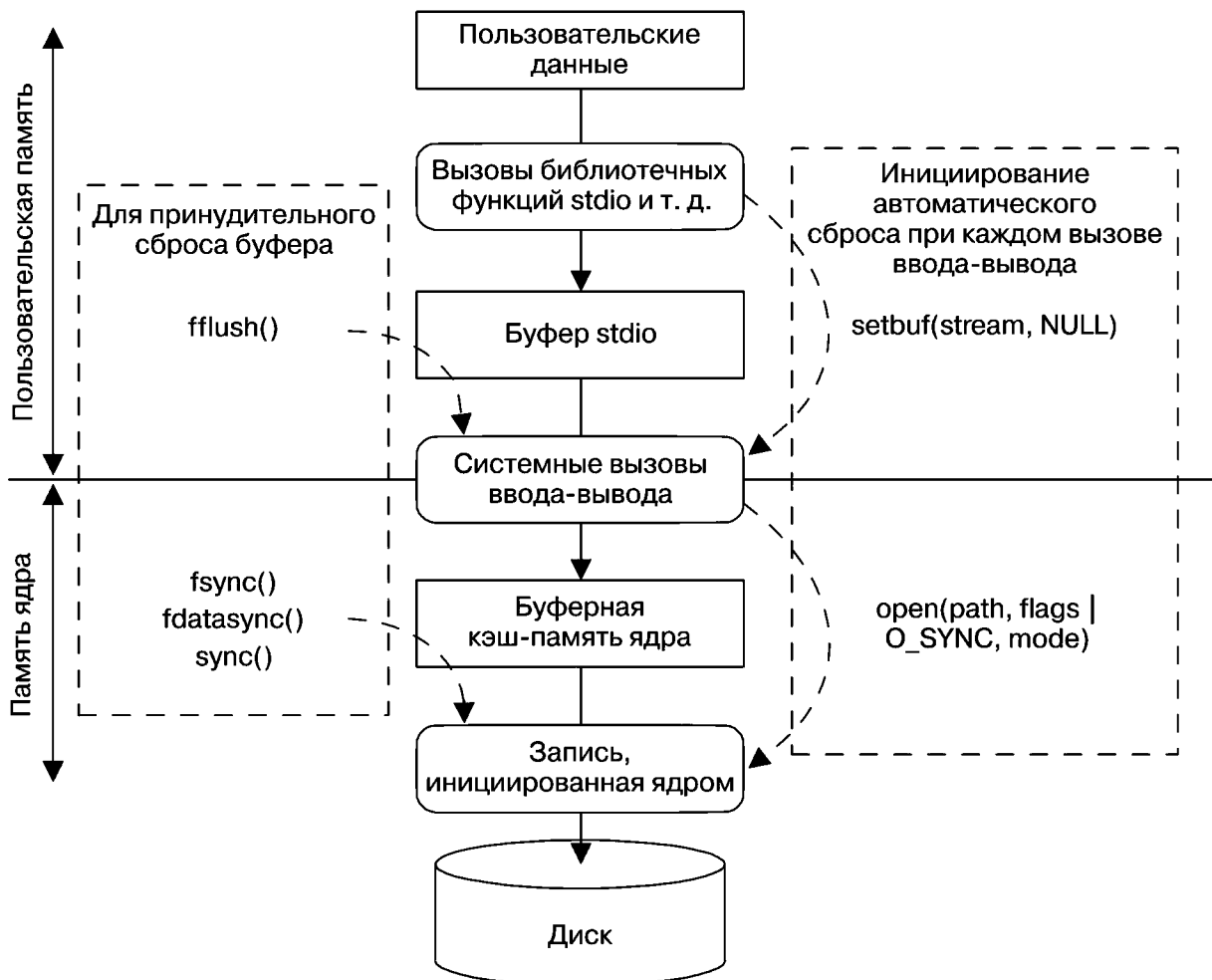
Рис. 13.1. Обзор буферизации ввода-вывода
