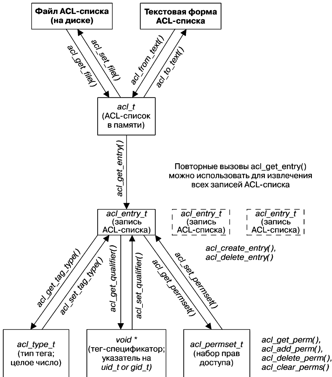
Рис. 17.2. Взаимосвязь между библиотечными ACL-функциями и структурами данных
