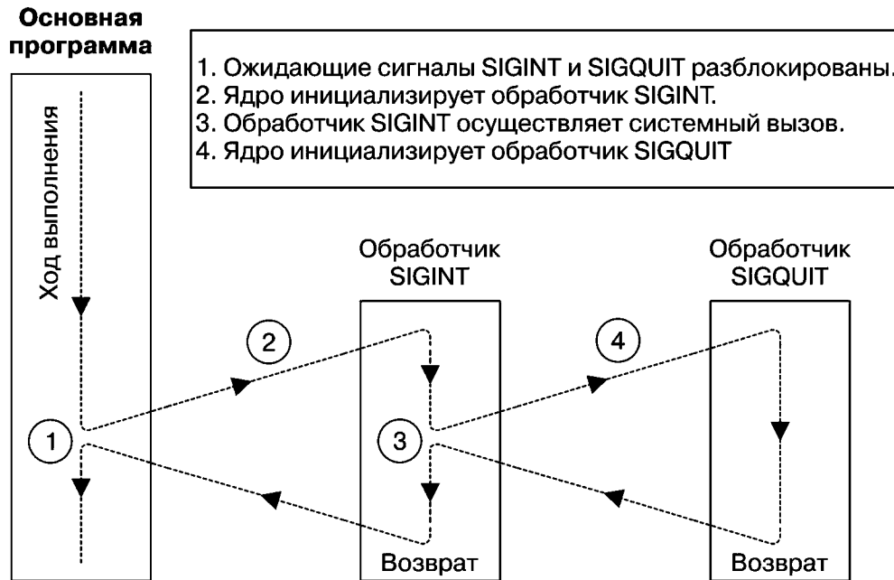
Рис. 22.1. Доставка нескольких разблокированных сигналов
