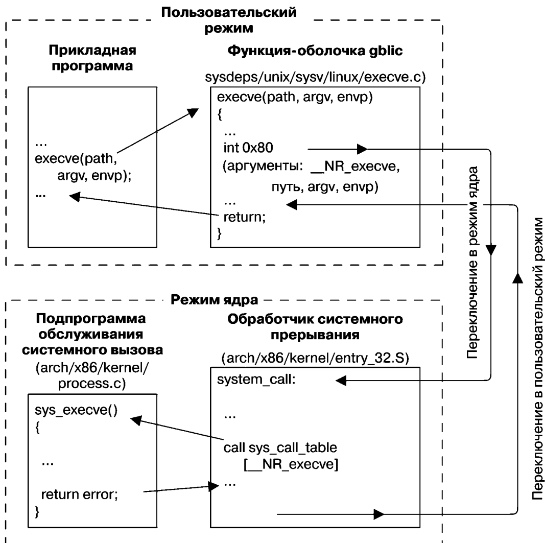
Рис. 3.1. Этапы выполнения системного вызова
