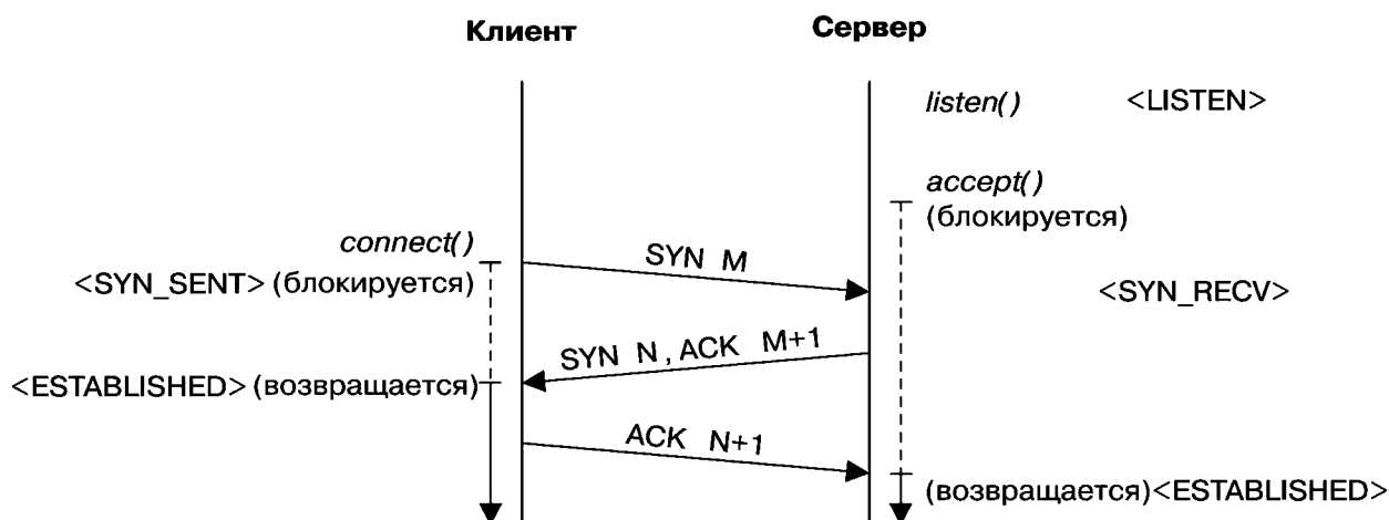
Рис. 57.5. Трехэтапное согласование при установке TCP-соединения
