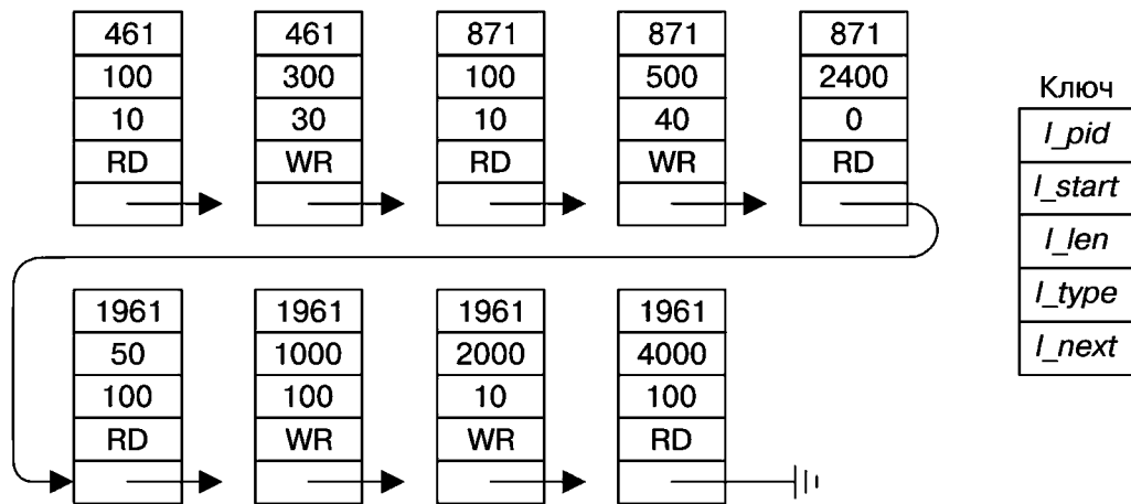
Рис. 51.6. Пример списка блокировок записей для одного файла
