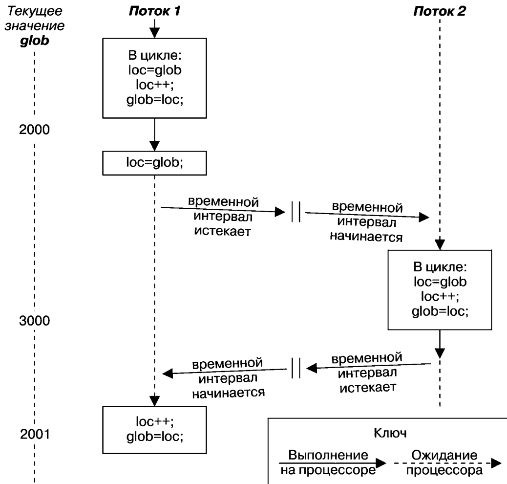
Рис. 30.1. Два потока, инкрементирующих глобальную переменную без синхронизации
