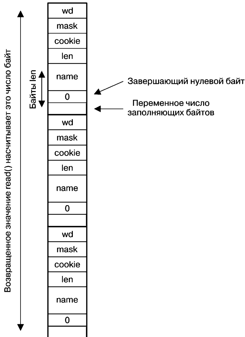
Рис. 19.2. Входящий буфер, содержащий три структуры inotify_event
