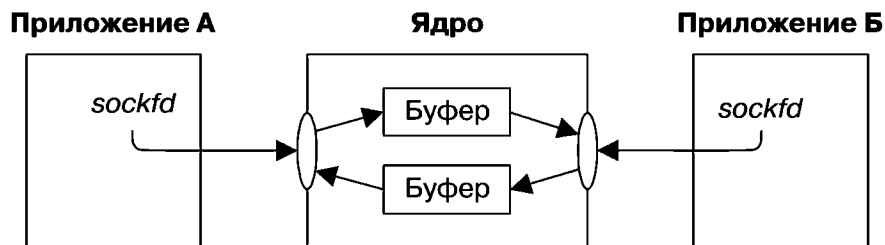
Рис. 52.3. Потоковые сокеты домена UNIX предоставляют двунаправленный канал взаимодействия
