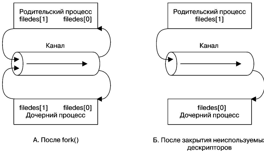
Рис. 44.3. Подготовка канала к передаче данных от родителя к потомку
