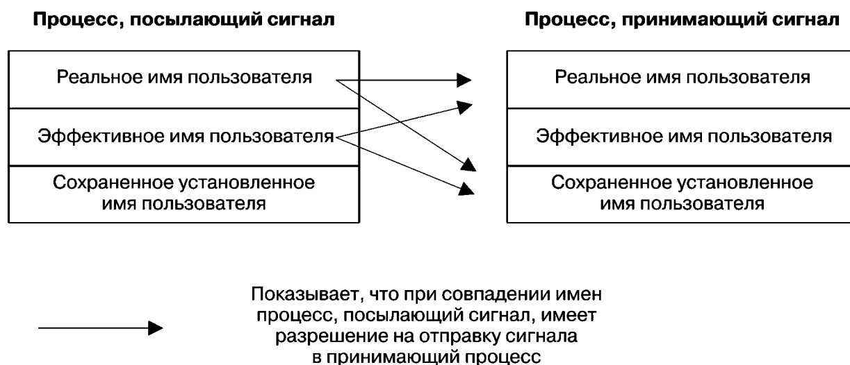
Рис. 20.2. Разрешения, необходимые непривилегированному процессу для отправки сигнала
