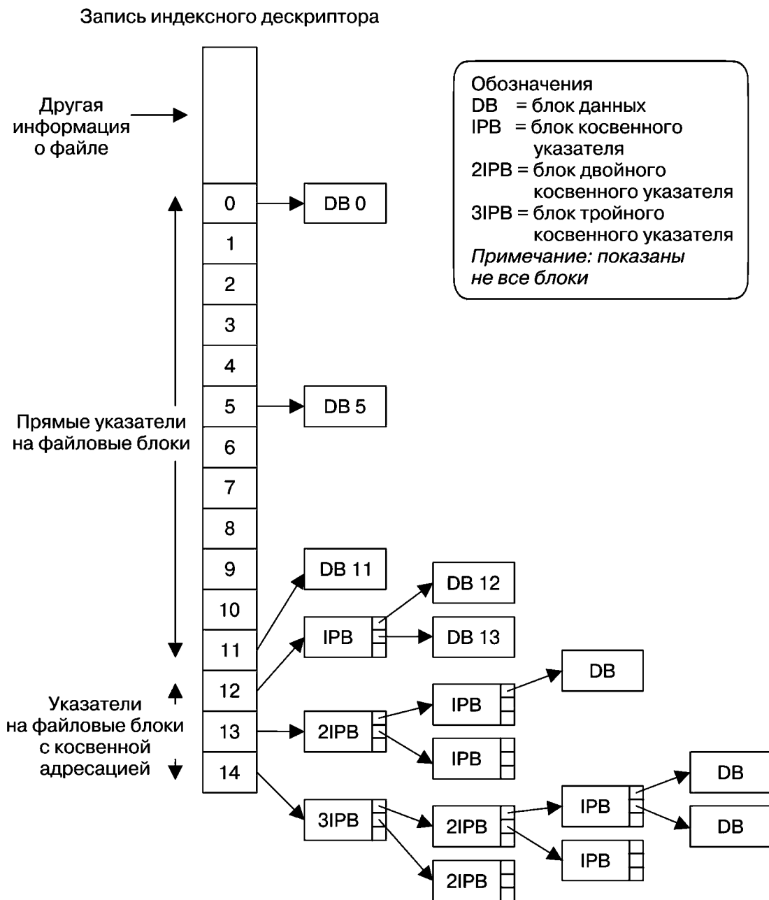
Рис. 14.2. Структура файловых блоков для файла в файловой системе ext2
