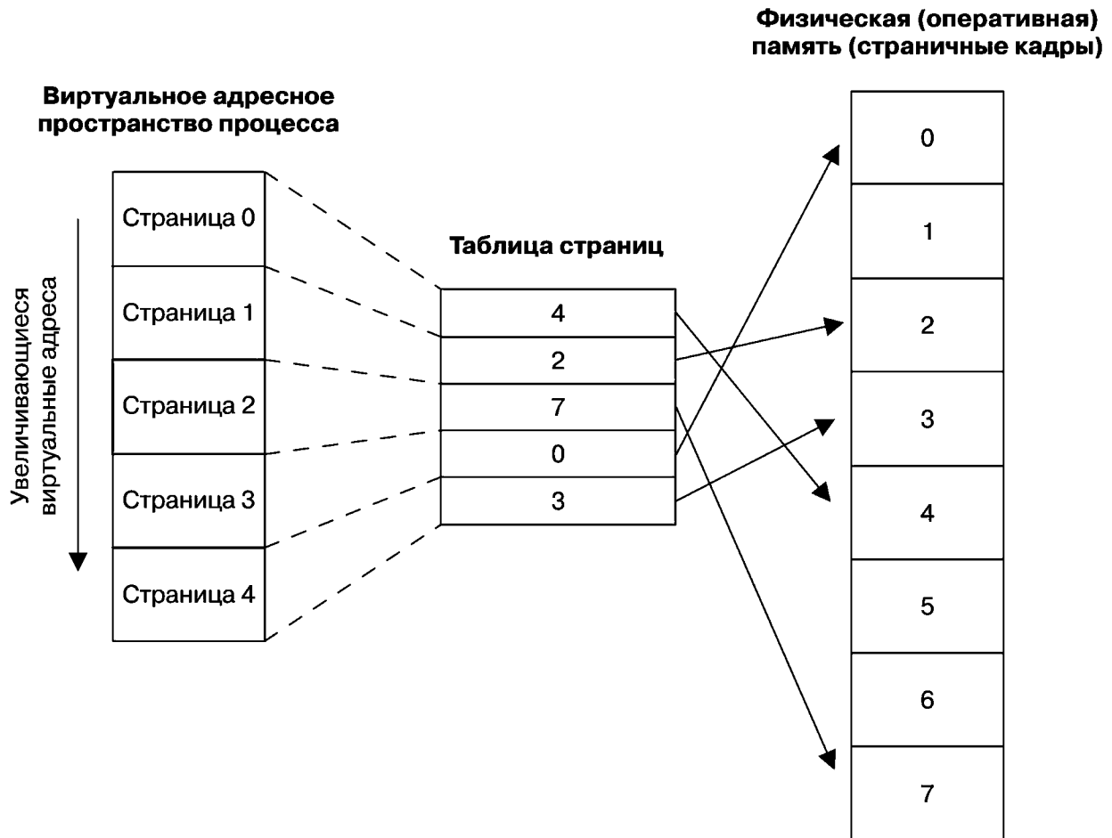
Рис. 6.2. Общий вид виртуальной памяти
