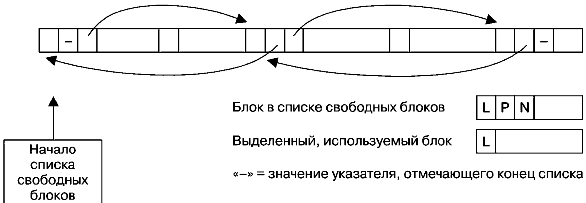
Рис. 7.3. Куча, содержащая выделенные блоки и блоки, входящие в список свободных блоков
