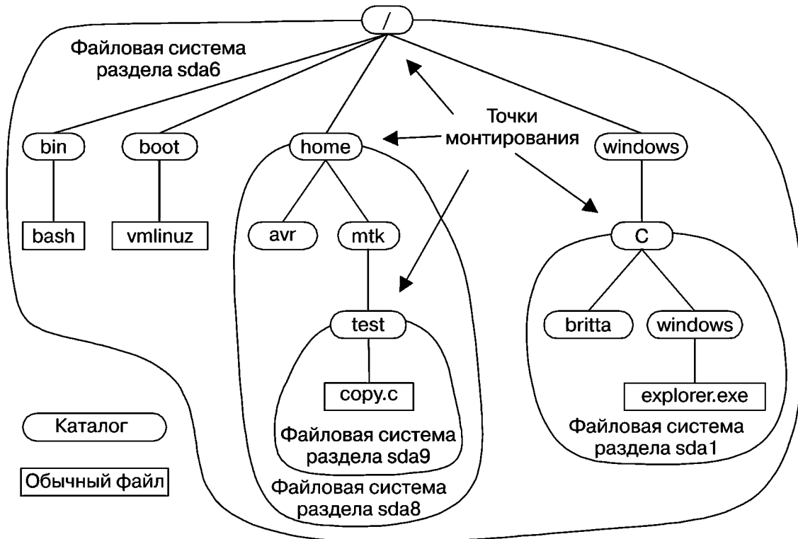
Рис. 14.4. Пример иерархии каталога, в которой показаны точки монтирования файловой системы
