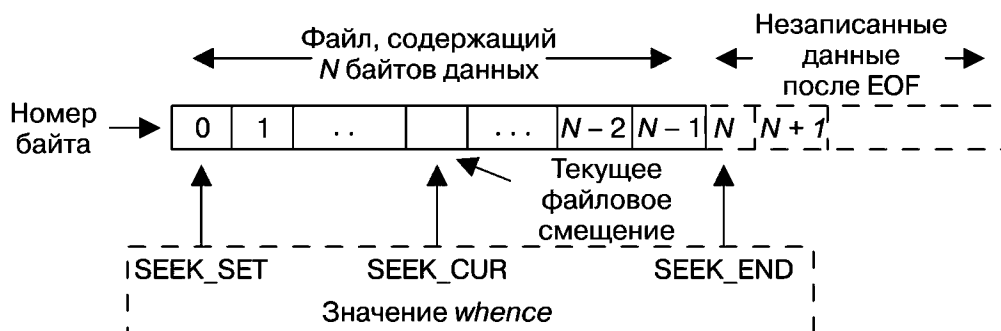
Рис. 4.1. Интерпретация аргумента whence системного вызова lseek()
