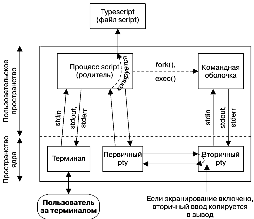
Рис. 60.4. Программа script
