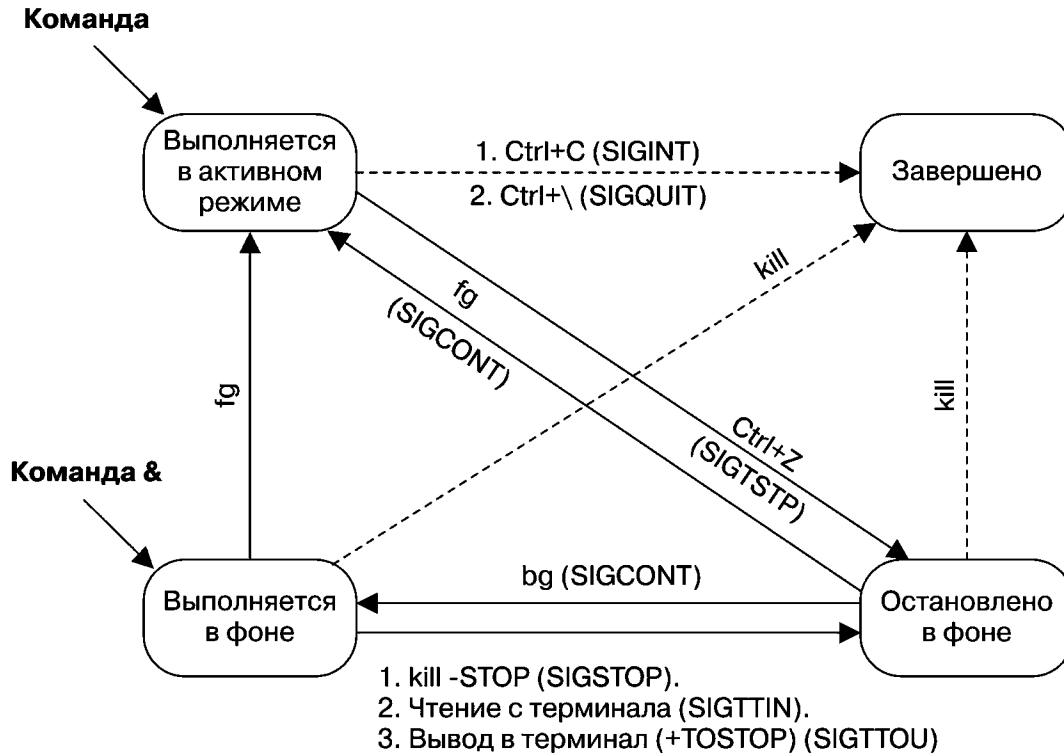
Рис. 34.2. Состояния задания
