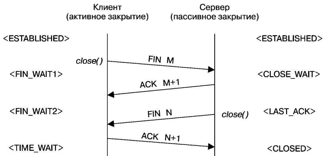
Рис. 57.6. Разрыв TCP-соединения
