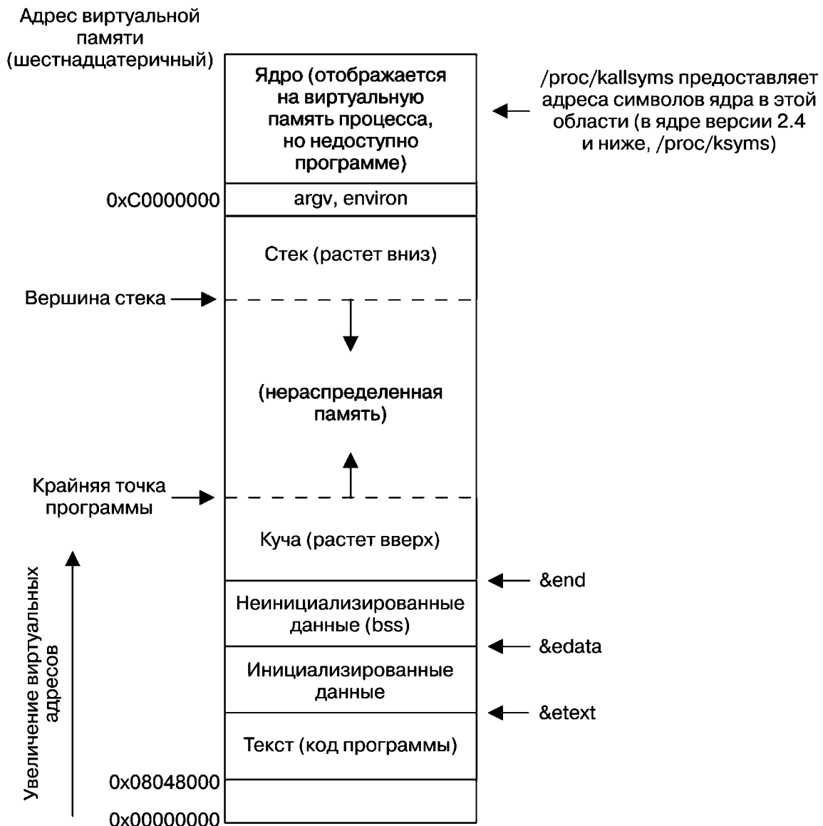
Рис. 6.1. Типичная структура памяти процесса в Linux/x86-32
