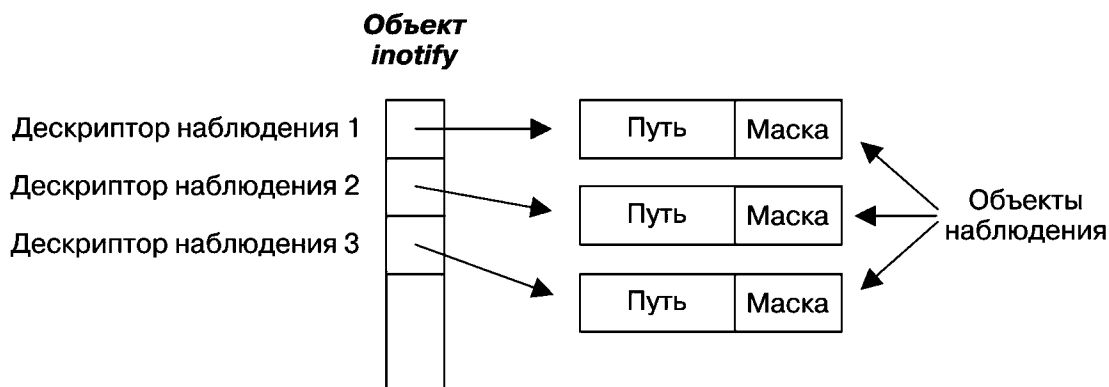
Рис. 19.1. Объект inotify и связанные структуры данных ядра
