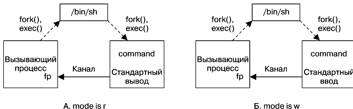
Рис. 44.4. Общая схема взаимодействия процессов и применения канала с помощью вызова popen()
