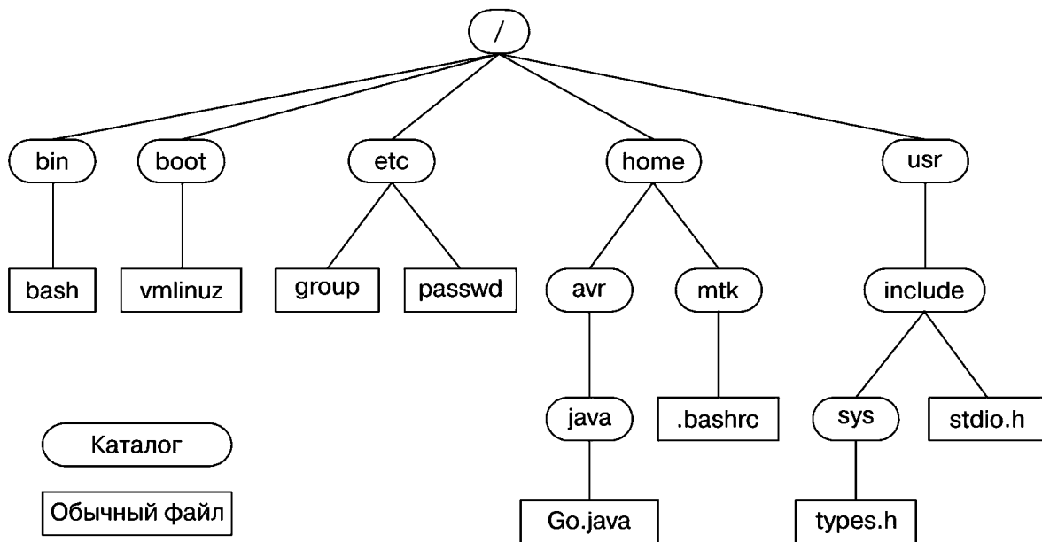
Рис. 2.1. Пример иерархии одного каталога Linux
