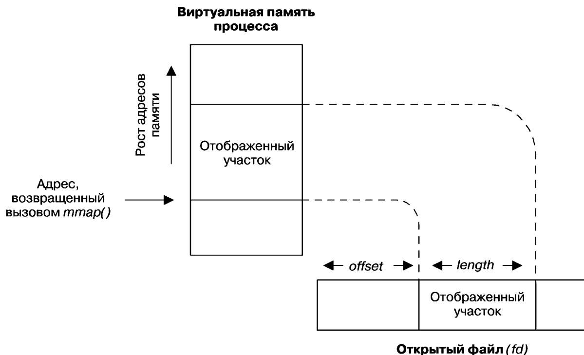
Рис. 45.1. Структура файла, отображенного в память
