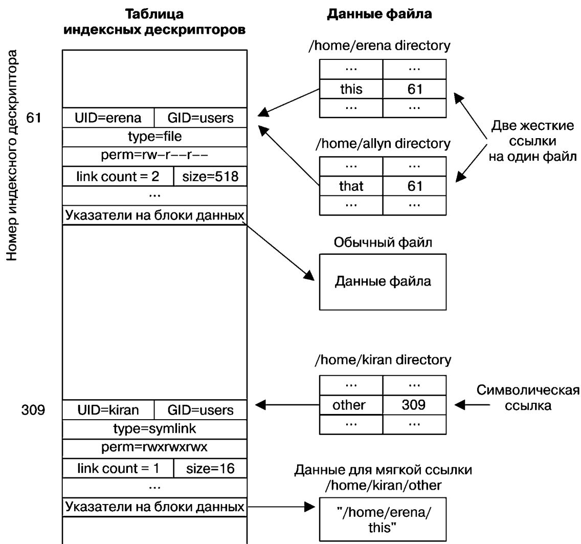
Рис. 18.2. Представление жестких и символических ссылок
