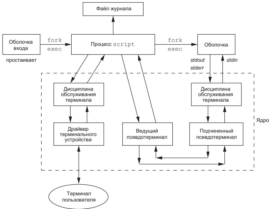
Рис. 19.5. Программа script
